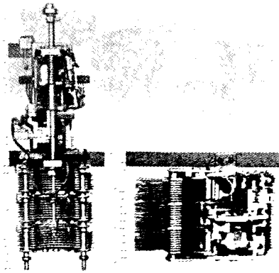
Sl. 14. STROWGEROV BIRAČ STARIJE I NOVIJE VRSTI u izvedbi Siemens-Halske
