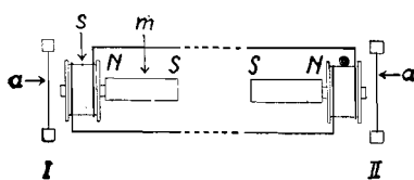
Sl. 2. BELLOV BRZOGLAS (načelno)
