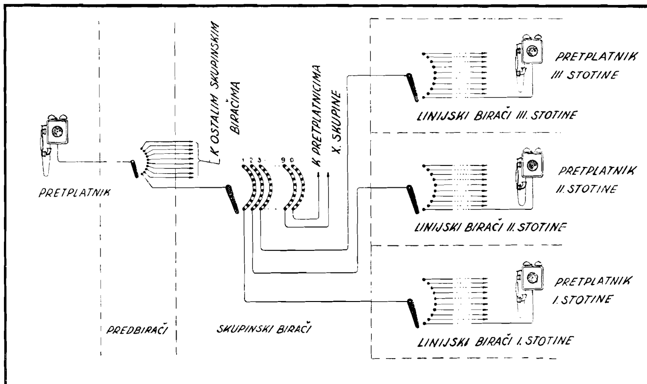
SL. 15. SHEMA SAMOSPOJNOG RADA SREDISNJICE ZA 1000 BROJEVA
