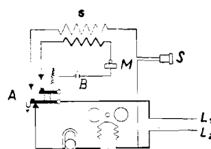
Sl. 7. SHEMA SPAJANJA INKUCTORSKOG APARATA. Slušalica položena na prekidač
