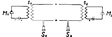
Sl. 5. SHEMA SPAJANJA BELLOVA BRZOGLASA S MIKROFONOM I INKUCIJSKIM SVITKOM
