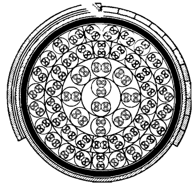
Sl. 19. PRESJEK BRZOGLASNOG KABLA S 51 CETVORKOM
