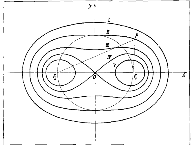
CASSINIJEVE KRIVULJE
