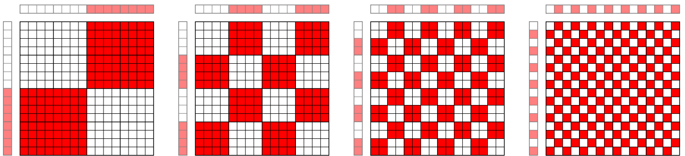
File:22^4; Cayley table; binary.svg
