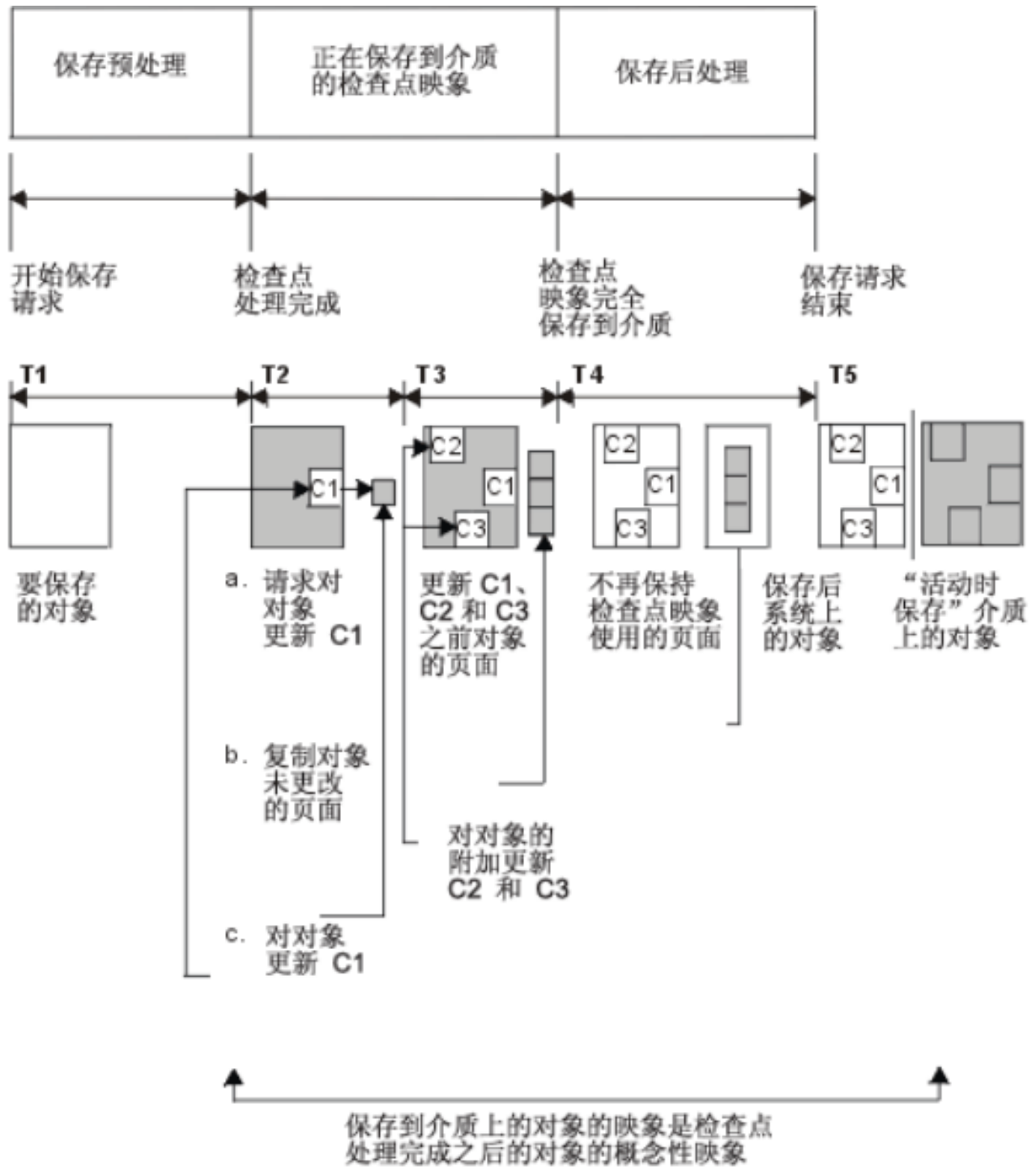
图 10. 检查点处理完成之后对象更新的服务器管理
