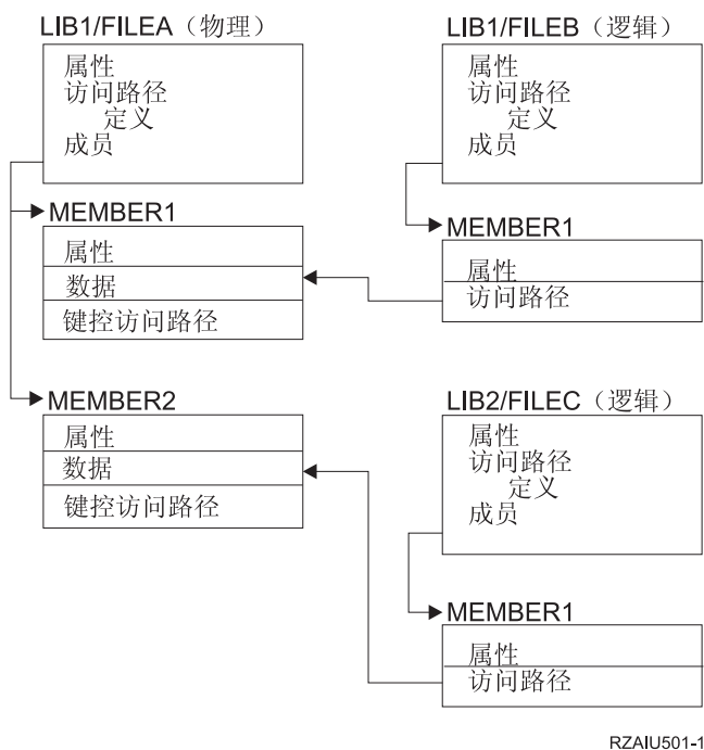
图 5. 保存访问路径
