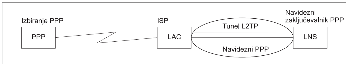
Slika 8. Klicni pobudnik PPP ali navidezni zaključevalnik PPP
