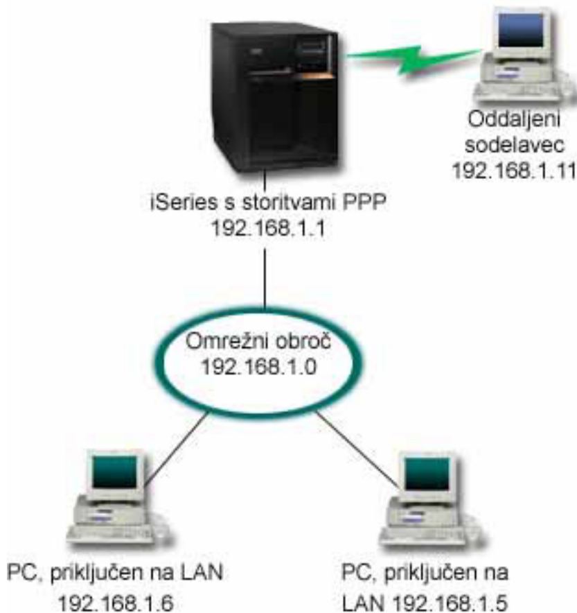
Slika 2. Povezovanje oddaljenih odjemalcev s strežnikom iSeries
