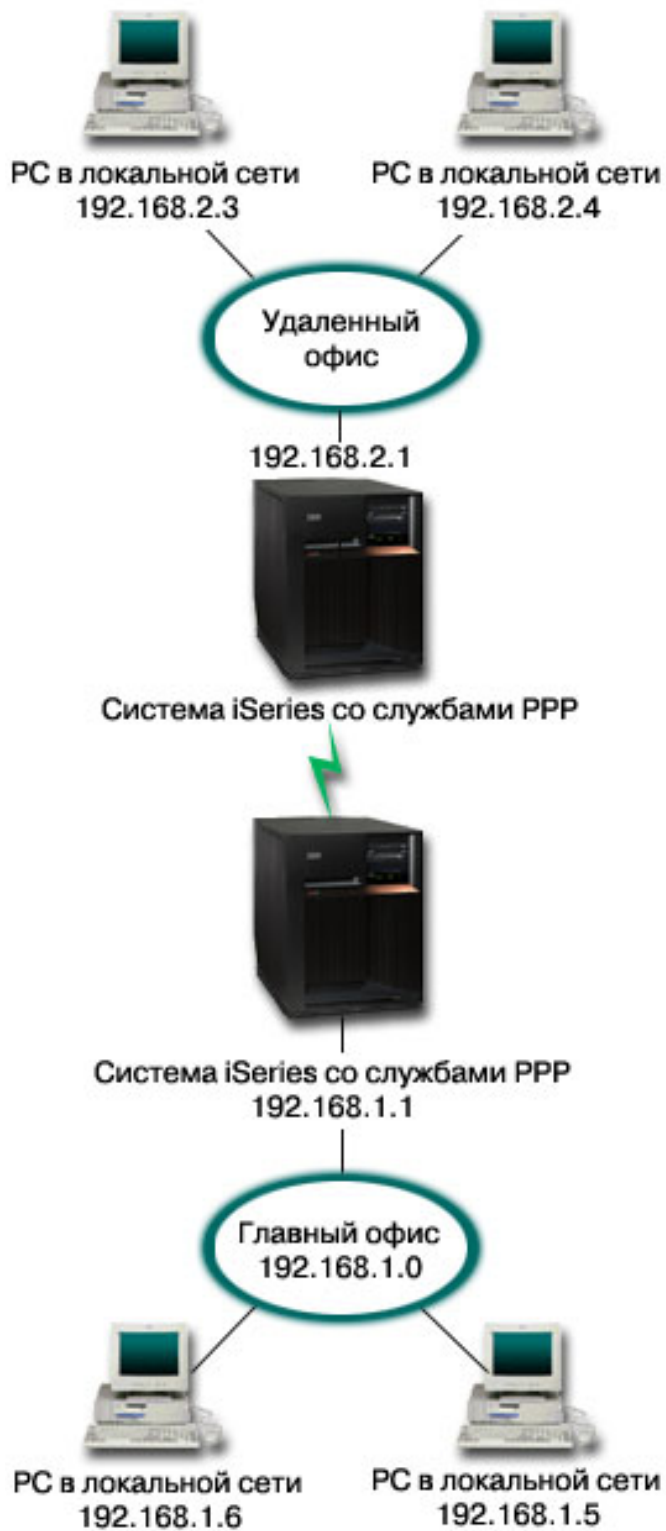
Рисунок 4. Подключение сети филиала компании к основной сети с помощью модема
