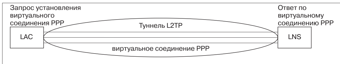
Рисунок 7. Виртуальный вызов PPP или виртуальный ответ PPP
