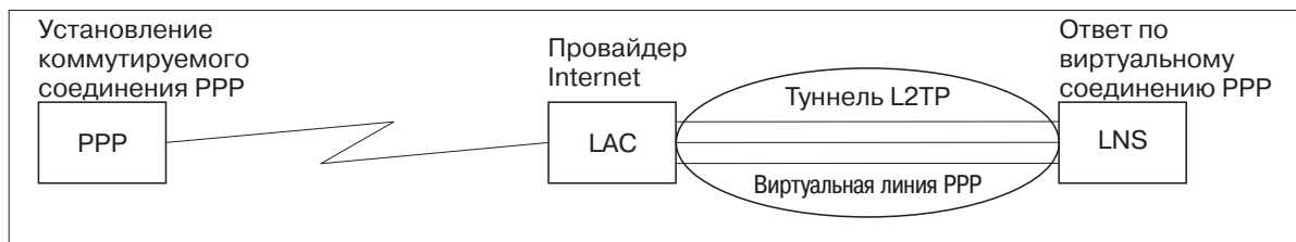
Рисунок 8. Набор номера PPP или виртуальный ответ PPP Virtual Terminator
