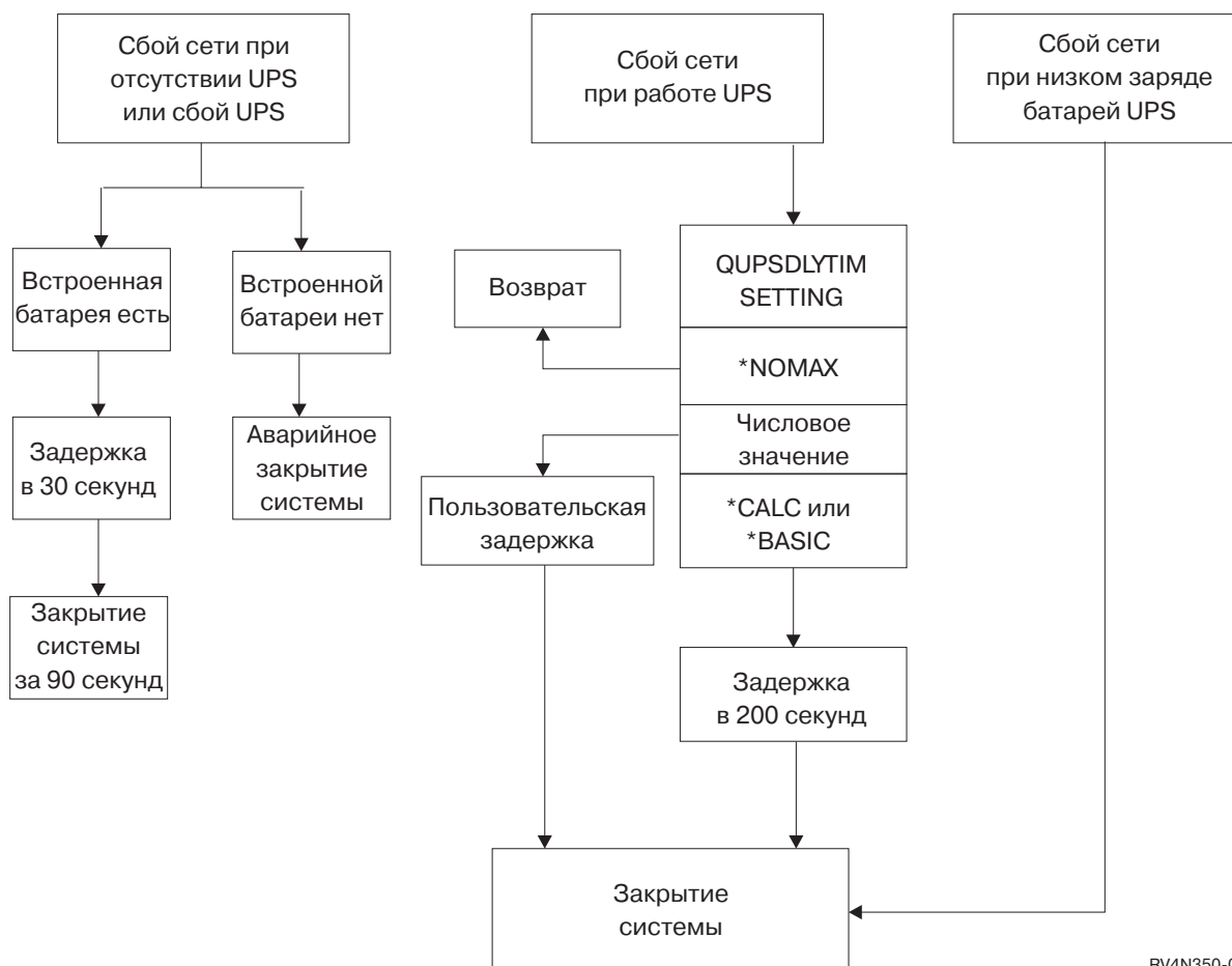
Рисунок 2. Значения QUPSDLYTIM и соответствующие действия
