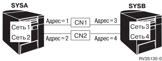
Рисунок 3. Правильная настройка, использующая две сети соединения и две линии связи локальной сети
