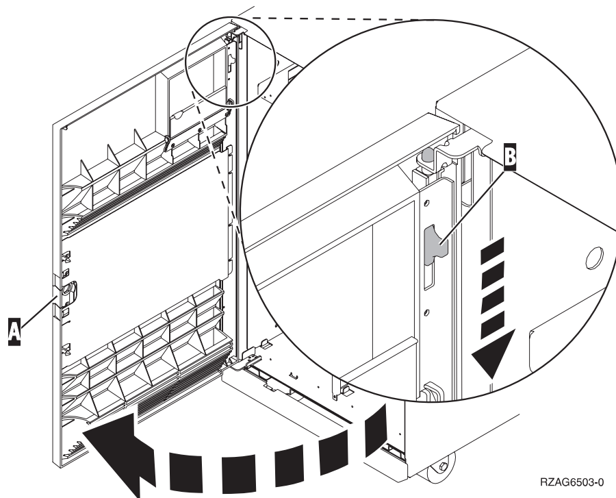
Figuur 1. Het voorpaneel openen (5074, 5094, 5095, 8093, 830, 840, 870, 890)
