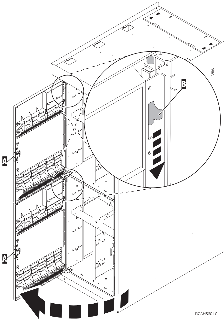
Figuur 4. Het voorpaneel openen (5079).
