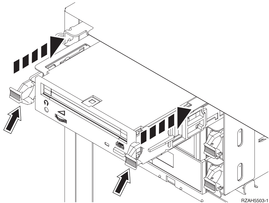
Figuur 6. Het CD-ROM- of bandstation installeren.
