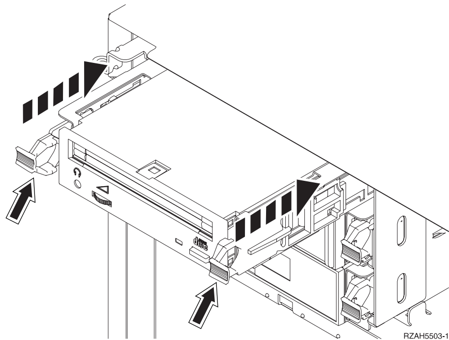
Figuur 5. Het CD-ROM- of bandstation installeren.
