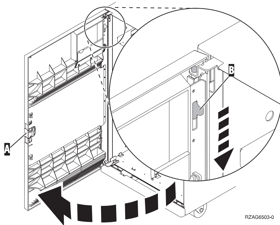
Figuur 3. Het voorpaneel openen (5074, 5094, 5095, 8093, 830, 840, 870, 890)
