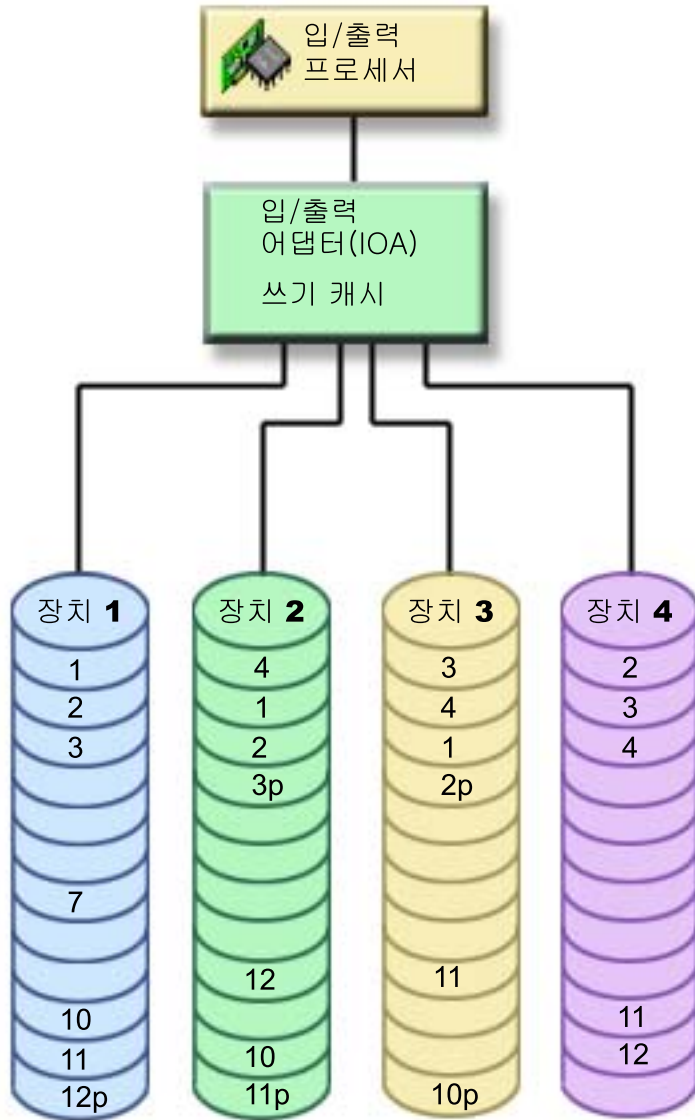
그림 2. 장치 패리티 보호 VSR2 이후 IOA를 사용하여 패리티 자료를 분산시키는 방법의 예
