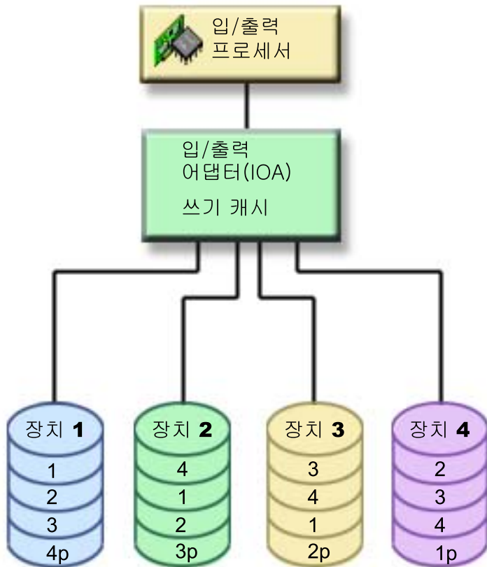
| 그림 1. 장치 패리티 보호 V5R2 이전 IOA를 사용하여 패리티 자료를 분산시키는 방법의 예 |
