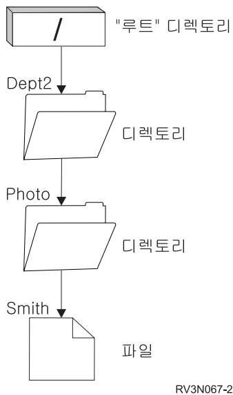
그림 6. 경로명의 구성요소
