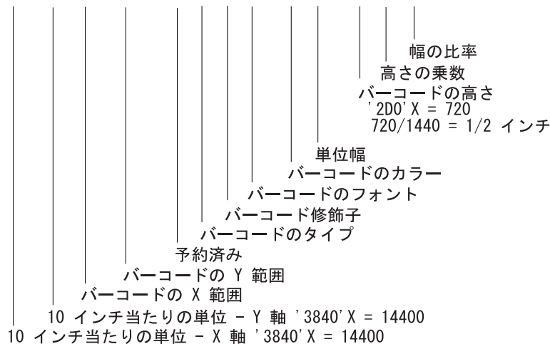
図 4. CVTDTA を使用するバーコード・コマンドのコマンド形式 (1/2)
