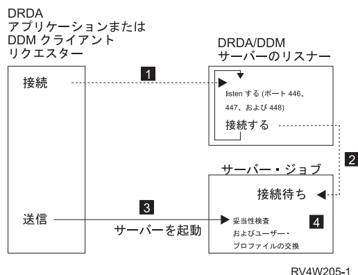
図 14. DRDA/DDM TCP/IP サーバー
