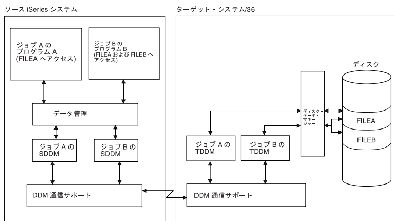
図 11. 複数のプログラムおよびファイル要求の処理例
