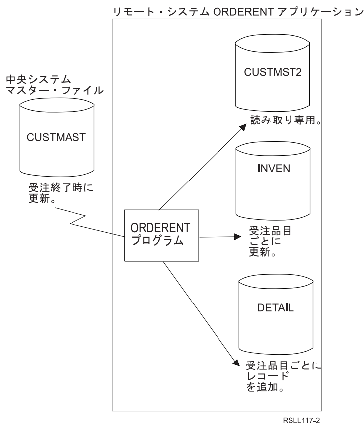
図 19. リモート ORDERENT プログラムが使用するファイル
