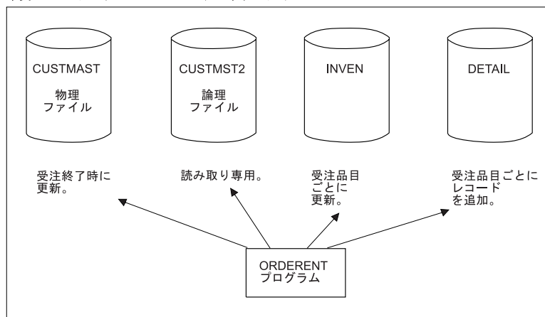
図 18. 中央サーバーの ORDERENT プログラムが使用するファイル
