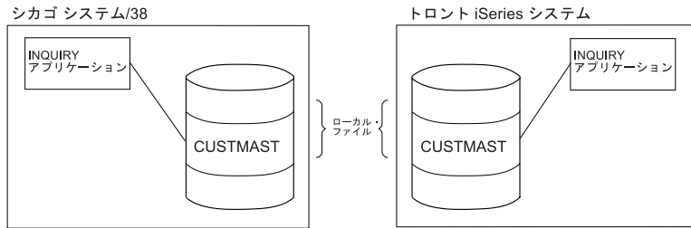
図 16. ローカル照会を行う 2 つの非 DDM サーバー
