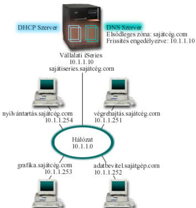
Ábra 3. DNS és DHCP ugyanazon az iSeries szerveren
