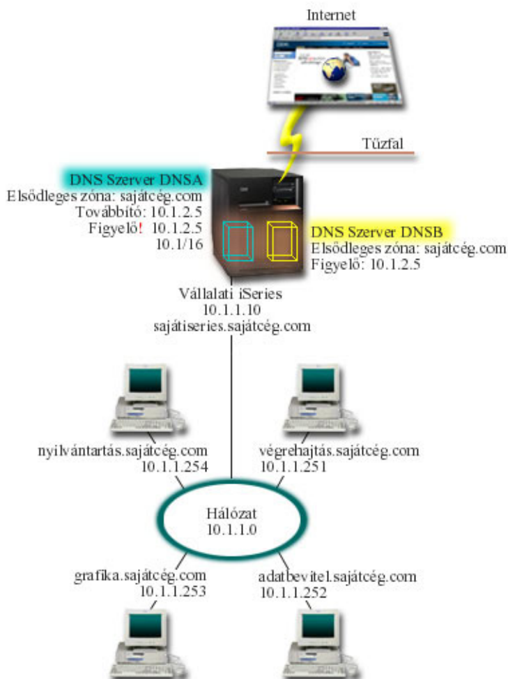
Ábra 4. DNS felosztása tűzfalon keresztül
