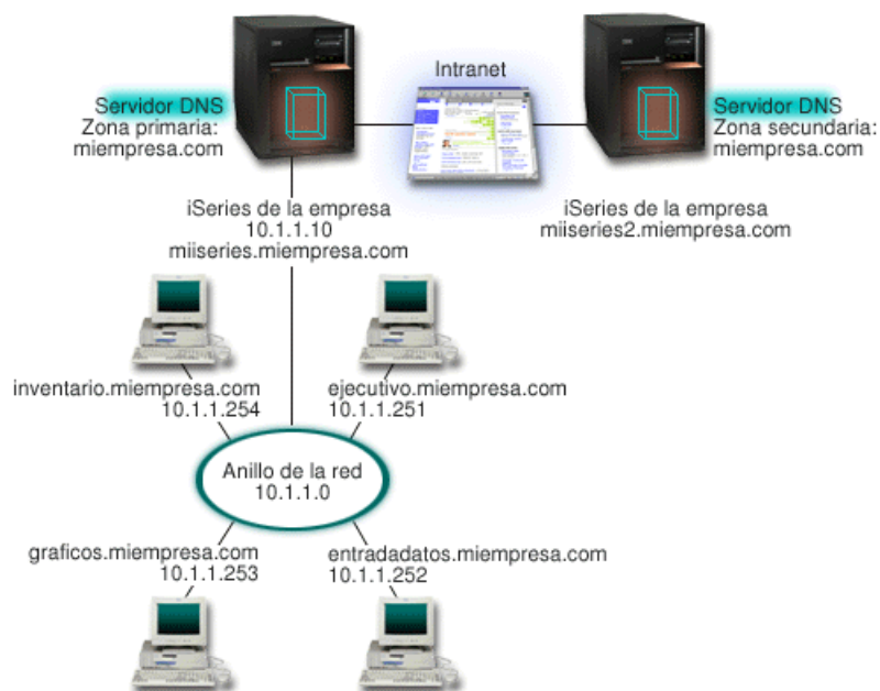
Figura 1. Un único servidor DNS para una intranet.
