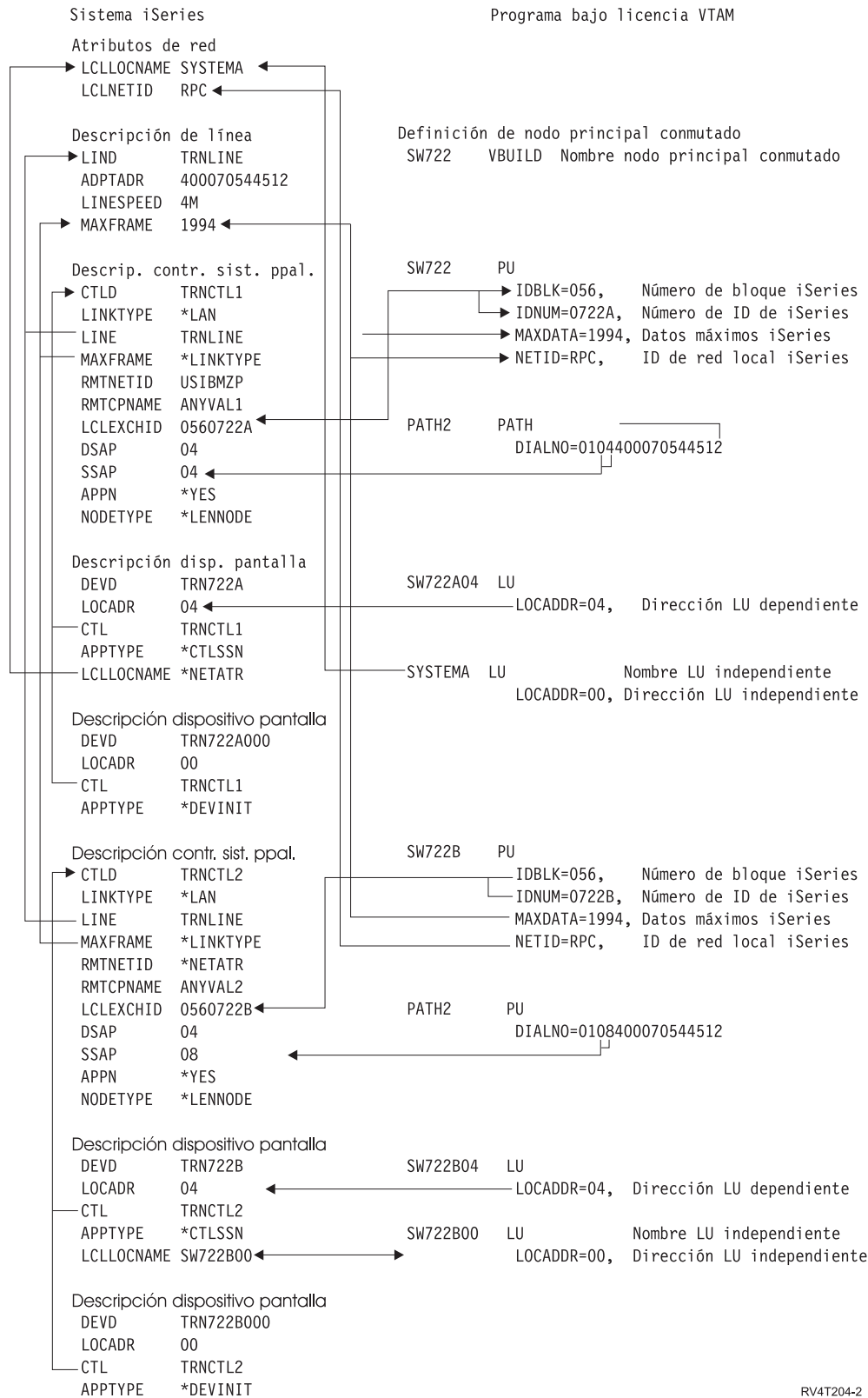
Ejemplo 3: soporte del sistema iSeries para el DLUR con el sistema principal.
