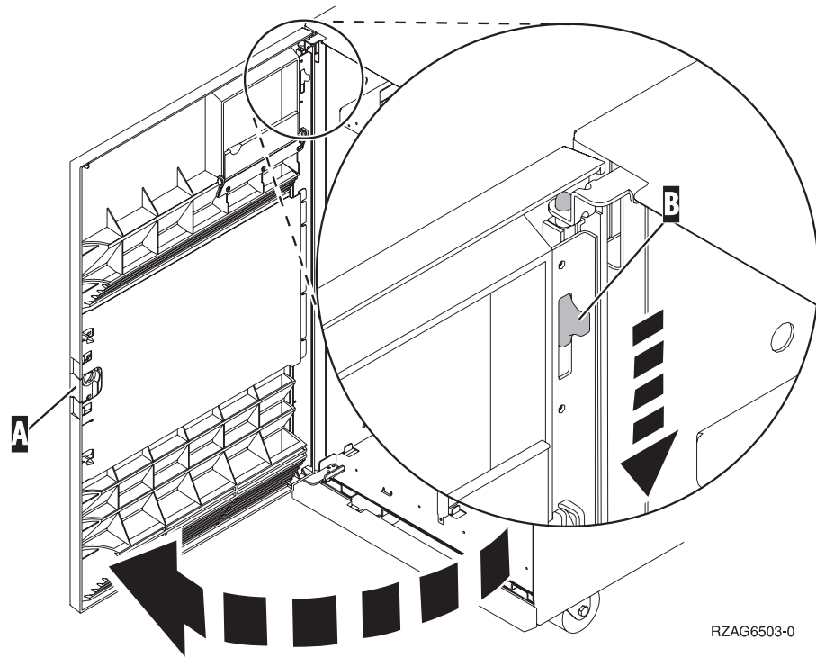
Figura 1. Apertura de la puerta de la cubierta frontal (5074, 5094, 5095, 8093, 830, 840, 870, 890)
