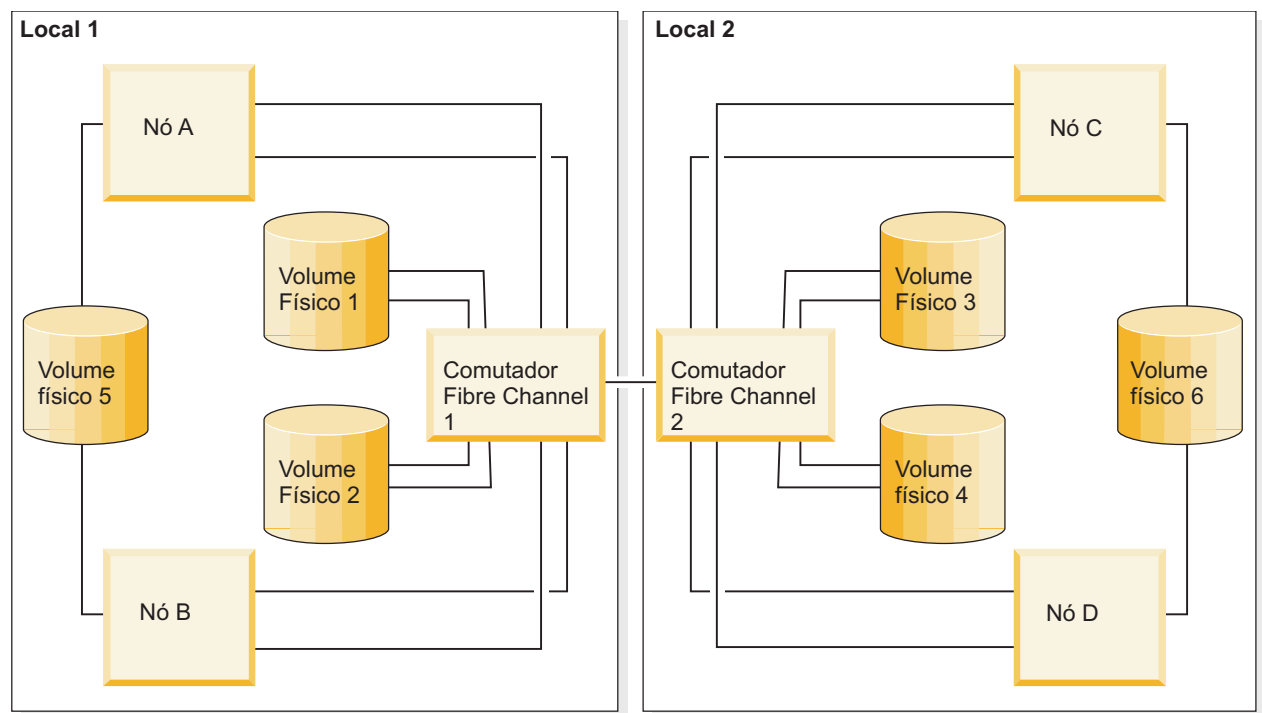
Figura 8. Configuração de espelhamento de site de divisão do LVM usando uma SAN
