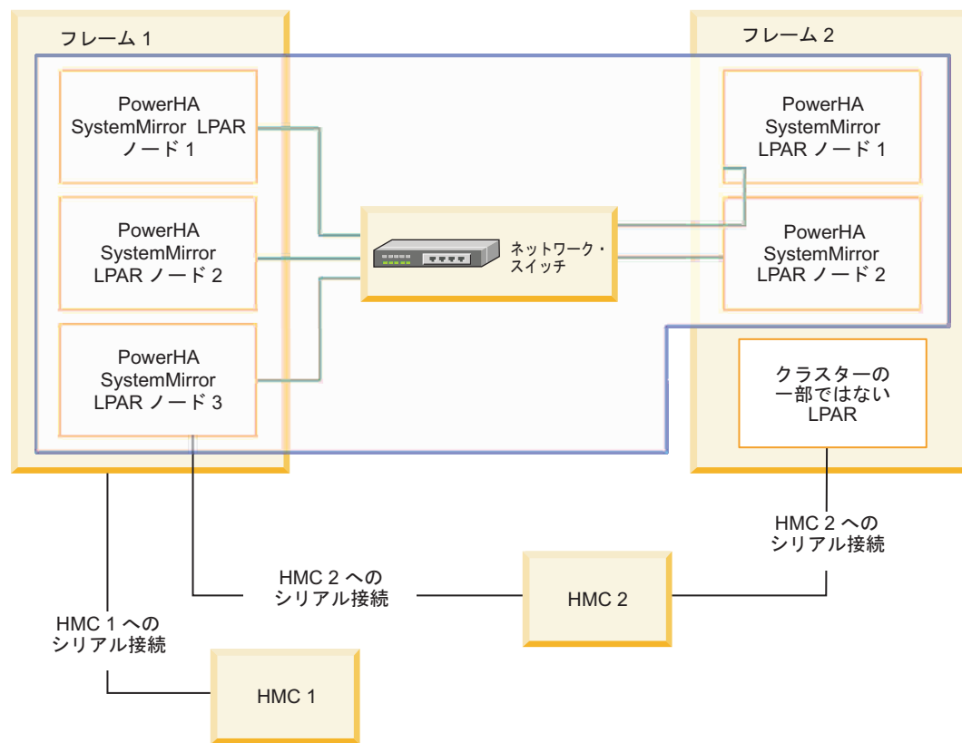
図 11. LPAR を使用した PowerHA SystemMirror クラスター構成
