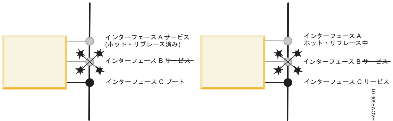
図 7. インターフェース A のホット・リブレース中にインターフェース B で障害が発生した場合のインターフェース C の動作
