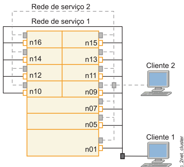
Figura 3. Configuração de rede dupla e NIC dupla
