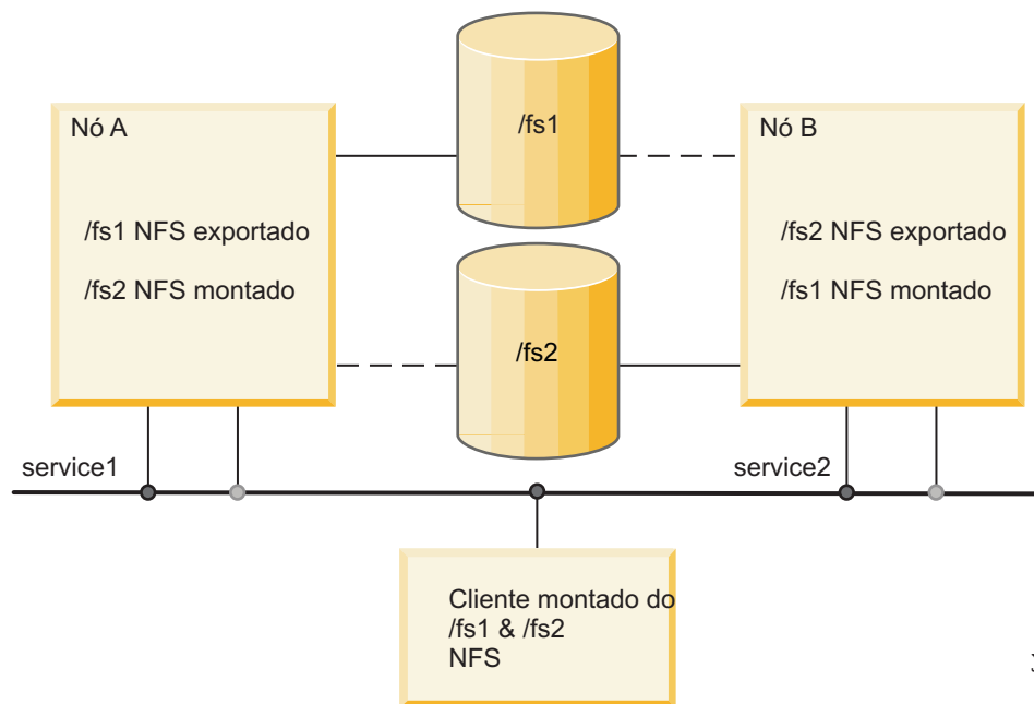
Figura 10. Montagem cruzada do NFS de dois nós
