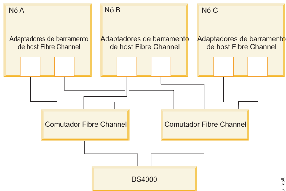
Figura 4. Ambiente do DS4000 Storage Server
