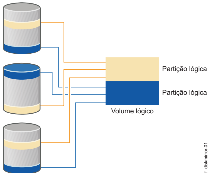
Figura 7. Volume lógico de duas partições lógicas com três cópias espelhadas
