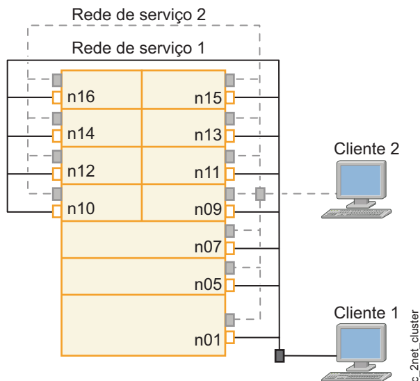
Figura 2. Configuração de rede dupla
