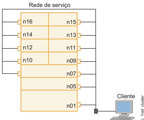
Figura 1. Configuração de rede única e NIC único
