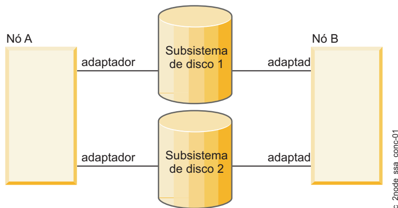
Figura 9. Configuração de acesso simultâneo do subsistema de disco da IBM
