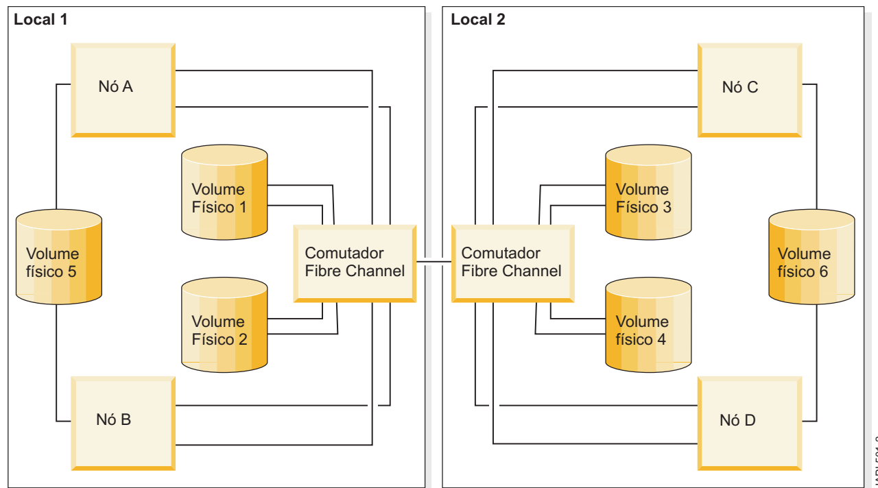
Figura 8. Configuração de espelhamento de site de divisão do LVM usando uma SAN
