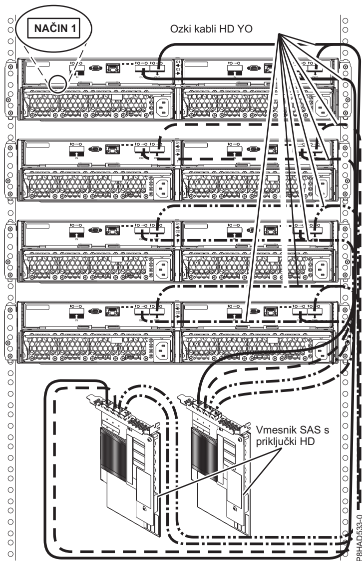
Slika 88. Povezava štirih ohišij 5887 v načinu 1 z dvema vmesnikoma PCIe3 SAS z ozkimi spojniki HD.
