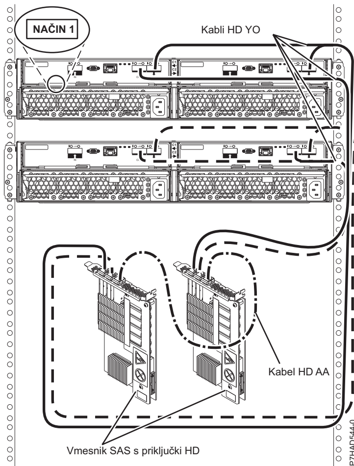
Slika 82. Povezava dveh ohišij 5887 v načinu 1 s spojniki HD z dvema vmesnikoma SAS PCIe2
