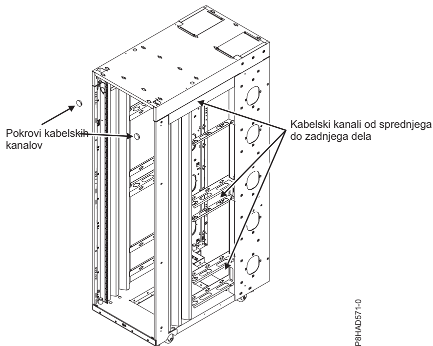
Slika 36. Povezovanje kablov znotraj omare
