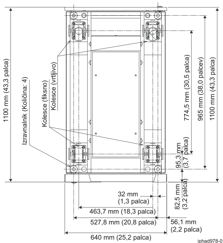
Slika 23. Lokacije koles in izravnalnikov
