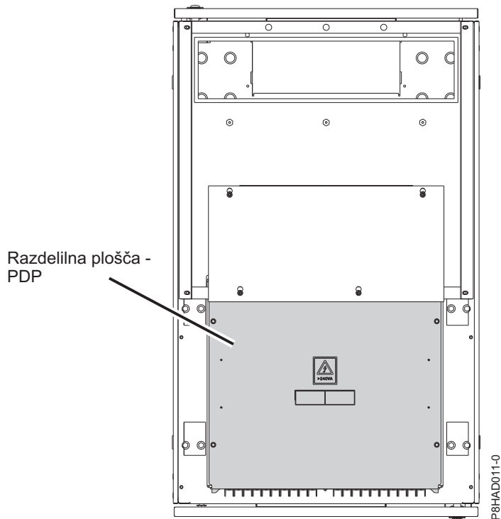
Slika 22. Koda možnosti EPB8 - razdelilna plošča (pogled od zgoraj navzdol)
