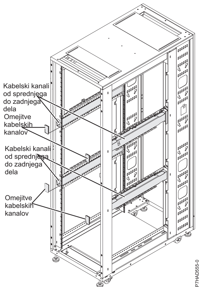
Slika 27. Povezovanje kablov znotraj omare
