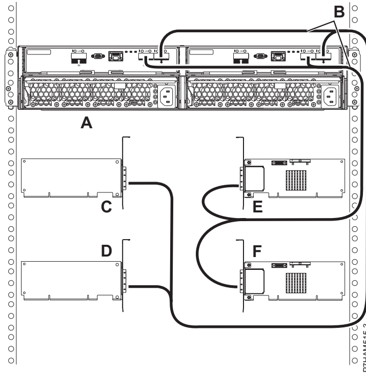
Slika 78. Povezava ohišja 5887 v načinu 4 s kabli X s štirimi enojnimi vmesniki SAS
