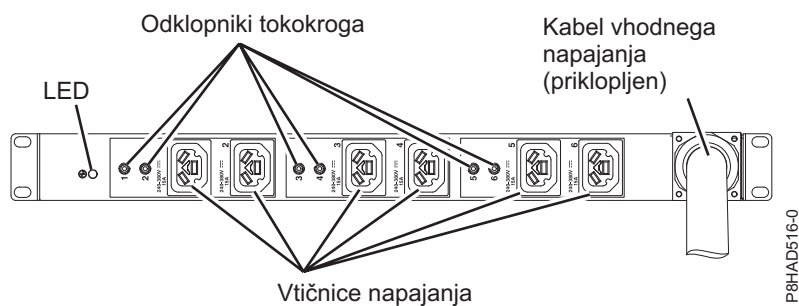
Slika 49. Napajalna distribucijska enota HVDC
