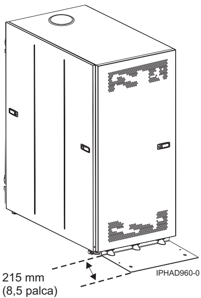
Slika 18. Model 0555 in 7014-S25 s stabilizacijsko nogo
