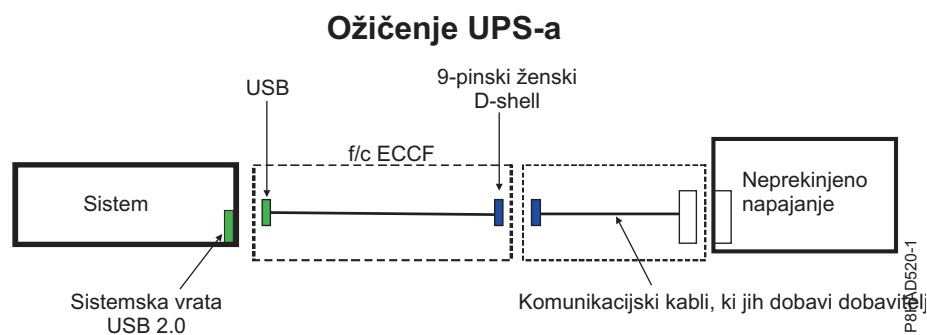
Slika 45. Ožičenje UPS-a za 5148-21L, 5148-22L, 8247-21L, 8247-21L, 8247-22L, 8247-42L, 8284-22A, 8286-41A in 8286-42A
