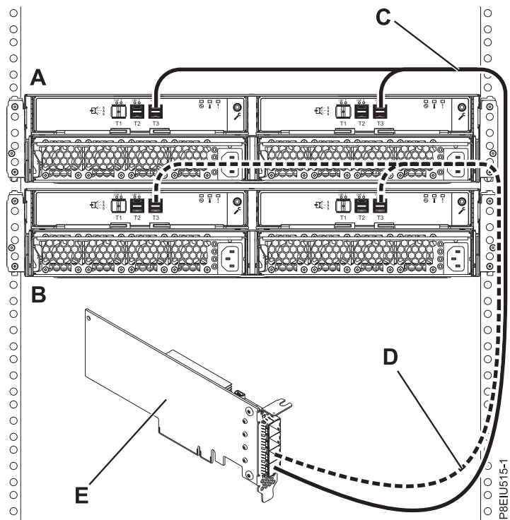
Slika 92. Povezava v načinu 1 dveh ohišij pomnilnika ESLL ali ESLS s kabli YO12 z enojnim vmesnikom SAS
