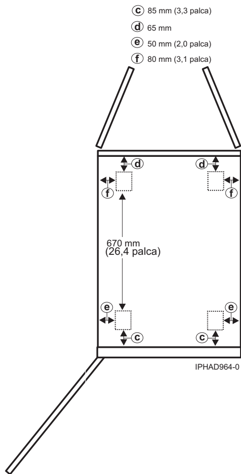
Slika 20. Lokacije kolesc za model 0555 in 7014-S25
