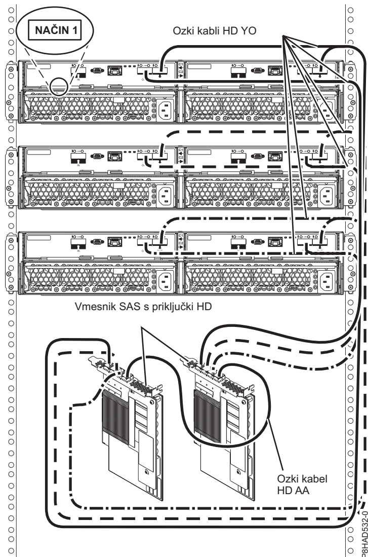
Slika 87. Povezava treh ohišij 5887 v načinu 1 z dvema vmesnikoma PCIe3 SAS z ozkimi spojniki HD.
