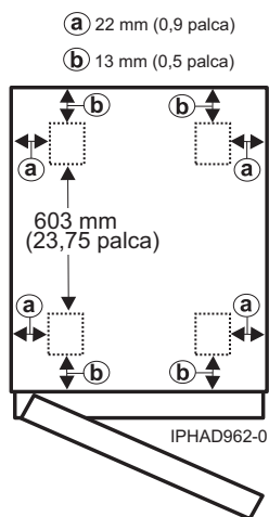
Slika 17. Lokacije koles za model 0554 in 7014-S11
