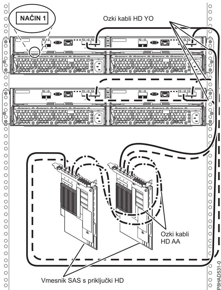
Slika 86. Povezava dveh ohišij 5887 v načinu 1 z dvema vmesnikoma PCIe3 SAS z ozkimi spojniki HD.
