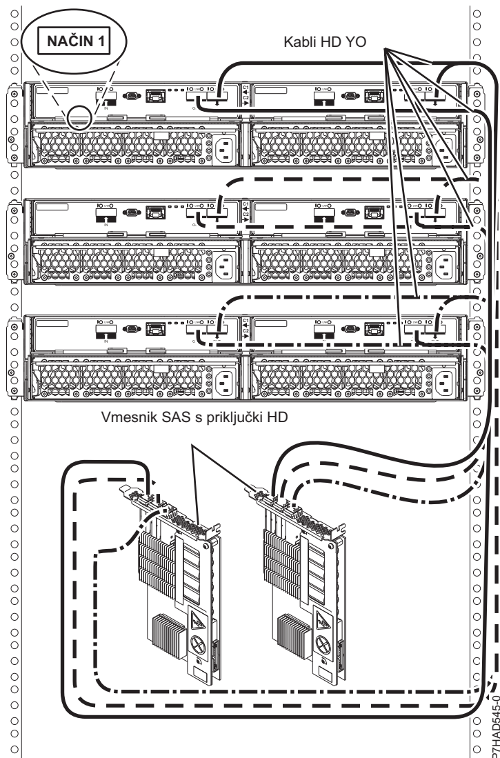
Slika 83. Povezava treh ohišij 5887 v načinu 1 z dvema vmesnikoma SAS PCIe2 s spojniki HD
