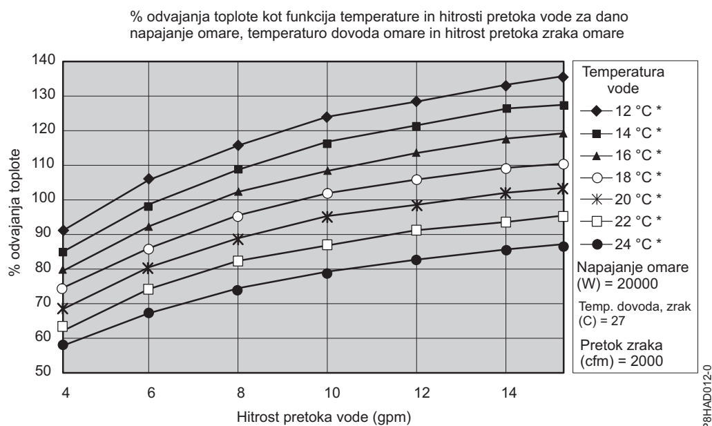
Slika 32. Običajna zmogljivost toplotnega izmenjevalnika z 20-kW toplotno obremenitvijo
