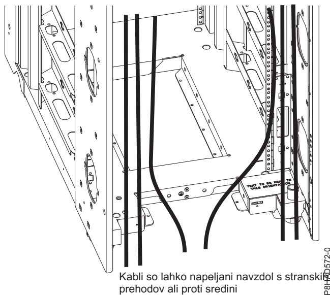
Slika 37. Povezovanje kablov pod tlemi
