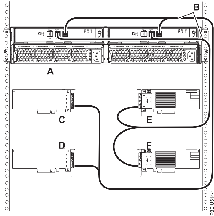
Slika 97. Povezava v načinu 4 enega ohišja Ohišje za pomnilnik ESSL ali ESLS s kabli X12 s štirimi neodvisnimi vmesniki SAS
