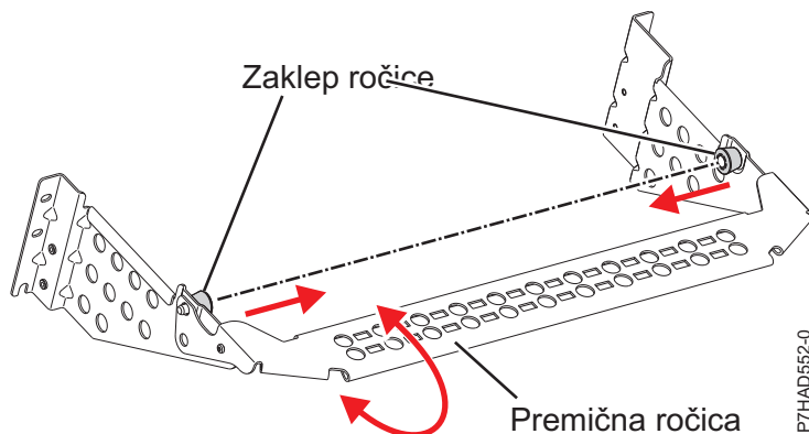
Slika 52. Nosilec za napeljavo kablov
