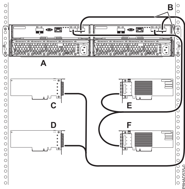
Slika 90. Povezava ohišja 5887 v načinu 4 s kablji X s štirimi enojnimi vmesniki SAS PCIe3 z ozkimi spojniki HD.
