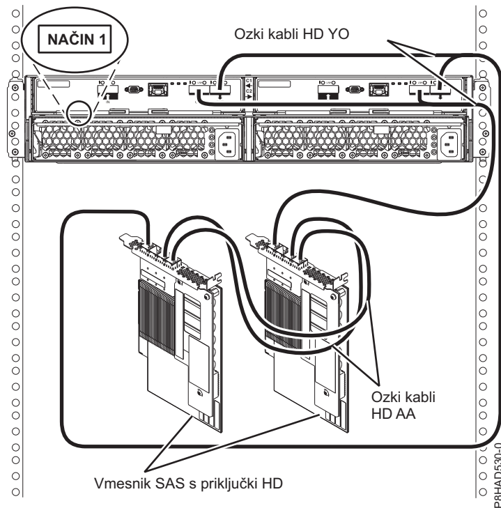
Slika 85. Povezava ohišja 5887 v načinu 1 z dvema vmesnikoma PCIe3 SAS z ozkimi spojniki HD.
