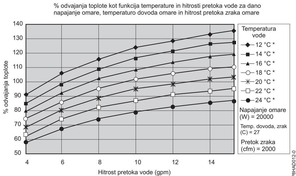
Slika 53. Običajna zmogljivost toplotnega izmenjevalnika z 20-kW toplotno obremenitvijo
