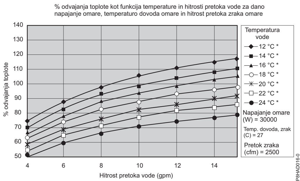
Slika 54. Običajna zmogljivost toplotnega izmenjevalnika s 30-kW toplotno obremenitvijo
