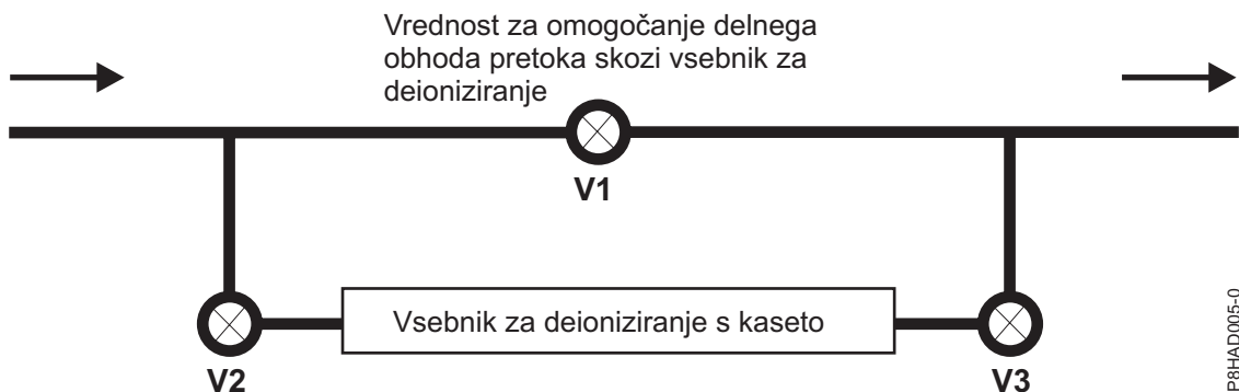
Slika 88. Deioniziranje vode s kasetami za deioniziranje, ki so nameščene v hladilni zanki
