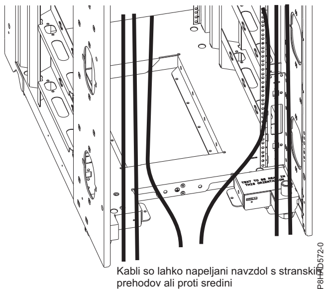
Slika 50. Povezovanje kablov pod tlemi
