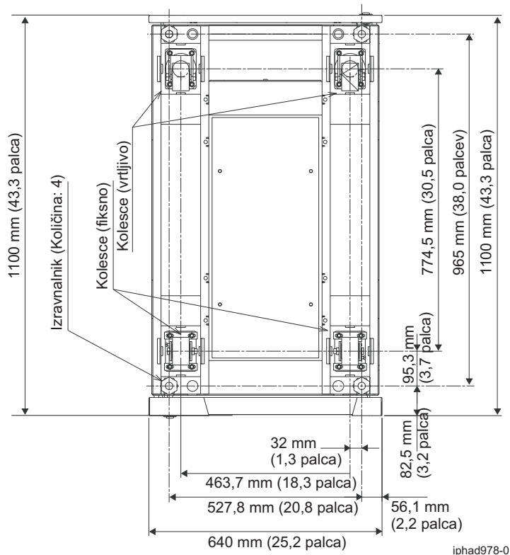
Slika 28. Lokacije koles in izravnalnikov
