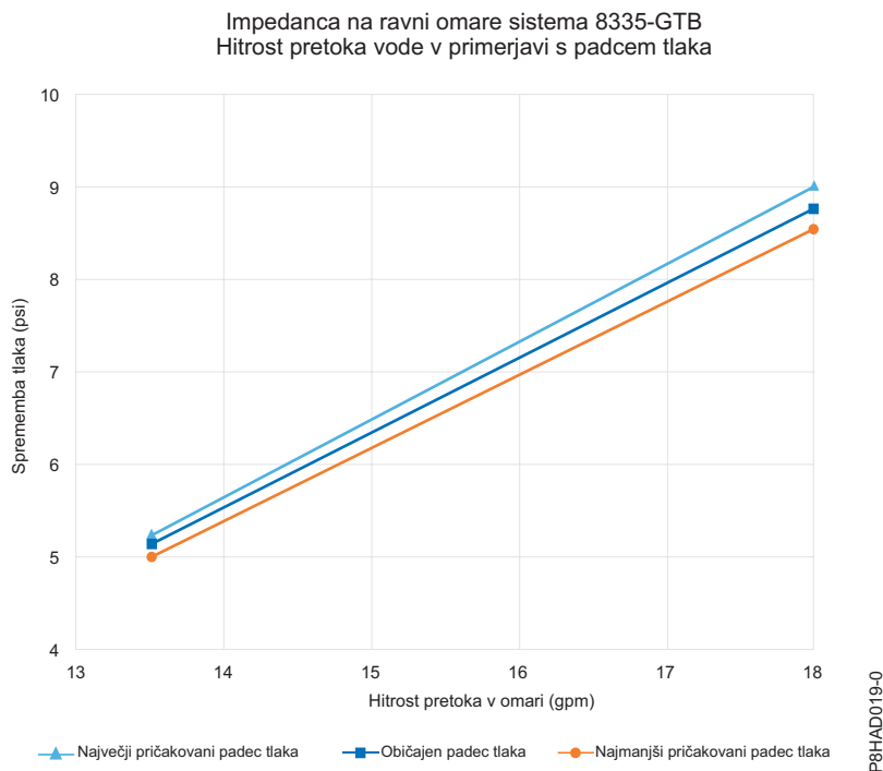
Slika 3. Hitrost pretoka v primerjavi s padcem tlaka (standardne enote) - polna omara z 18 strežniki
