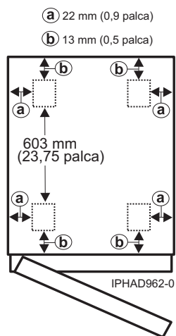
Slika 22. Lokacije kolesa za model 0554 in 7014-S11
