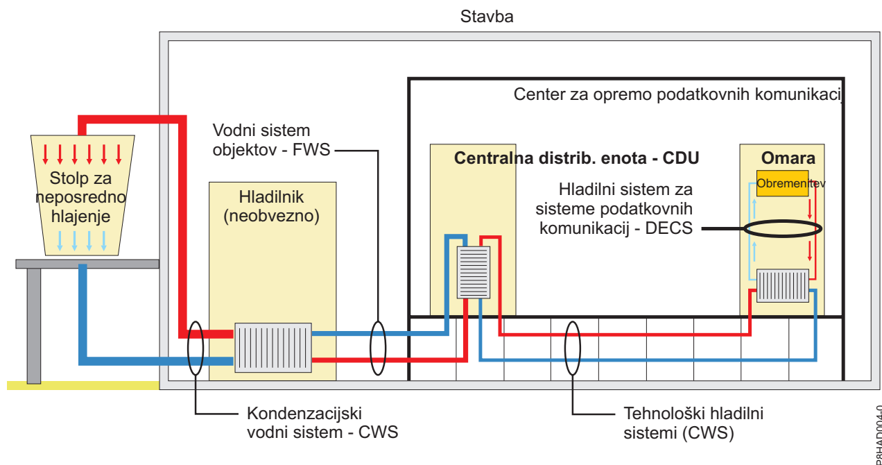
Slika 87. Primer tekočinskih hladilnih sistemov in zank v podatkovnem centru
