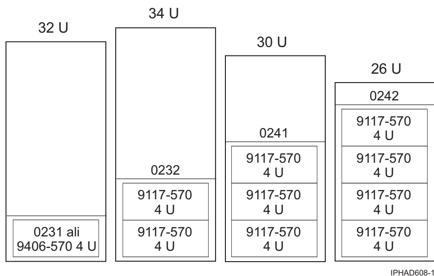
Slika 12. 570 v omari
