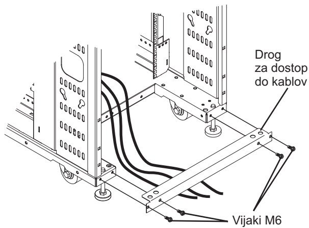
Slika 33. Drog za dostop do kablov
