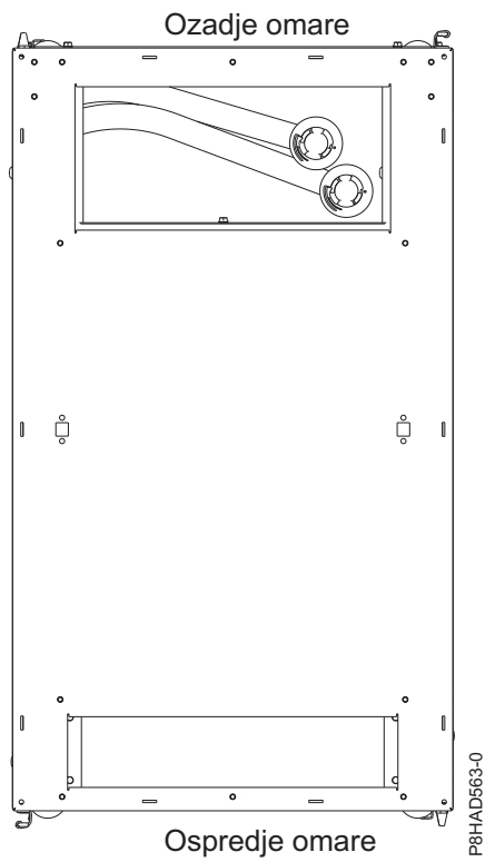
Slika 43. Mesta za izhod cevi na vrhu (gledano z zgornje strani)
