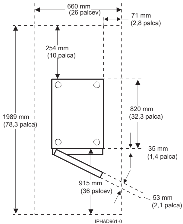
Slika 21. Prikaz načrta modela 0554 in 7014-S11
