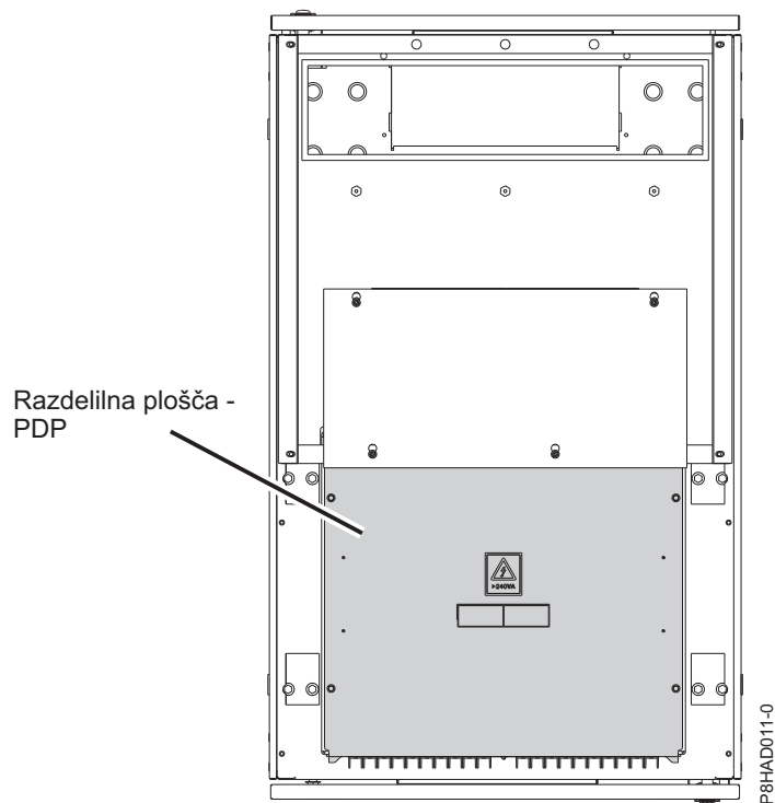
Slika 27. Koda možnosti EPB8 - razdelilna plošča (pogled od zgoraj navzdol)
