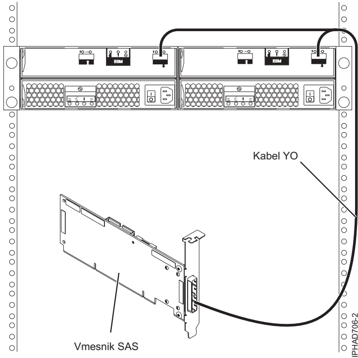
Slika 69. Vmesnik SAS s predalom za razširitev diskov
