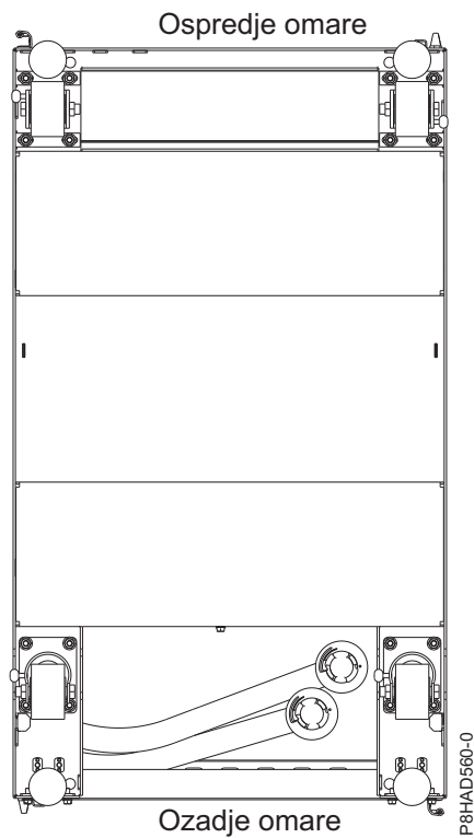
Slika 45. Mesta na izhod cevi na dnu (gledano od spodaj)
