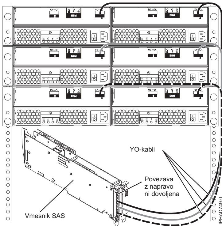
Slika 72. Trivratni vmesnik SAS s predali za razširitev diskov
