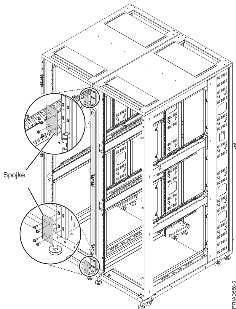
Slika 36. Spojke
