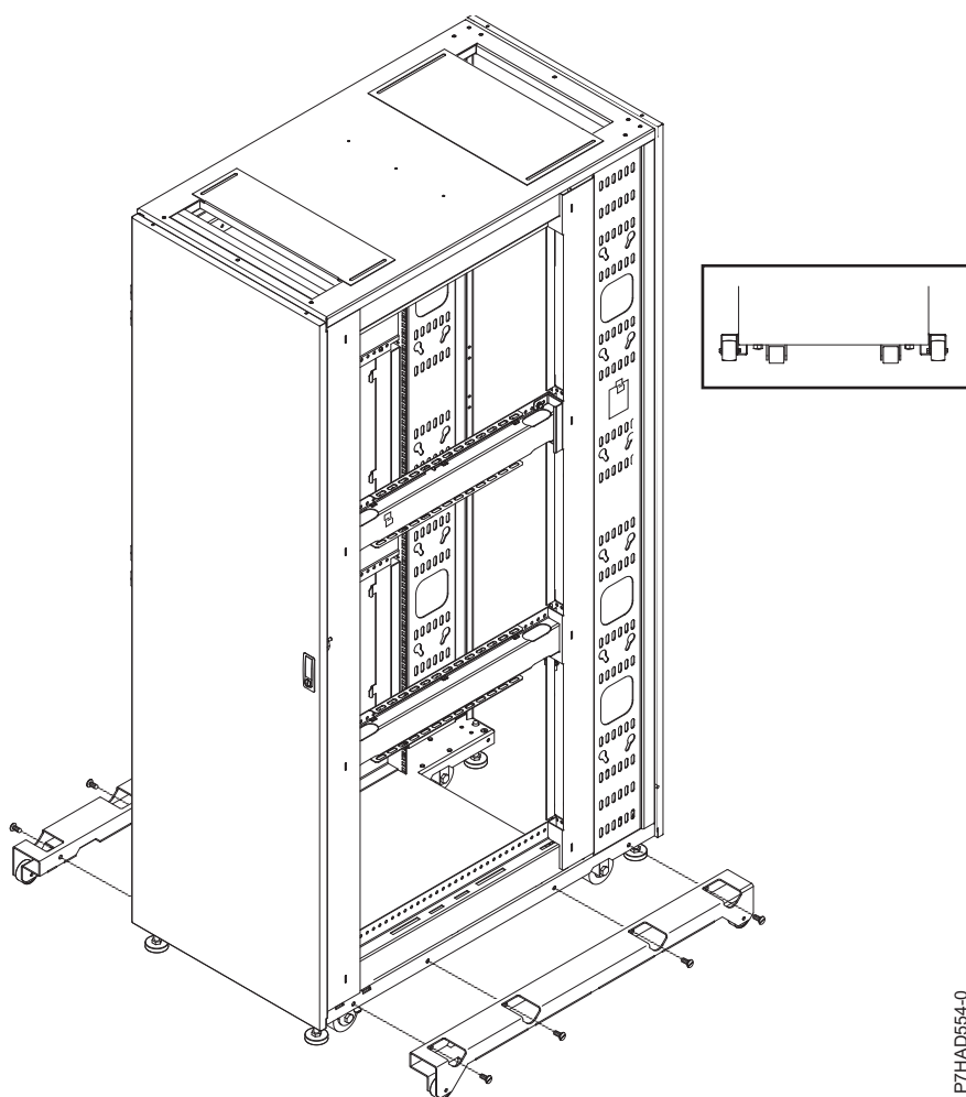
Slika 35. Lokacije preves
