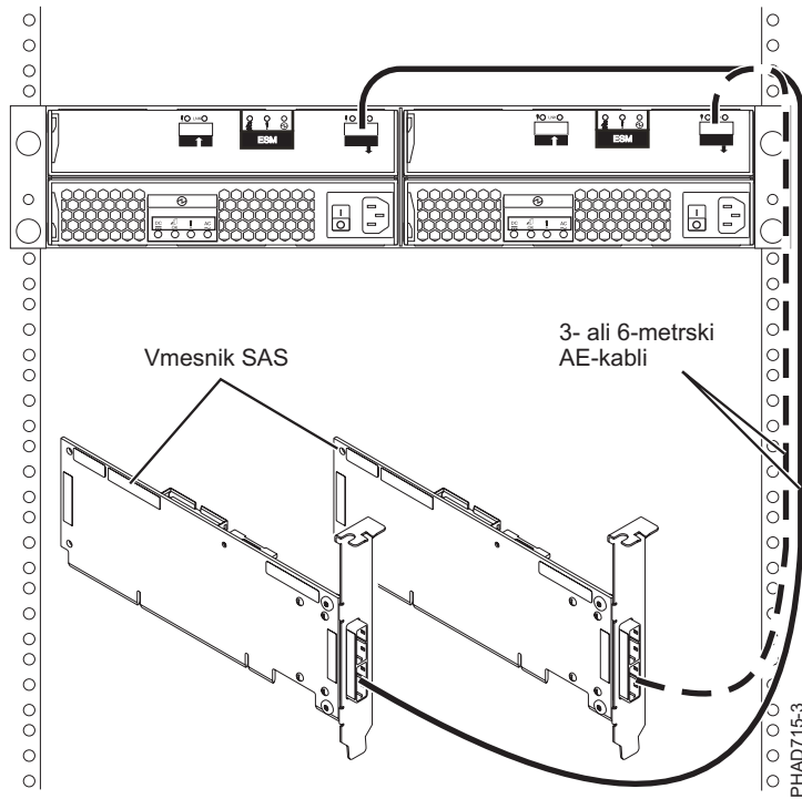
Slika 86. Dva vmesnika RAID SAS, povezana s predalom za razširitev diskov v konfiguraciji JBOD visoke razpoložljivosti z več iniciatorji
