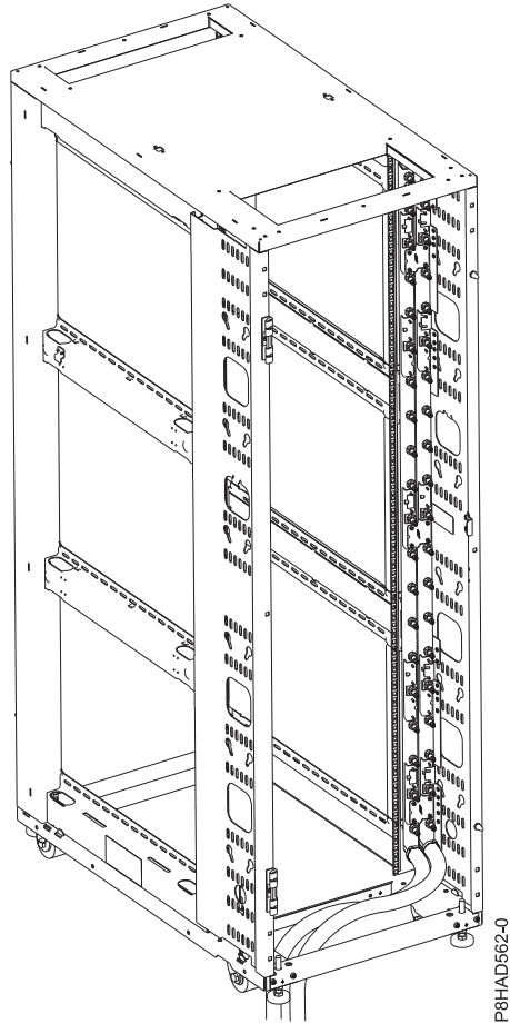
Slika 41. Omara in razdelilnik z izhodom za dovodno in odvodno cev na dnu omare
