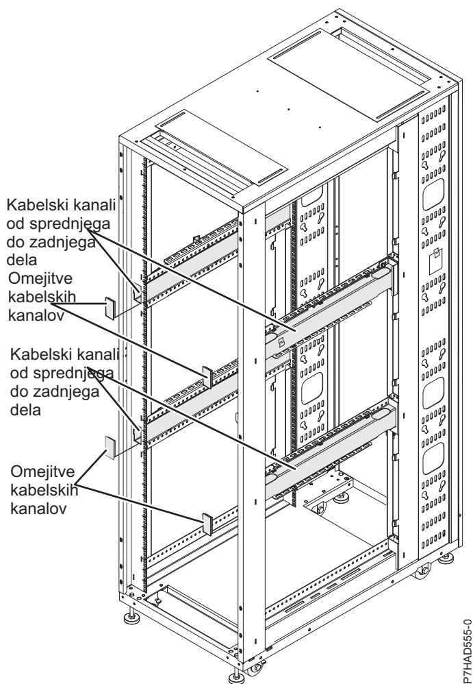
Slika 32. Povezovanje kablov znotraj omare
