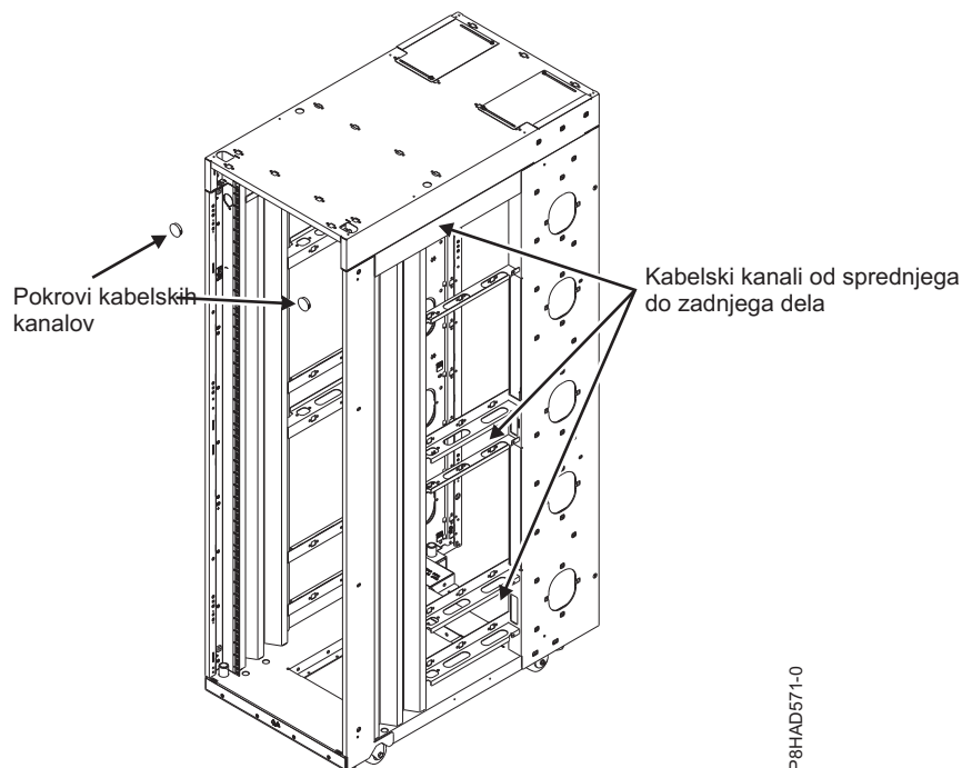
Slika 49. Povezovanje kablov znotraj omare
