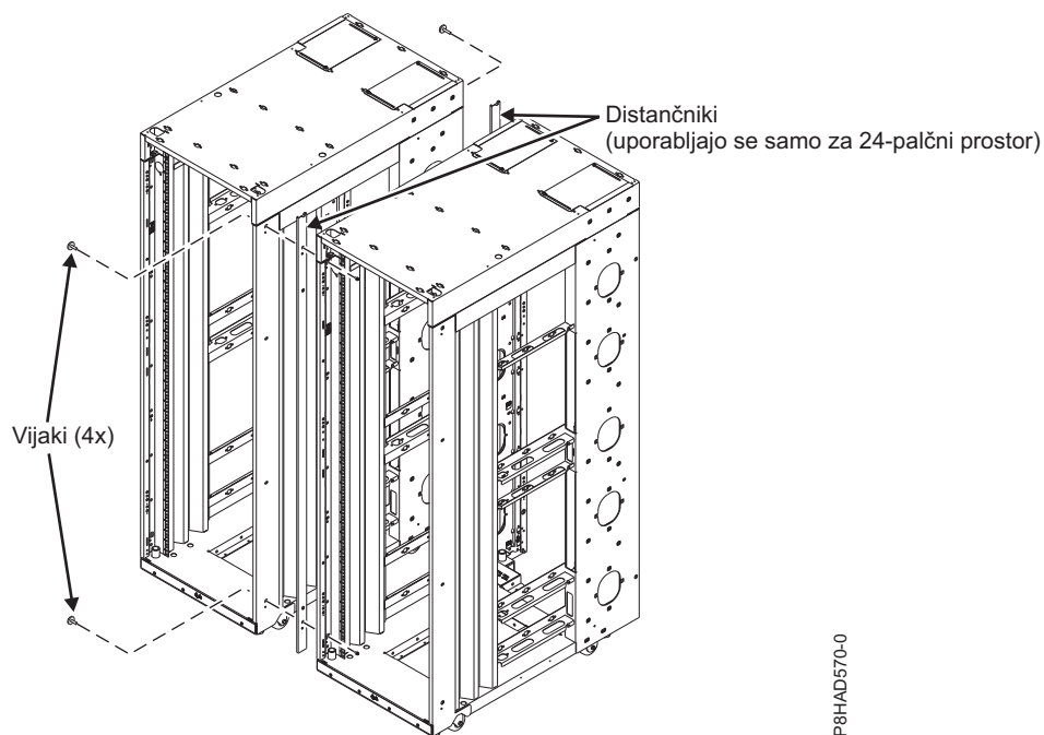
Slika 52. Povezovanje več omar
