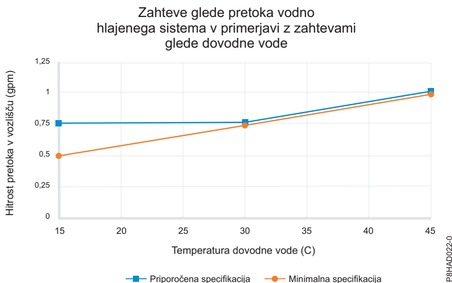
Slika 2. Zahteve glede pretoka za sistem z vodnim hlajenjem v primerjavi z zahtevami glede dovodne vode (standardne enote)
