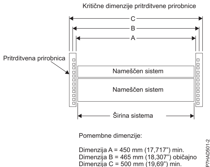
Slika 56. Kritične dimenzije pritrditvene prirobnice
