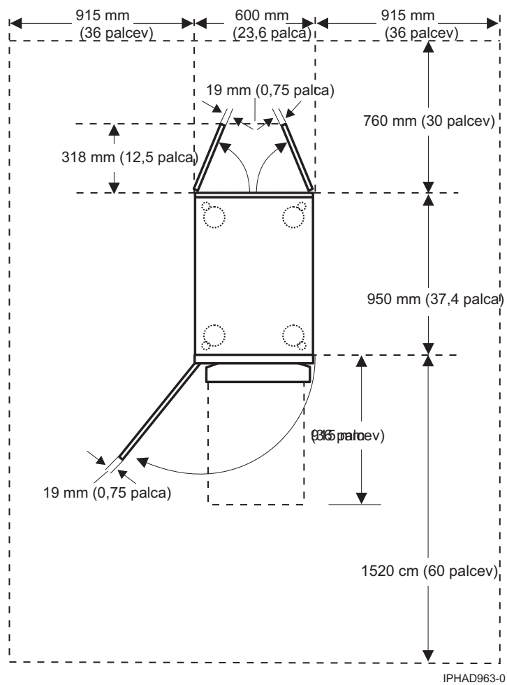
Slika 24. Prikaz načrta za model 0555 in 7014-S25
