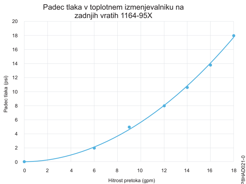
Slika 39. Padec tlaka (standardne enote)
