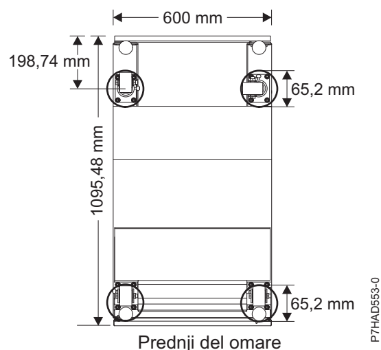
Slika 31. Lokacije kolesc
