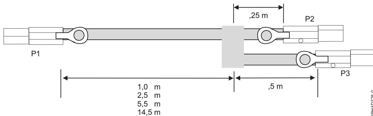
Slika 67. Dolžine kablov v zunanjem SAS YO-kabelskem kompletu
