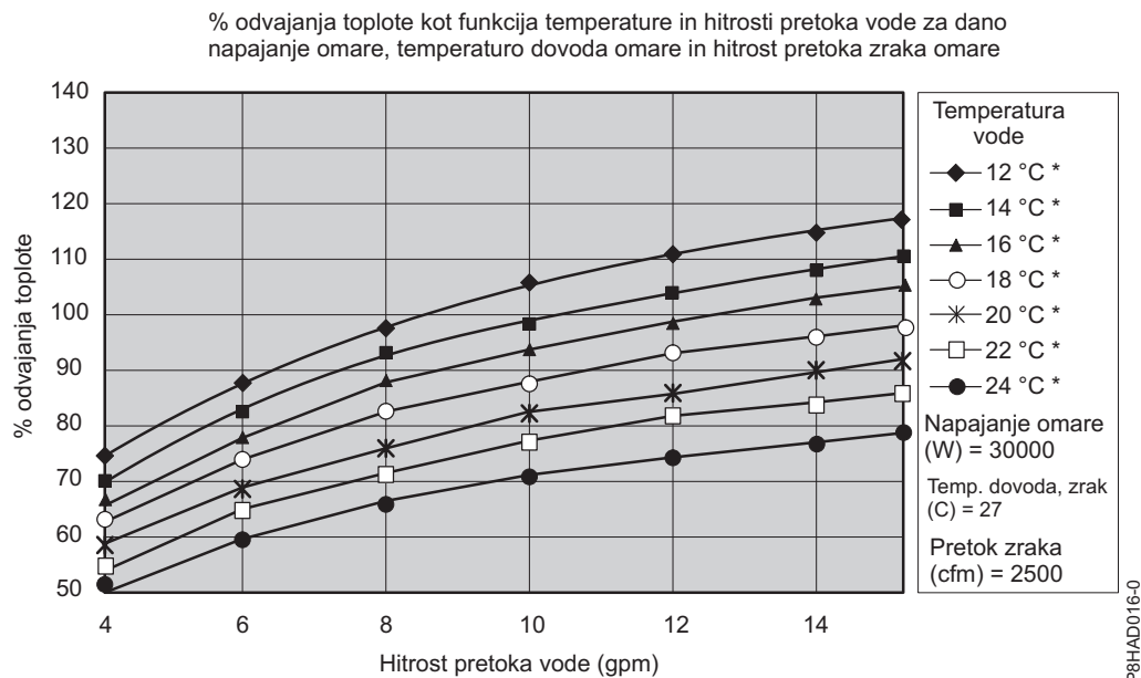
Slika 38. Običajna zmogljivost toplotnega izmenjevalnika s 30-kW toplotno obremenitvijo
