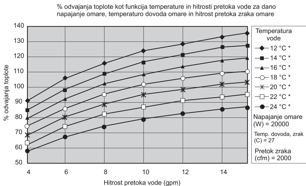
Slika 37. Običajna zmogljivost toplotnega izmenjevalnika z 20-kW toplotno obremenitvijo
