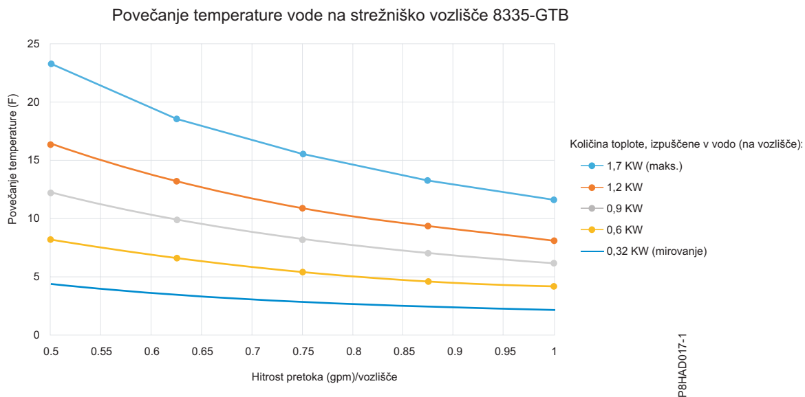
Slika 4. Hitrost pretoka vode v primerjavi s temperaturo dovodne vode - en strežnik (standardne enote)
