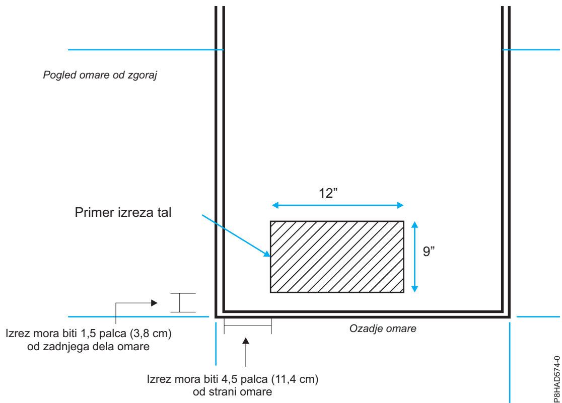
Slika 48. Izrez tal
