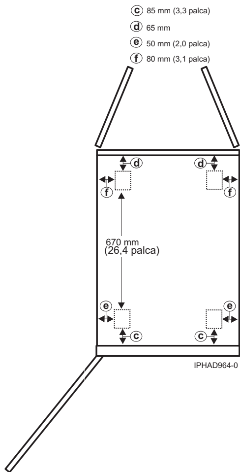
Slika 25. Lokacije kolesa za model 0555 in 7014-S25
