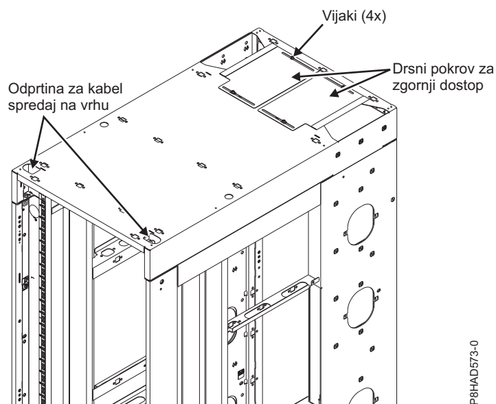
Slika 51. Povezovanje kablov nad glavo
