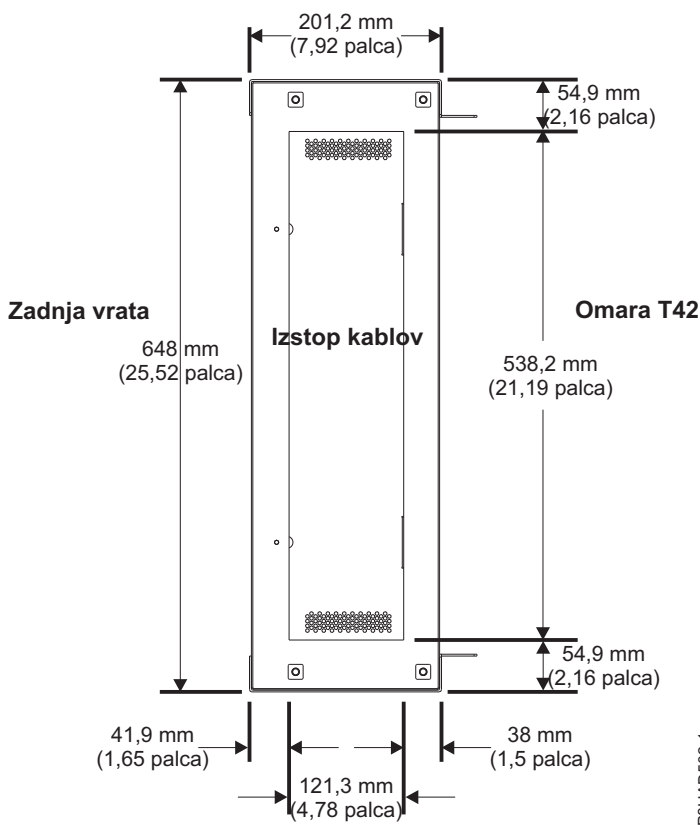
Slika 29. Razširitev zadnjega dela omare, koda možnosti FC ERG0 (pogled od zgoraj navzdol)
