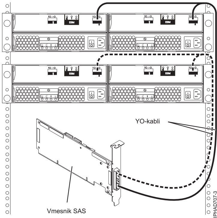
Slika 70. Vmesnik SAS z dvema predaloma za razširitev diskov
