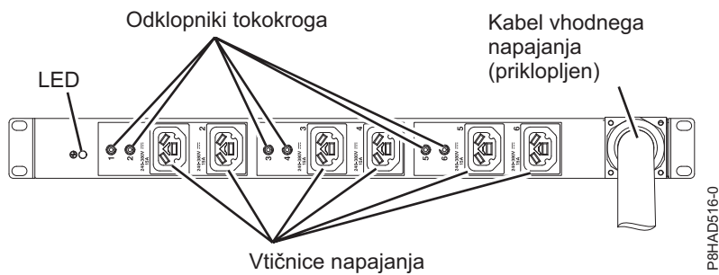
Slika 62. Napajalna distribucijska enota HVDC
