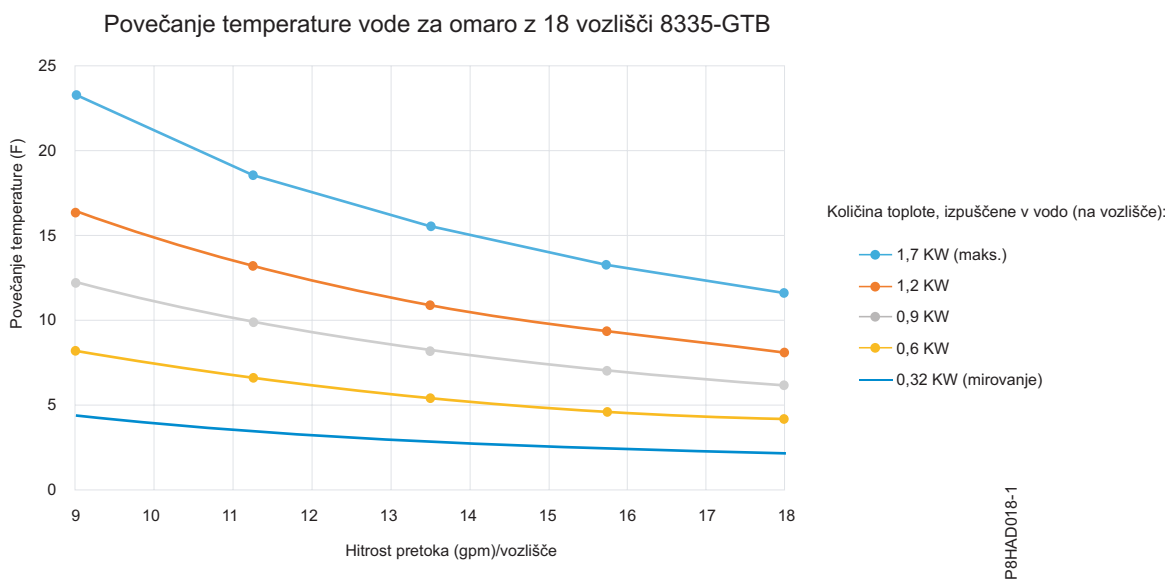
Slika 5. Hitrost pretoka vode v primerjavi s temperaturo dovodne vode - polna omara z 18 strežniki
