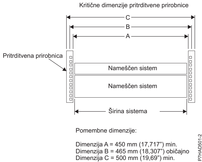
Slika 43. Kritične dimenzije pritrditvene prirobnice
