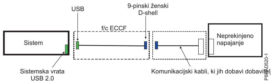
Slika 45. Ožičenje UPS-a za 5148-21L, 5148-22L, 8247-21L, 8247-21L, 8247-22L, 8247-42L, 8284-22A, 8286-41A in 8286-42A
