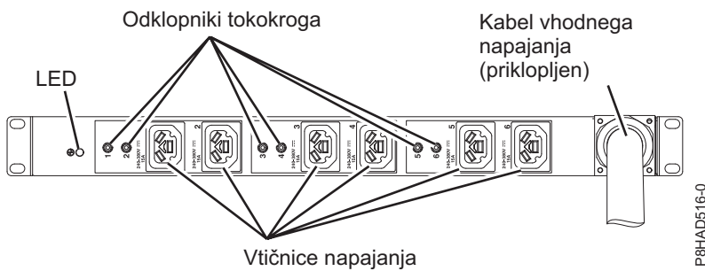
Slika 49. Napajalna distribucijska enota HVDC
