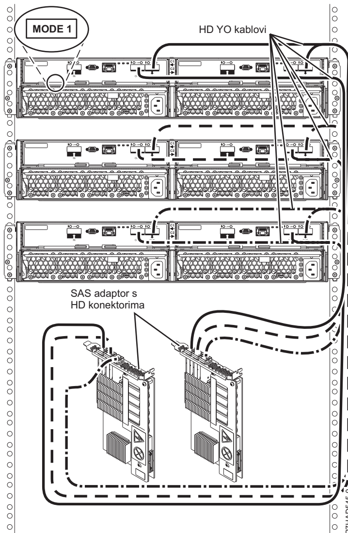
Slika 83. Način 1 povezivanje za tri 5887 kućišta na dva PCIe2 SAS adaptera s HD konektorima
