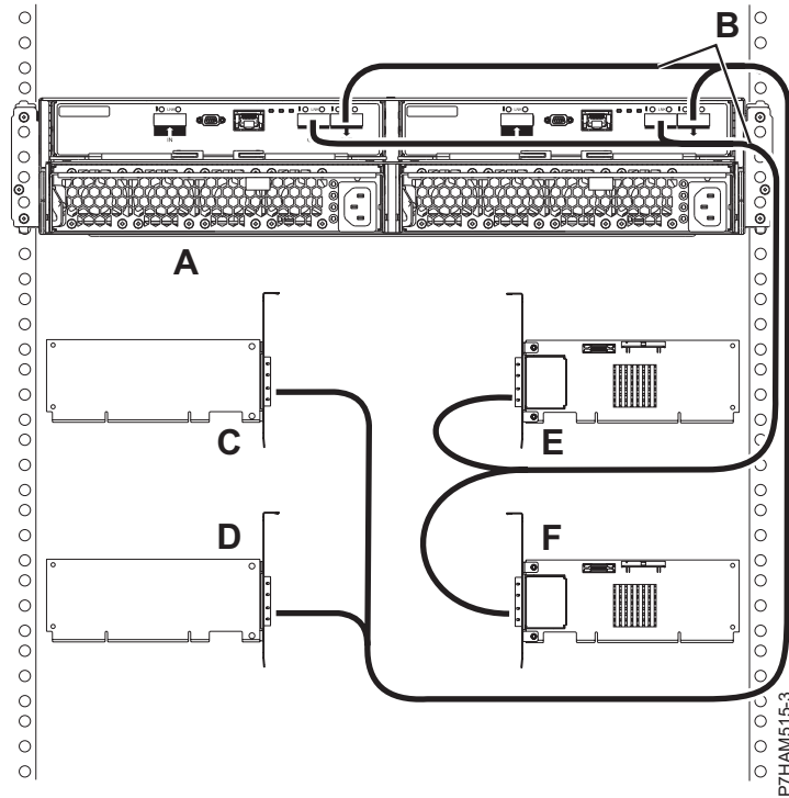
Slika 78. Povezivanje s načinom 4 za 5887 kućište pomoću X kablova na četiri pojedinačna SAS adaptora
