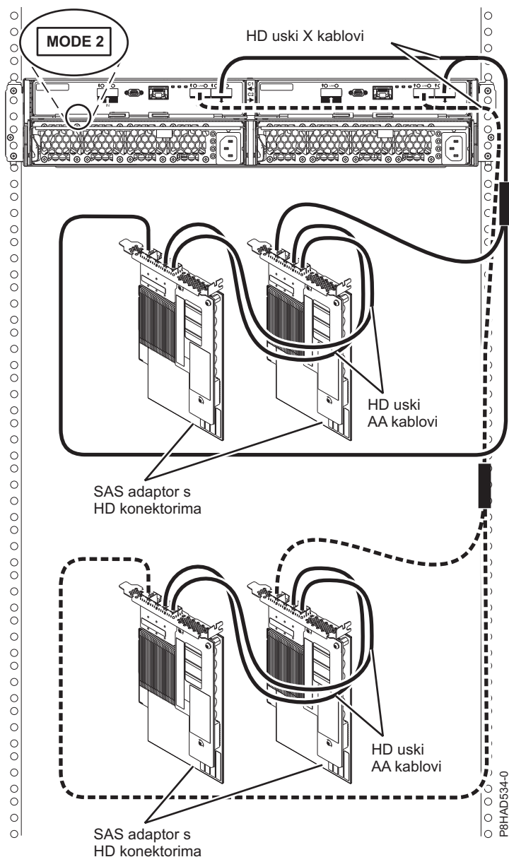
Slika 89. Način 2 povezivanje za 5887 kućište na dva para PCIe3 SAS adaptora s HD uskim konektorima.
