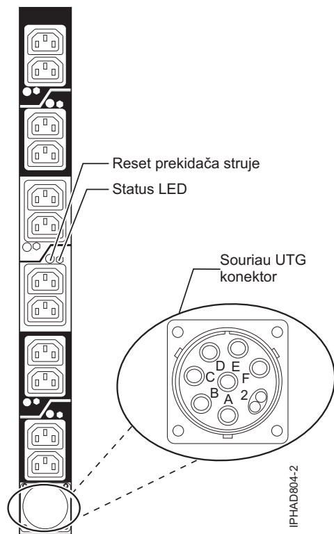
Slika 47. Grafika za PDU utičnice
