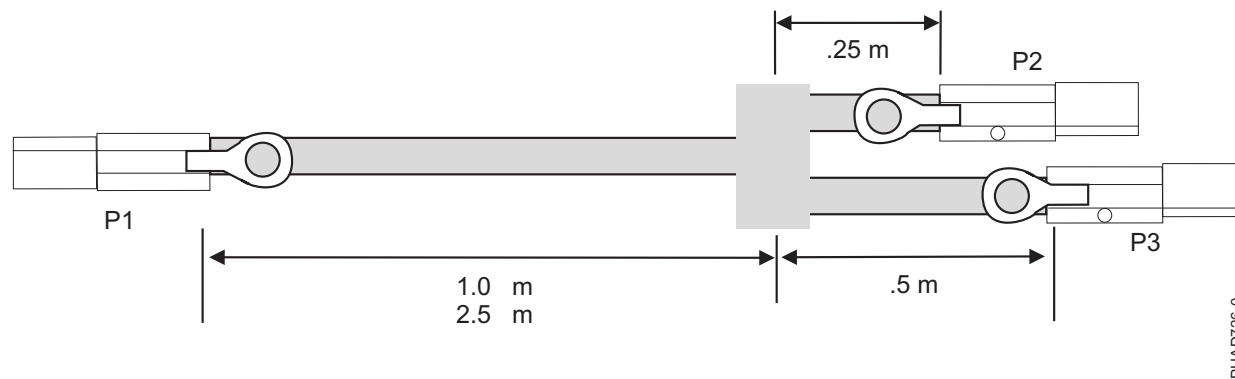
Slika 55. Dužine kablova sklopa SAS eksternih YI kablova
