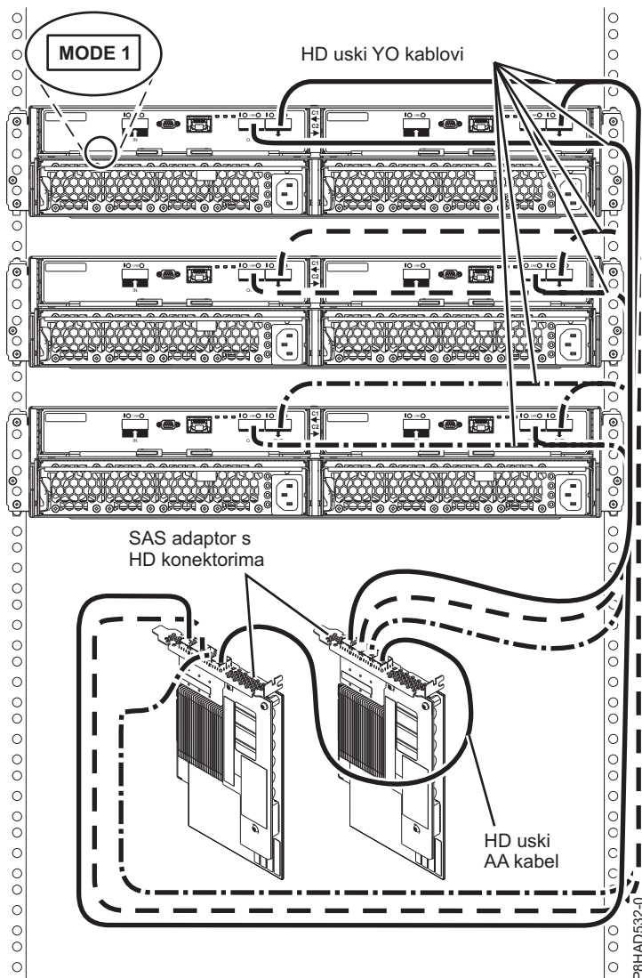
Slika 87. Način 1 povezivanje za tri 5887 kućišta na dva PCIe3 SAS adaptora s HD uskim konektorima
