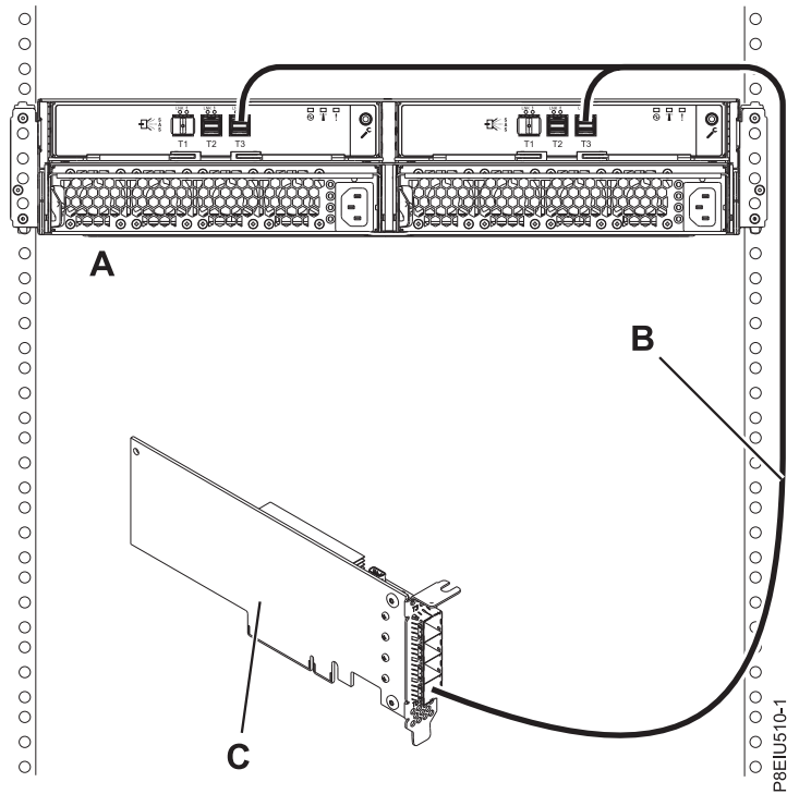
Slika 91. Način 1 povezivanje za jedno ESLL ili ESLS memorijsko kućište s YO12 kablom na jedan SAS adaptor
