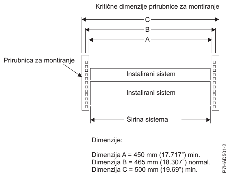
Slika 43. Kritične dimenzije prirubnice za montiranje
