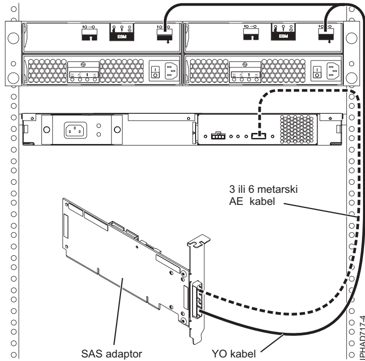
Slika 61. SAS adaptor na pretinac proširenja diska i pretinac proširenja medija
