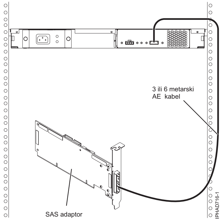
Slika 60. SAS adaptor na pretinac proširenja medija
