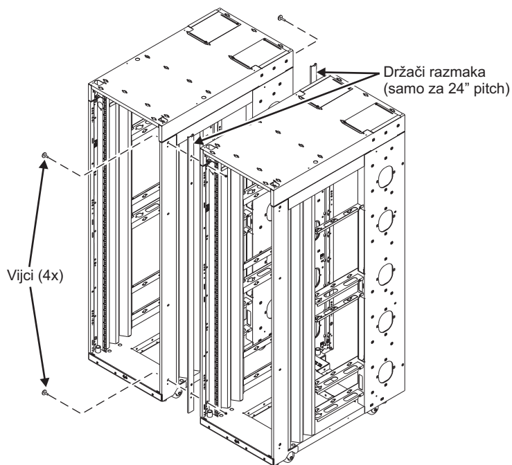
Slika 39. Spajanje više stalaka
