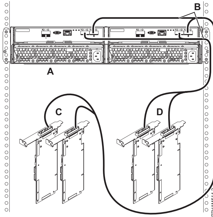
Slika 77. Način 2 povezivanje za 5887 kućište s X kablovima na dva para SAS adaptora
