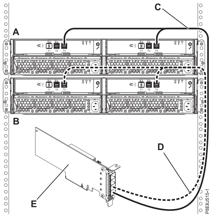
Slika 92. Način 1 povezivanje za dva ESLL ili ESLS memorijska kućišta s YO12 kablovima na jedan SAS adaptor
