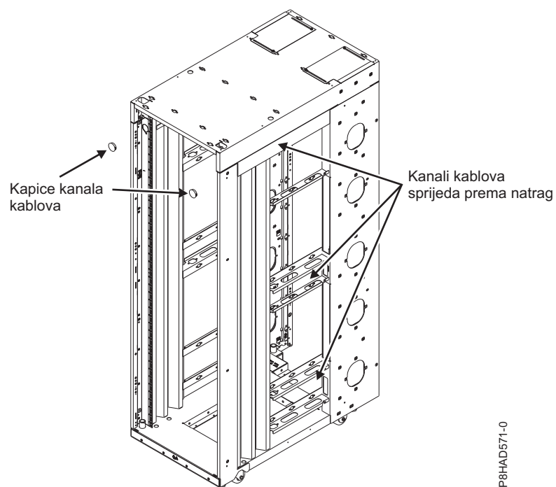
Slika 36. Kabliranje unutar stalka
