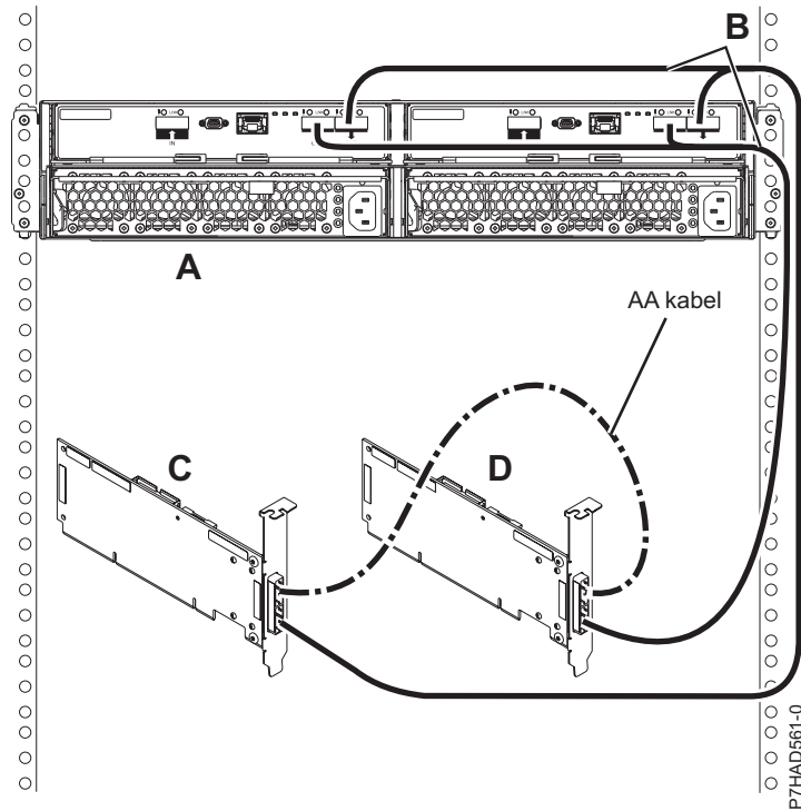
Slika 76. Povezivanje s načinom 2 za 5887 kućište pomoću YO kablova na dva SAS adaptora
