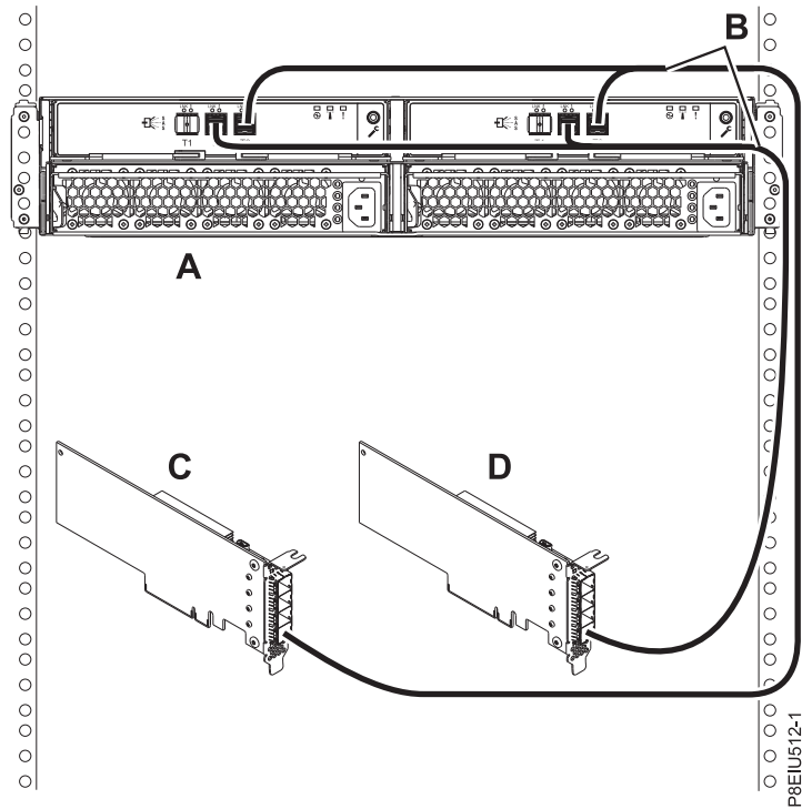
Slika 95. Način 2 povezivanje za ESLL ili ESLS memorijsko kućište s YO12 kablovima na dva nezavisna SAS adaptora
