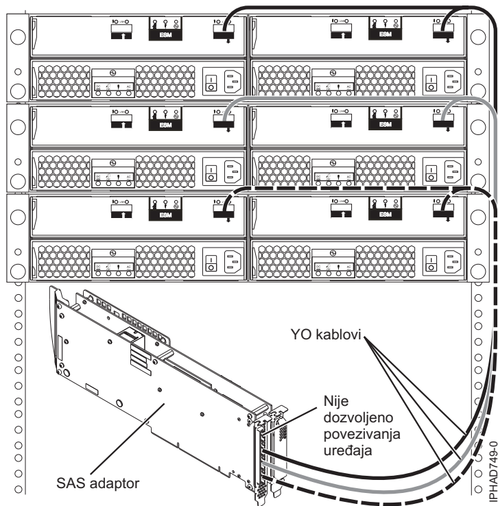
Slika 59. Tri-port SAS adaptor na pretince proširenja diska
