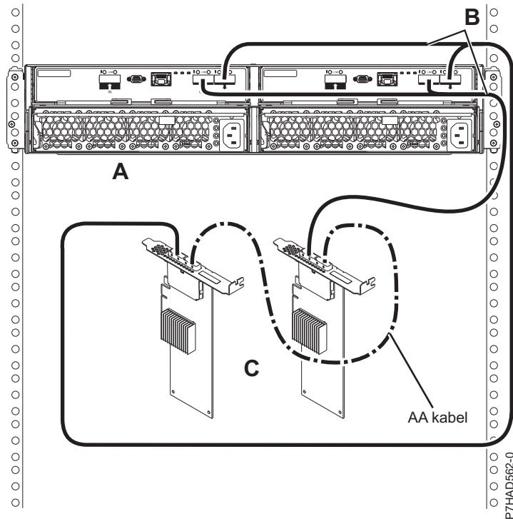
Slika 75. Povezivanje s načinom 1 za 5887 kućište pomoću YO kablova na dva SAS adaptora
