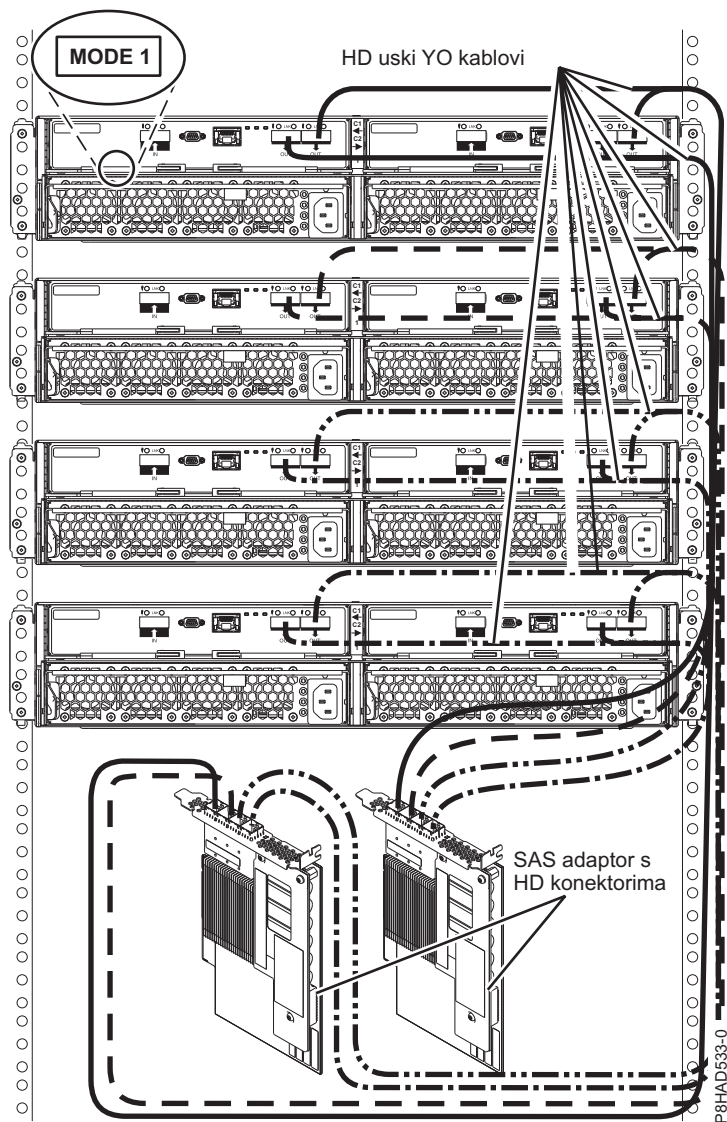
Slika 88. Način 1 povezivanje za četiri 5887 kućišta na dva PCIe3 SAS adaptora s HD uskim konektorima
