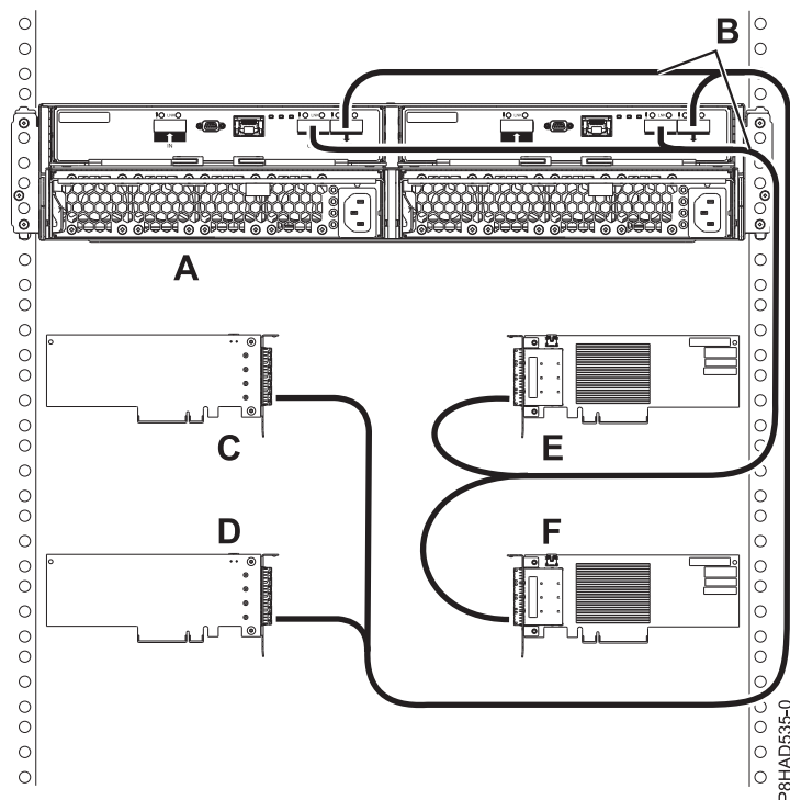
Slika 90. Povezivanje s načinom 4 za 5887 kućište pomoću X kablova na četiri pojedinačna PCIe3 SAS adaptora s HD uskim konektorima.
