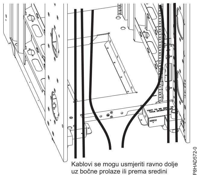
Slika 37. Kabliranje ispod poda
