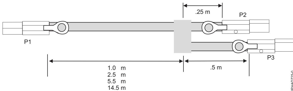
Slika 54. Dužine kablova sklopa SAS eksternih YO kablova
