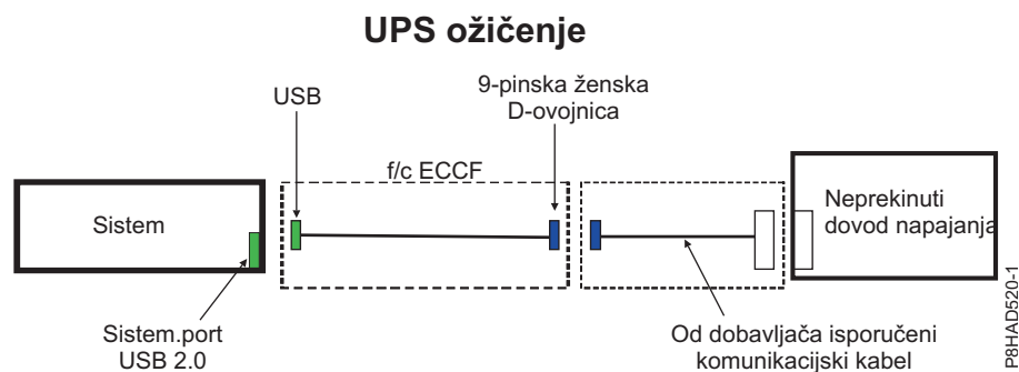
Slika 45. UPS ožičenje za 5148-21L, 5148-22L, 8247-21L, 8247-21L, 8247-22L, 8247-42L, 8284-22A, 8286-41A i 8286-42A
