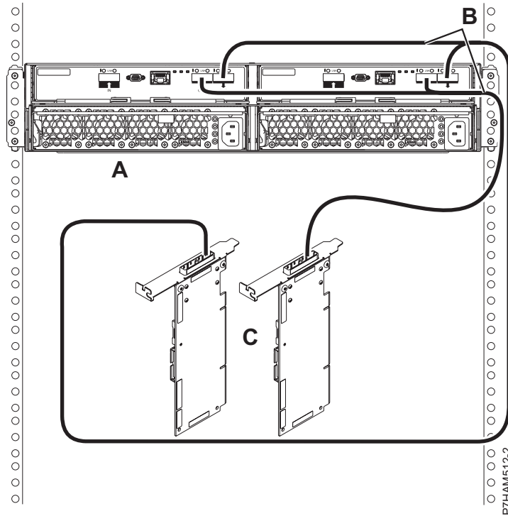
Slika 79. Povezivanje s načinom 1 za 5887 kućište pomoću YO kablova na dva SAS adaptora
