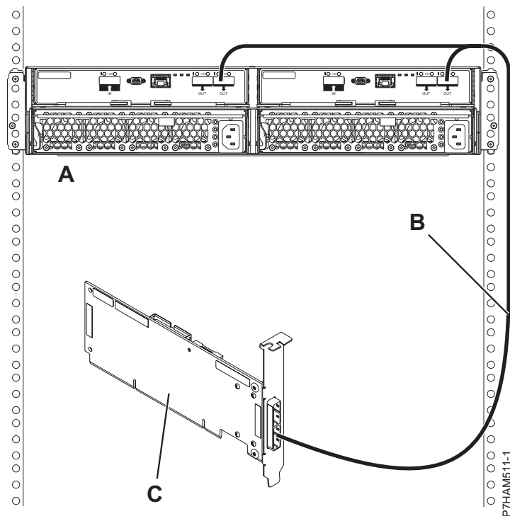
Slika 74. Način 1 povezivanje za 5887 kućište s YO kablom na jedan SAS adaptor
