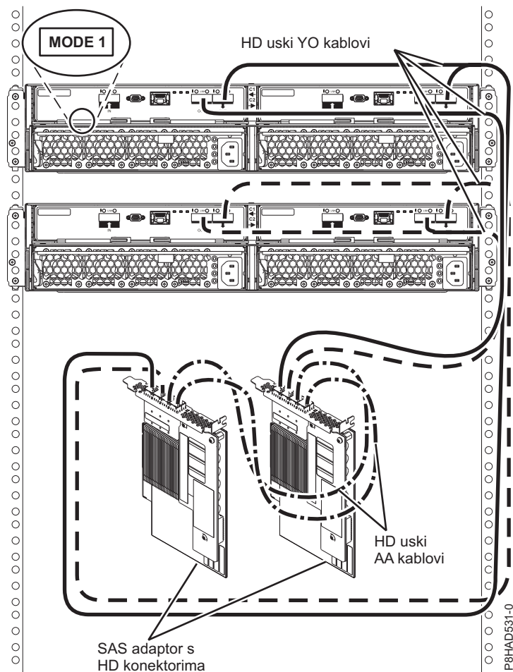
Slika 86. Način 1 povezivanje za dva 5887 kućišta na dva PCIe3 SAS adaptora s HD uskim konektorima
