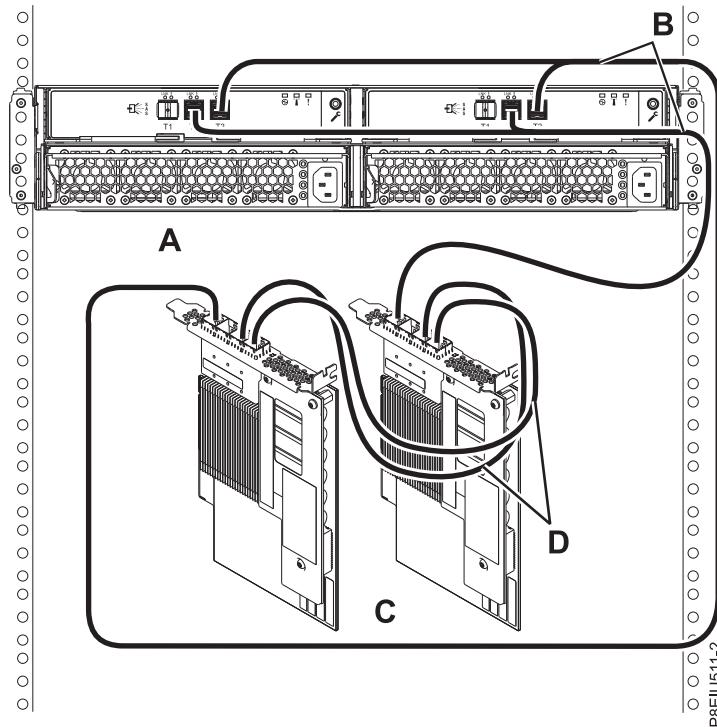
Slika 93. Način 1 povezivanje za jedno ESLL ili ESLS memorijsko kućište s YO12 kablovima na jedan par SAS adaptora
