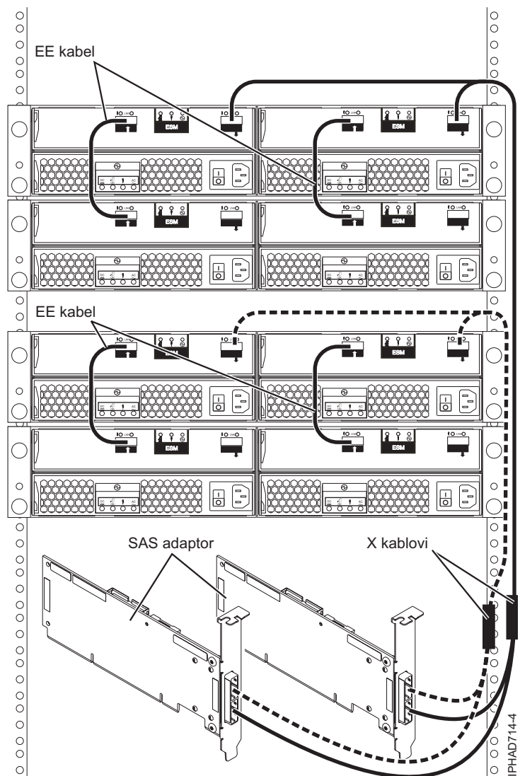
Slika 67. Dva SAS adaptoru na četiri pretinca proširenja diska u HA RAID konfiguraciji
