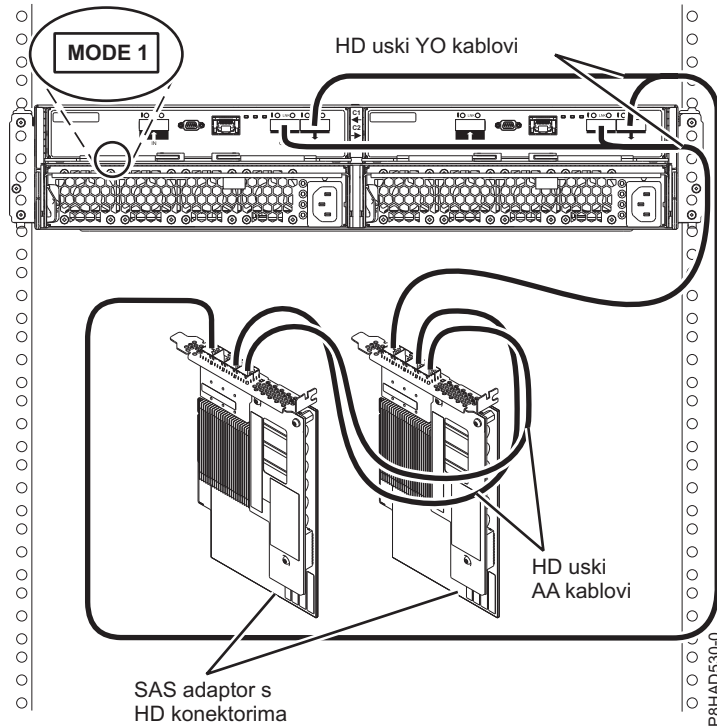
Slika 85. Način 1 povezivanje za 5887 kućište na dva PCIe3 SAS adaptora s HD uskim konektorima
