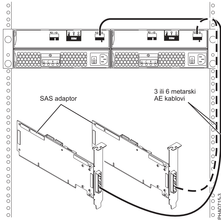
Slika 73. Dva RAID SAS adaptorora na pretinac proširenja diska u višepokretnoj HA JBOD konfiguraciji
