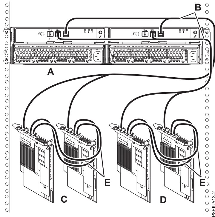
Slika 96. Način 2 povezivanje za jedno ESLL ili ESLS memorijsko kućište s X12 kablovima na dva para SAS adaptora
