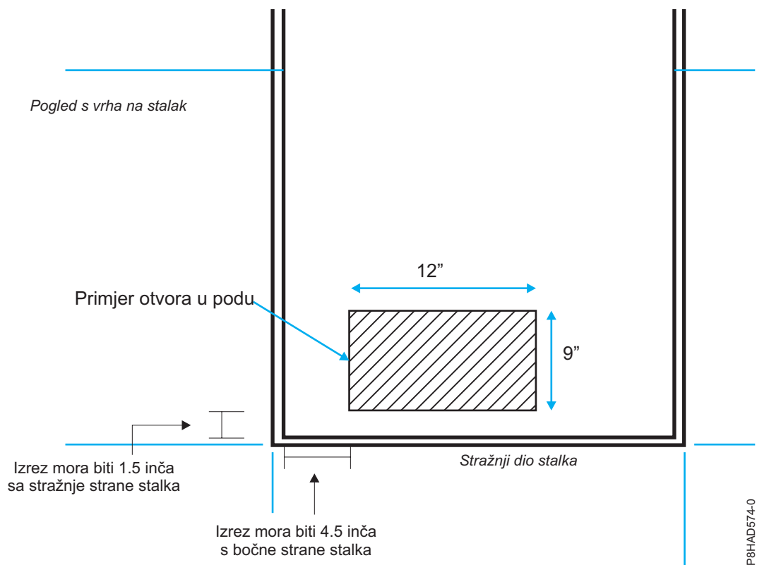
Slika 35. Otvor na podu
