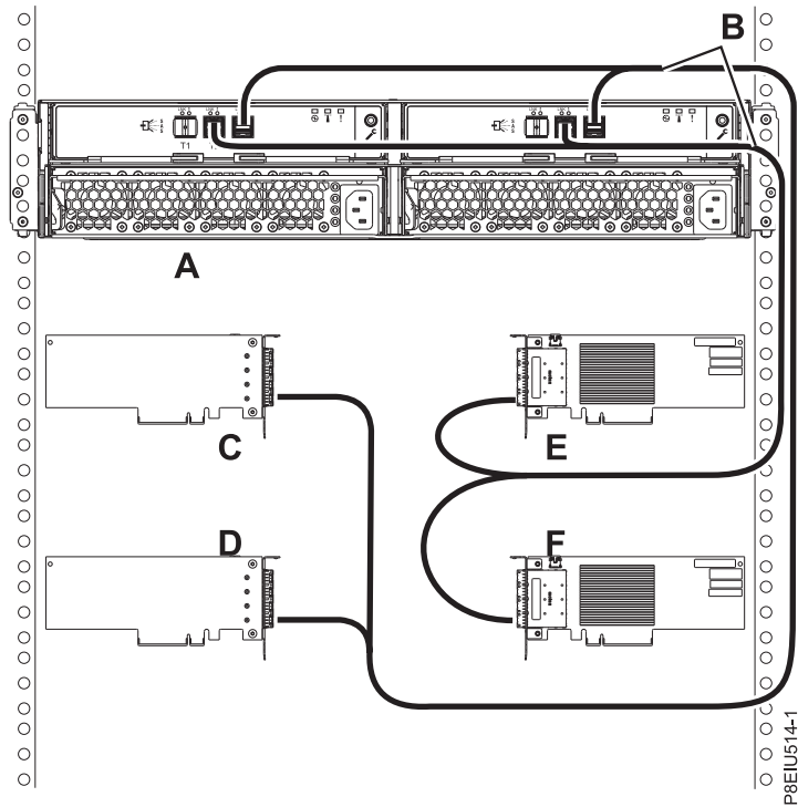
Slika 97. Način 4 povezivanje za jedno ESLL ili ESLS memorijsko kućište s X12 kablovima na četiri nezavisna SAS adaptora
