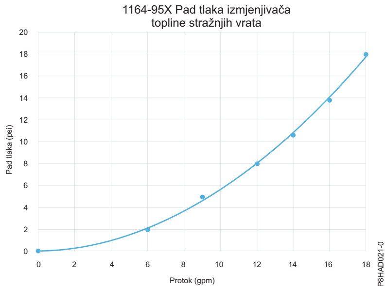
Slika 42. Pad tlaka (standardne jedinice)
