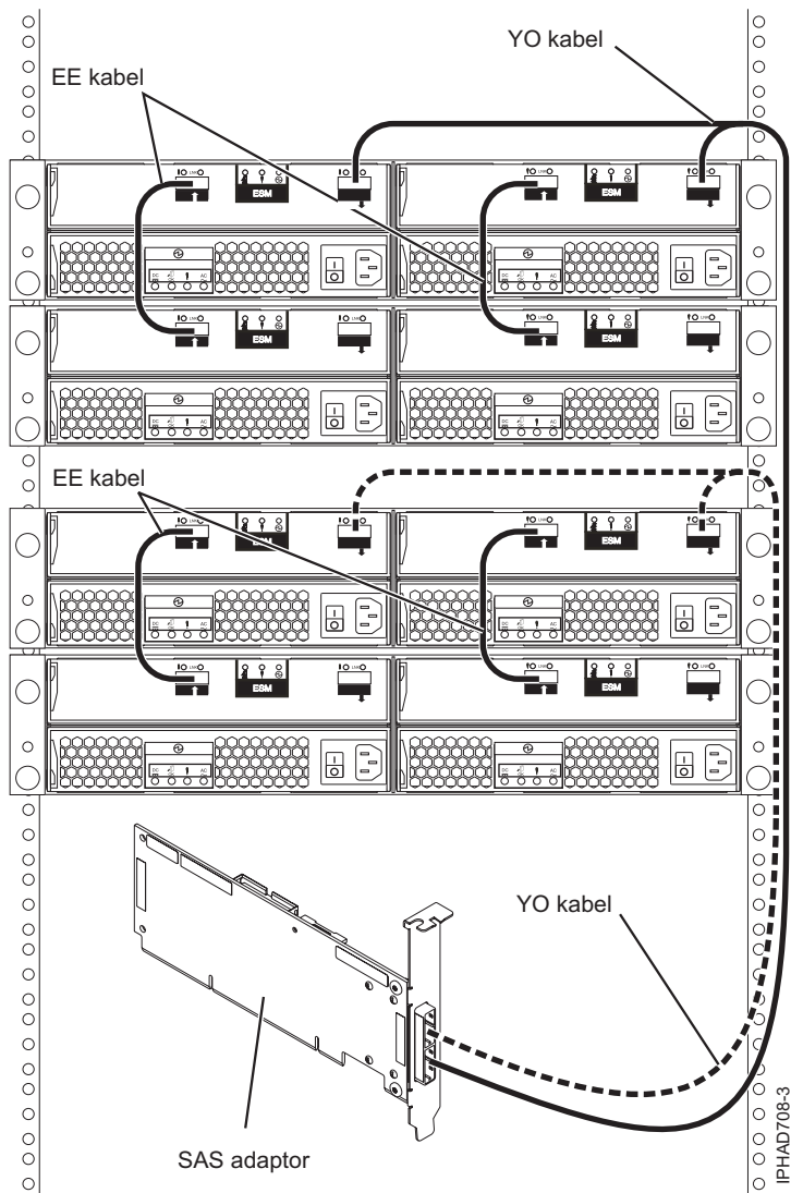
Slika 58. SAS adaptor na četiri pretinca proširenja diska
