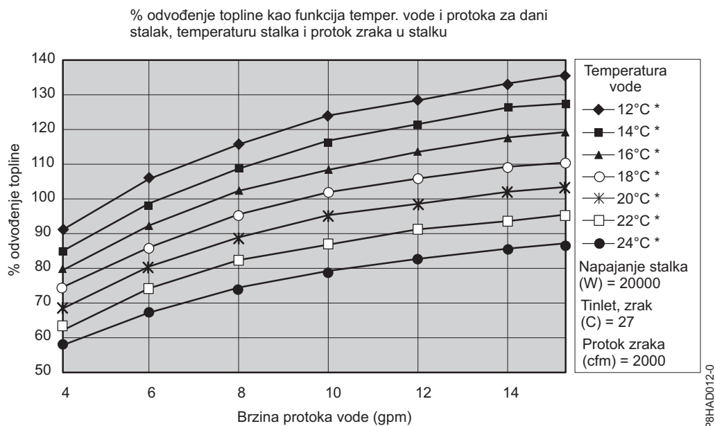
Slika 40. Tipične performanse izmjenjivača topline, 20 kW opterećenje topline
