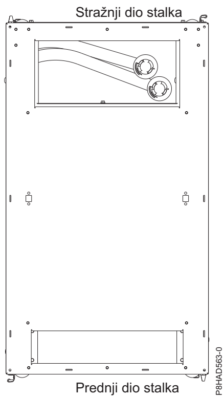
Slika 43. Lokacije izlaza cijevi na vrhu (gledano odozgo)
