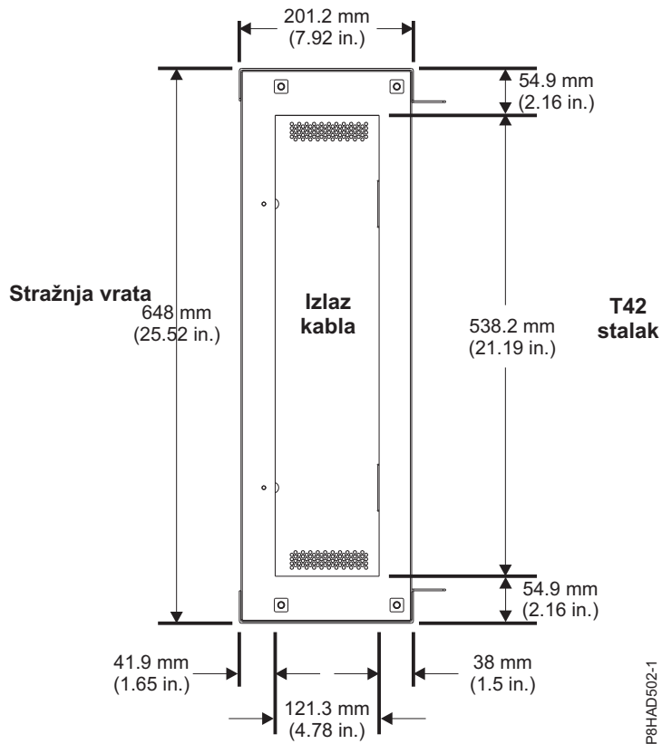
Slika 29. FC ERG0 proširenje staka (pogled odozgo)
