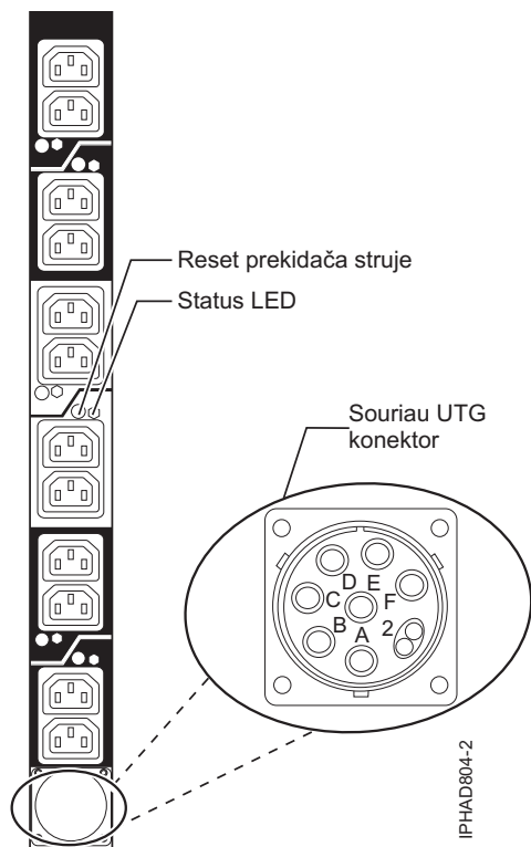
Slika 60. Grafika za PDU utičnice
