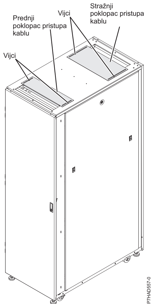
Slika 34. Poklopci pristupa kablovima
