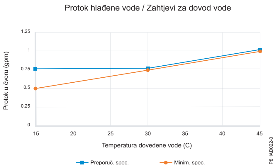
Slika 2. Brzina protoka ohlađene vode u usporedbi sa zahtjevima za dovod vode (standardne jedinice)
