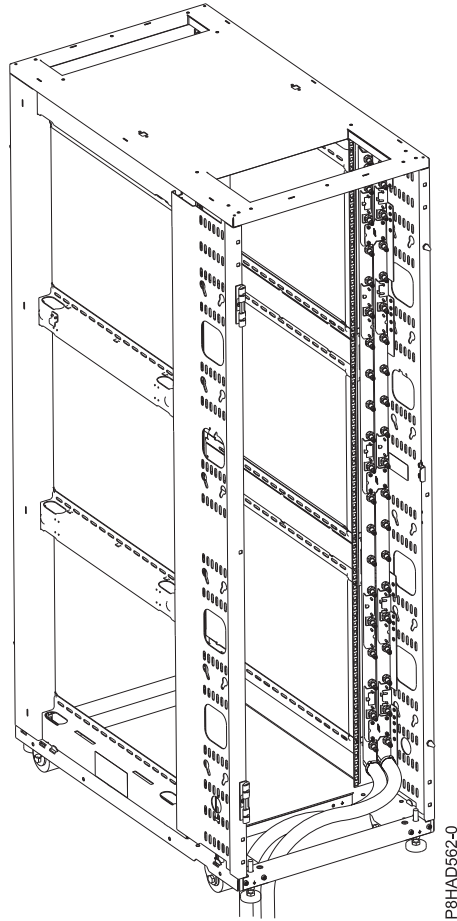
Slika 41. Stalak i cjevovod s dovodnim i povratnim cijevima koje izlaze na dnu stalka
