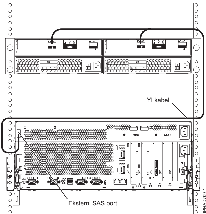
Slika 75. Sistemski eksterni port SAS adaptora na pretinac proširenja diska
