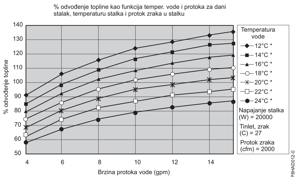
Slika 37. Tipične performanse izmjenjivača topline, 20 kW opterećenje toplinom
