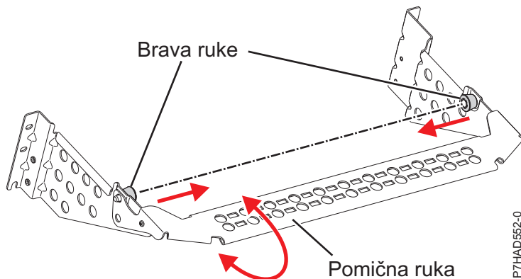
Slika 65. Držači za upravljanje kablovima
