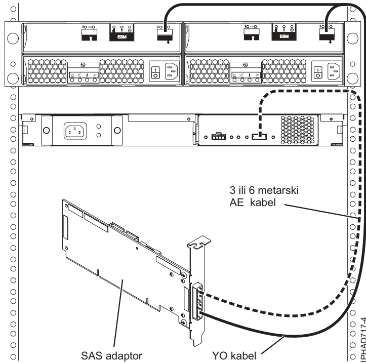
Slika 74. SAS adaptor na pretinac proširenja diska i pretinac proširenja medija
