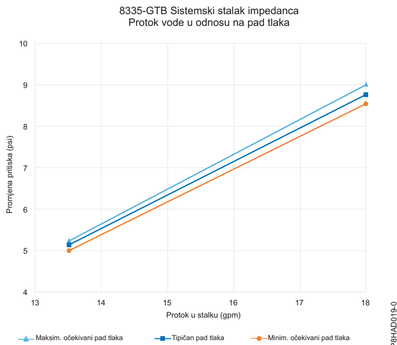
Slika 3. Brzina protoka u odnosu na pad tlaka (standardne jedinice) - stalak napunjen s 18 poslužitelja
