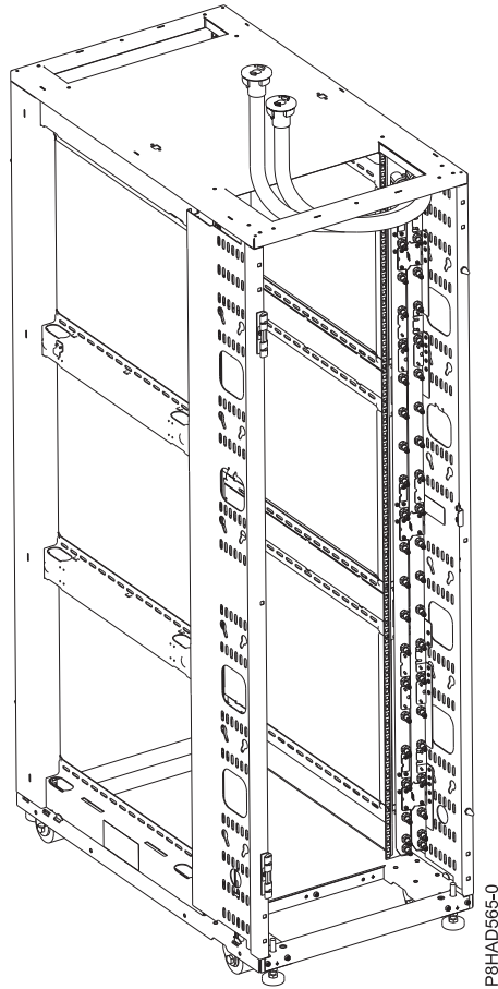
Slika 40. Stalak i cjevovod s dovodnim i povratnim cijevima koje izlaze na vrhu stalka
