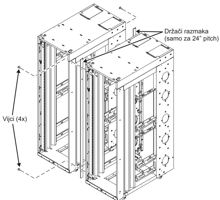
Slika 52. Spajanje više stalaka
