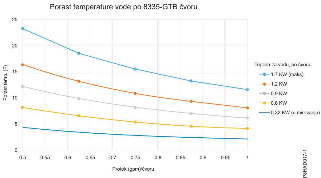
Slika 4. Brzina protoka vode u odnosu na temperaturu dovedene vode - jedan poslužitelj (standardne jedinice)
