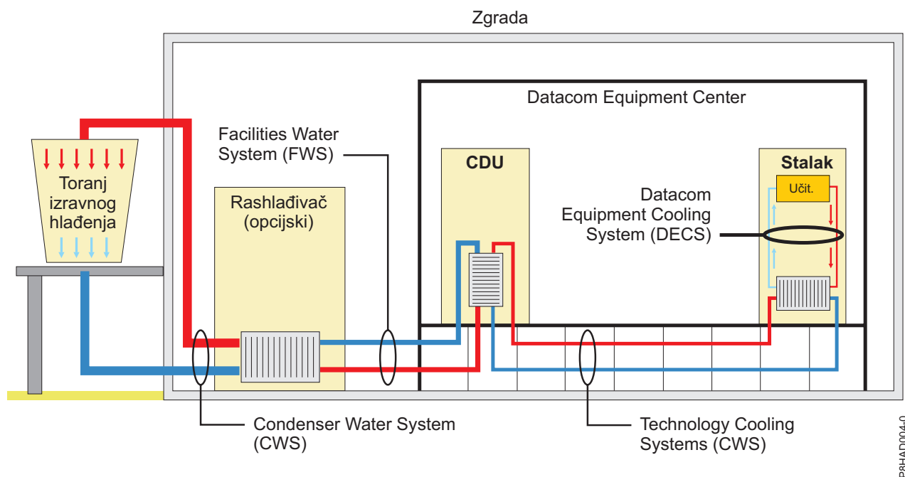
Slika 87. Primjer sistema za hlađenje tekućinom i krugova unutar centra podataka
