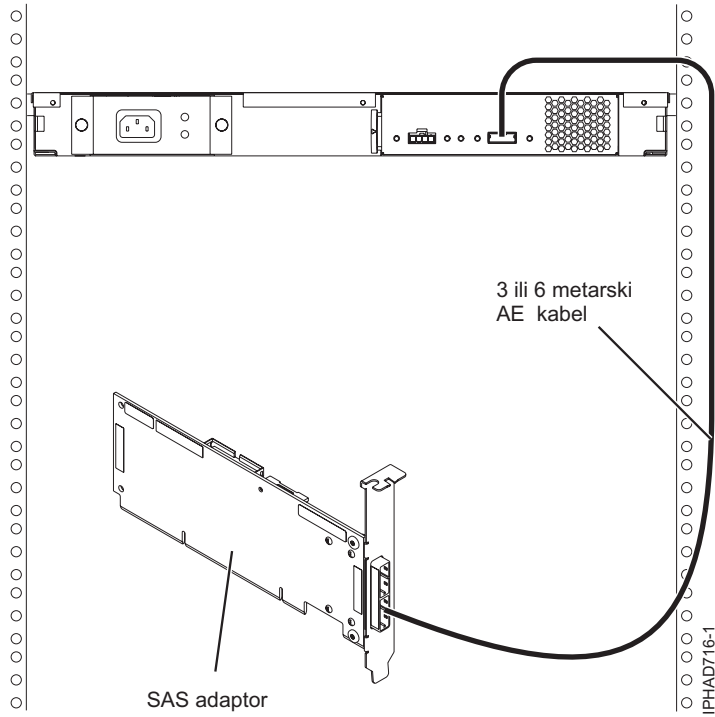
Slika 73. SAS adaptor na pretinac proširenja medija
