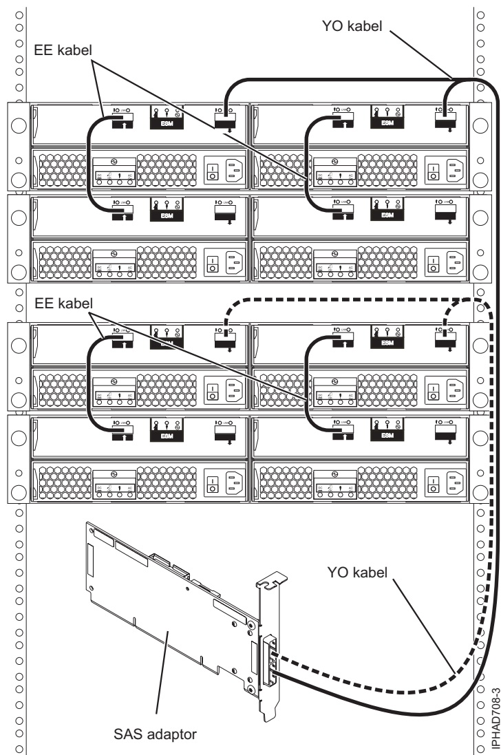
Slika 71. SAS adaptor na četiri pretinca proširenja diska
