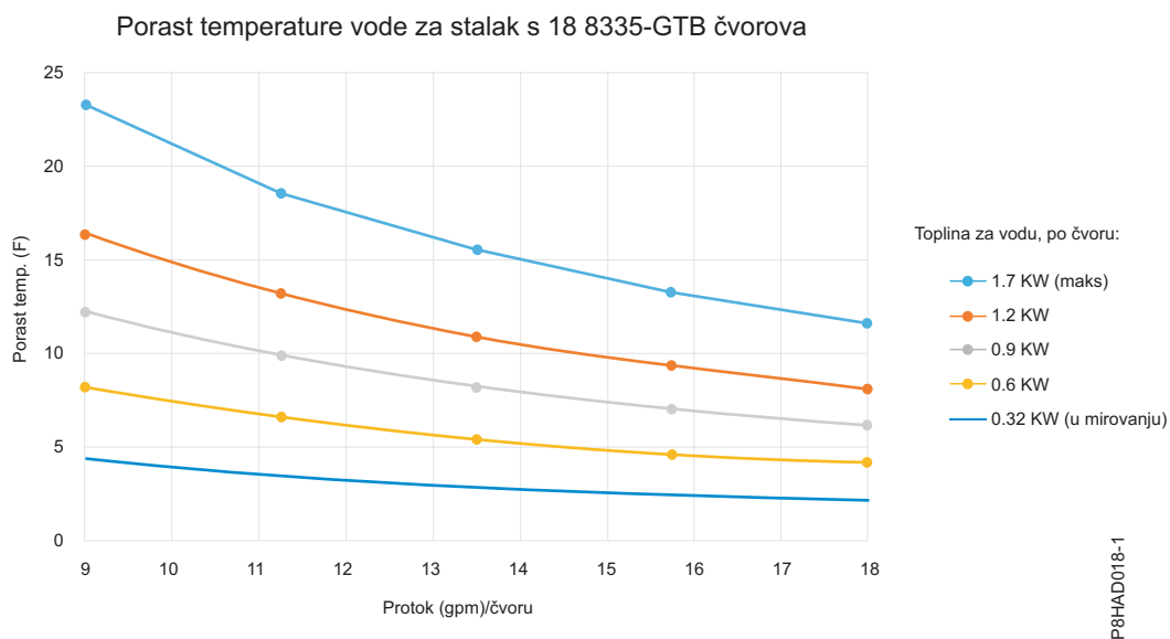
Slika 5. Brzina protoka vode u odnosu na temperaturu dovedene vode - puni stalak s 18 poslužitelja
