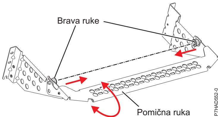
Slika 52. Držači za upravljanje kablovima
