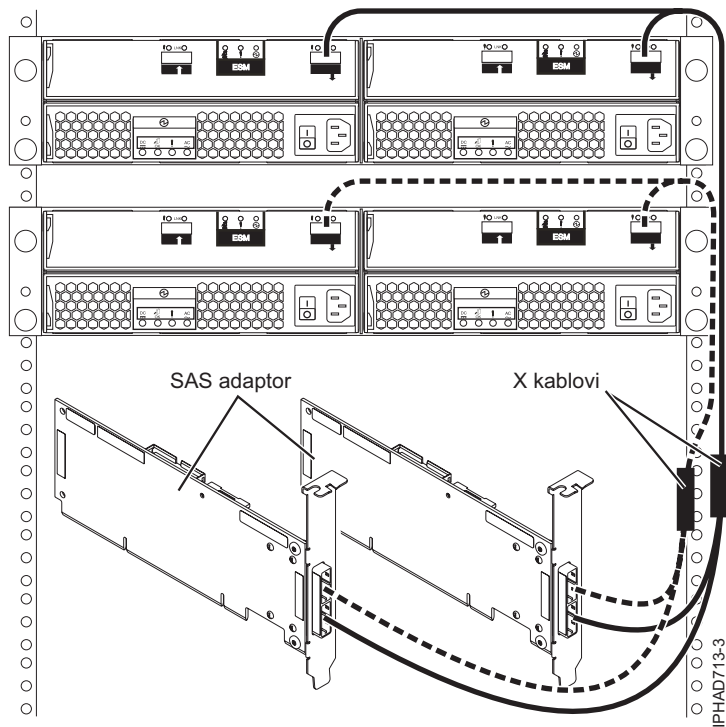
Slika 66. Dva SAS adaptorora na pretince proširenja diska u HA RAID konfiguraciji
