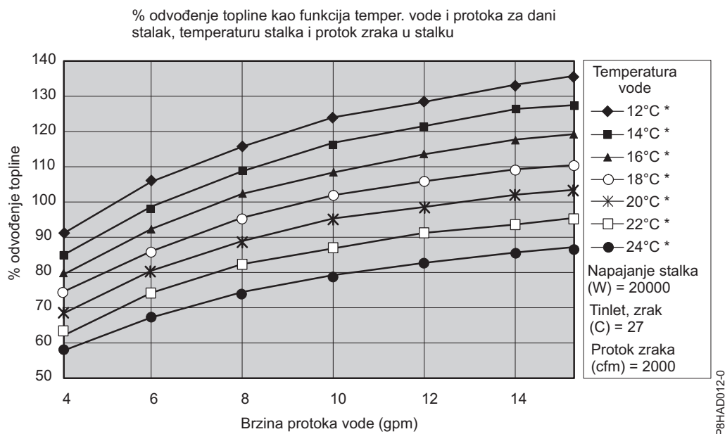
Slika 40. Tipične performanse izmjenjivača topline, 20 kW opterećenje toplinom
