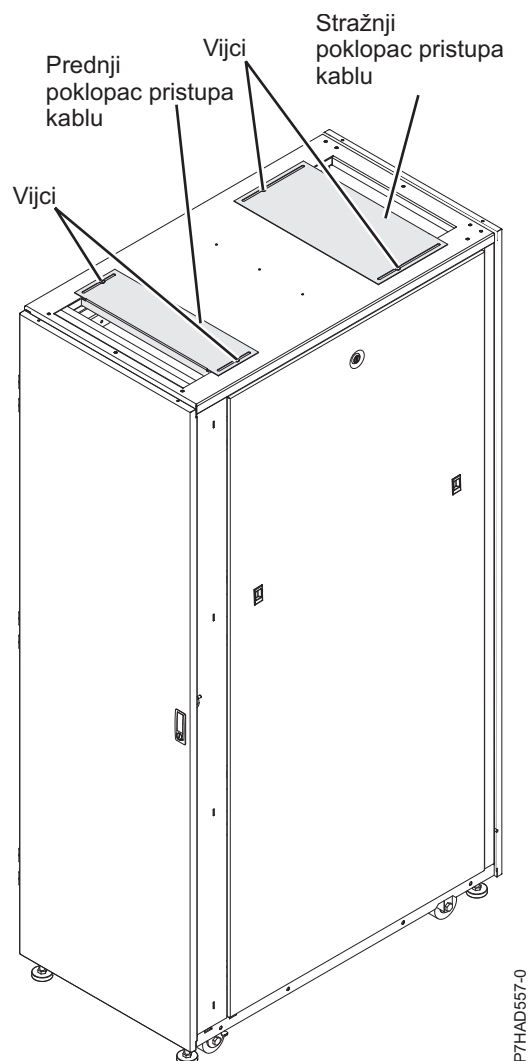
Slika 29. Poklopci pristupa kablovima
