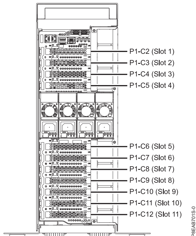
Slika 3. Pogled straga na samostalni 8286-41A sistem sa šiframa lokacija PCIe priključnica.
