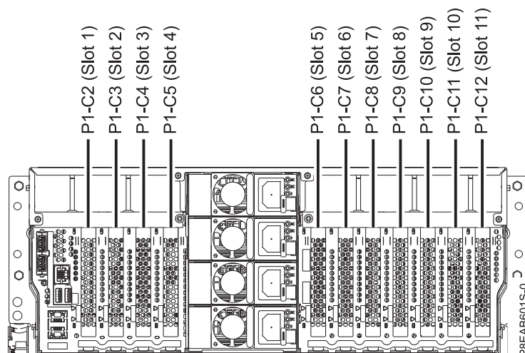
Slika 1. Pogled straga na 8247-42L sistem montiran u stalak sa šiframa lokacije PCIe priključnica
