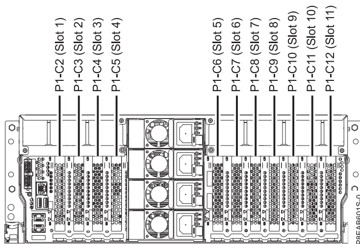
Slika 2. Pogled straga na 8286-41A i 8286-42A sistem montiran u stalak sa šiframa lokacija PCIe priključnica
