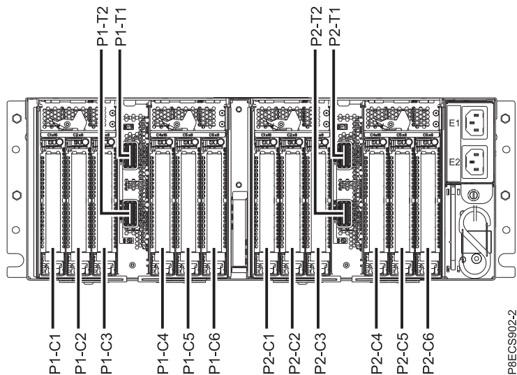
Slika 4. Pogled straga na EMX0 PCIe3 pretinac proširenja sa šiframa lokacija PCIe priključnica
