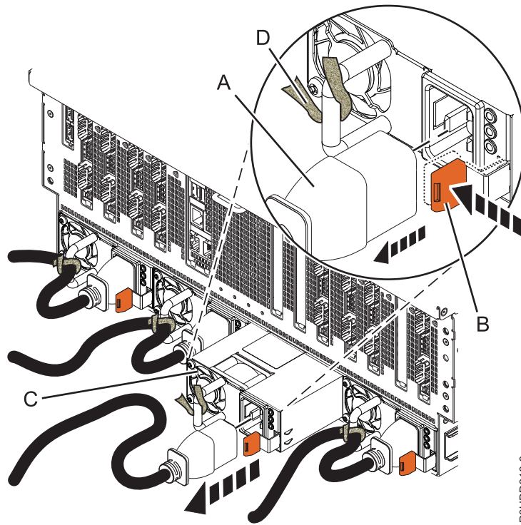
Figure 3. Retrait d'un bloc d'alimentation du système 8408-44E
