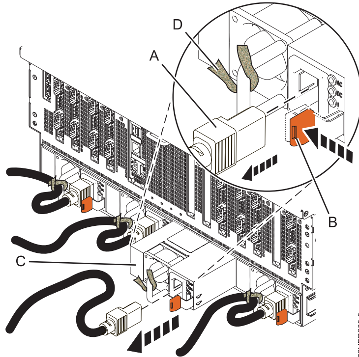
Figure 4. Retrait d'un bloc d'alimentation du système 8408-E8E
