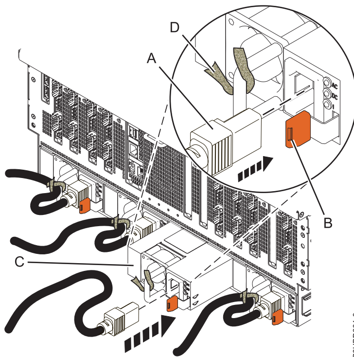
Figure 6. Remise en place d'un bloc d'alimentation dans le système 8408-E8E
