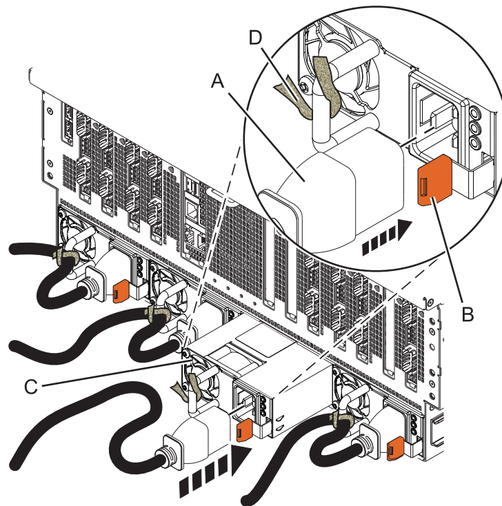
Figure 5. Remise en place d'un bloc d'alimentation dans le système 8408-44E
