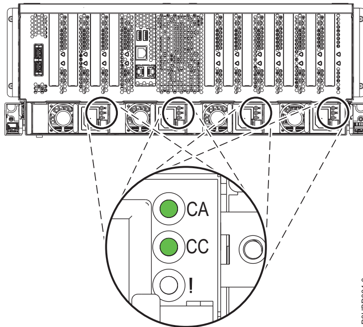
Figure 14. Voyants d'un bloc d'alimentation en cours de fonctionnement
