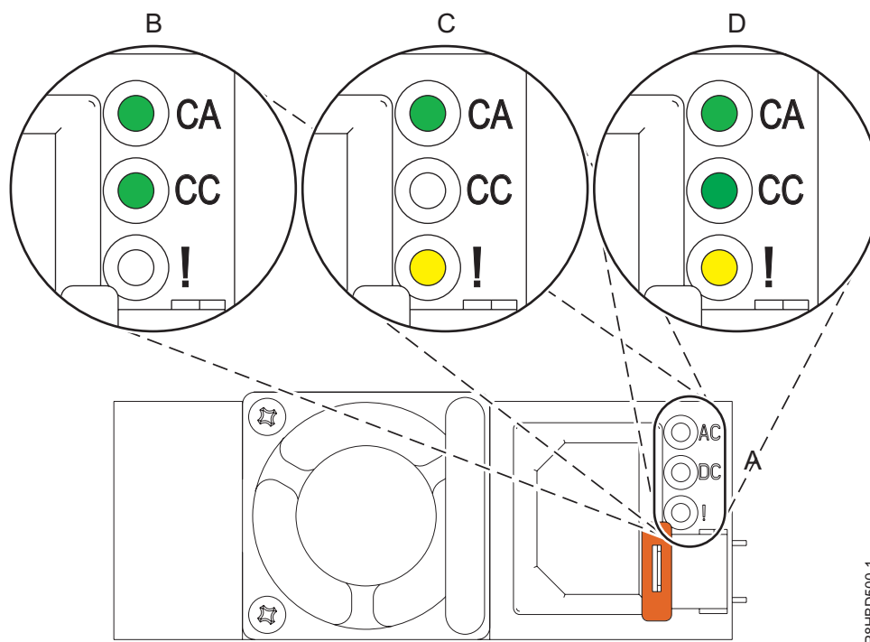
Figure 2. Voyants d'un bloc d'alimentation opérationnel et défaillant
