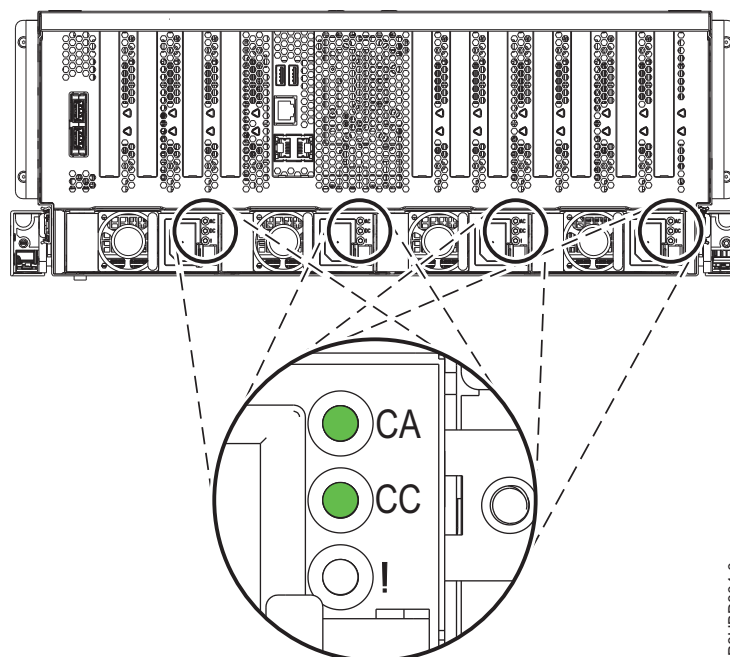
Figure 7. Voyants d'un bloc d'alimentation en cours de fonctionnement
