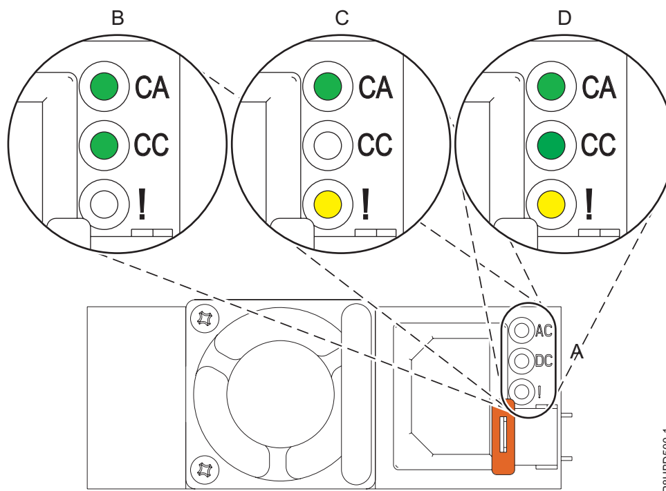
Figure 9. Voyants d'un bloc d'alimentation opérationnel et défectueux
