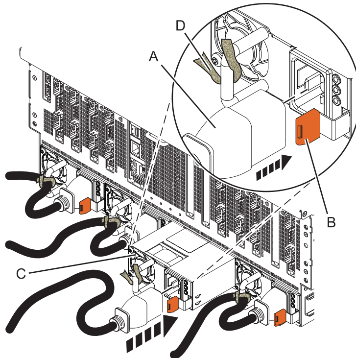
Figure 12. Remise en place d'un bloc d'alimentation dans le système 8408-44E
