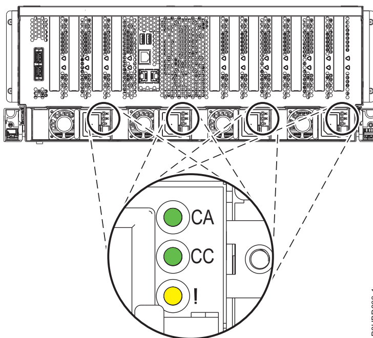
Figure 8. Emplacement des blocs d'alimentation et des voyants dans un système 8408-44E ou 8408-E8E
