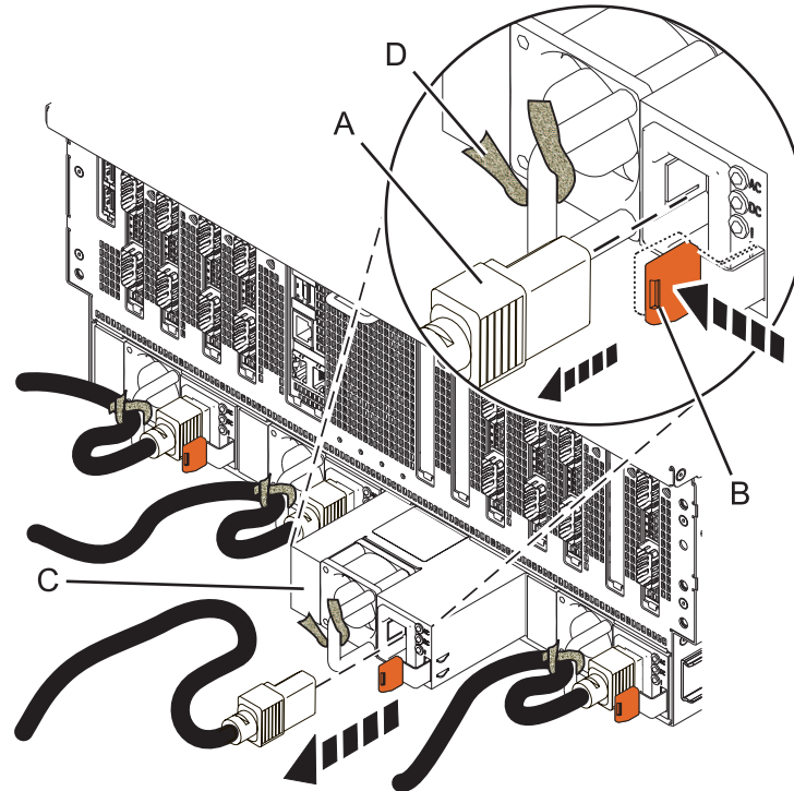
Figure 11. Retrait d'un bloc d'alimentation du système 8408-E8E
