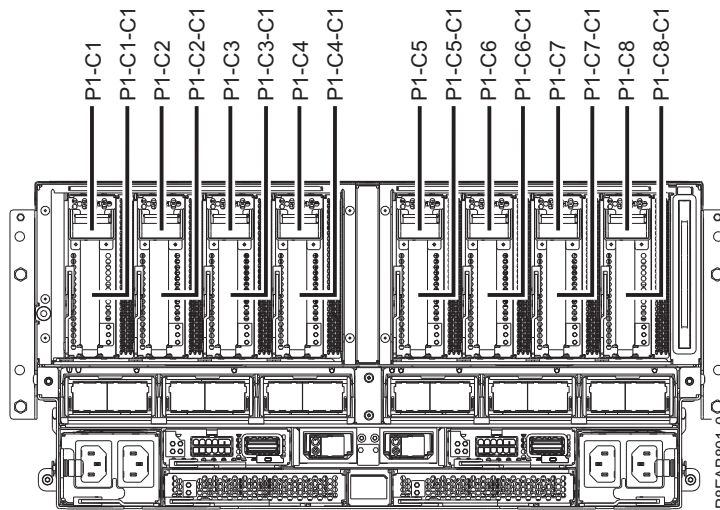
Figure 1. Vue arrière d'un système 9080-MHE, 9080-MME 9119-MHE ou 9119-MME avec codes d'emplacement PCIe
