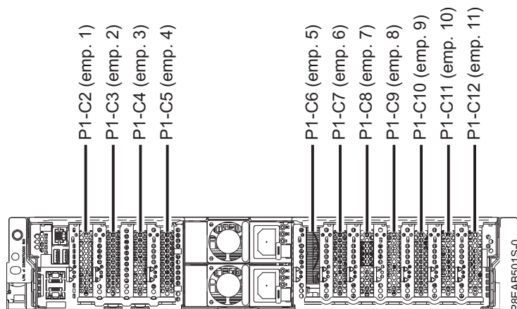
Figure 1. Vue arrière des systèmes 5148-21L, 5148-22L, 8247-21L, 8247-22L, 8284-21A ou 8284-22A avec codes d'emplacement PCIe
