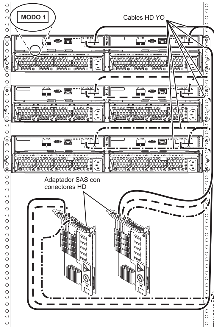
Figura 83. Conexión de modalidad 1 de tres alojamientos 5887 a dos adaptadores SAS PCIe2 con conectores HD
