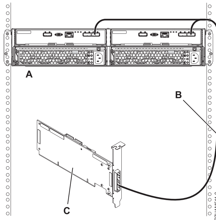
Figura 74. Conexión de modalidad 1 de un alojamiento 5887 mediante un cable YO a un único adaptador SAS
