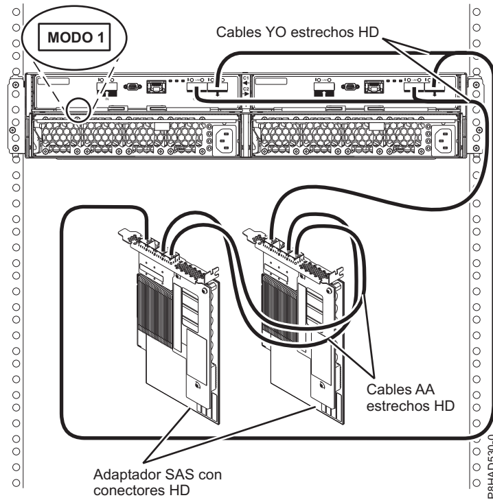
Figura 85. Conexión de modalidad 1 de un alojamiento 5887 a dos adaptadores SAS PCIe3 con conectores estrechos HD.
