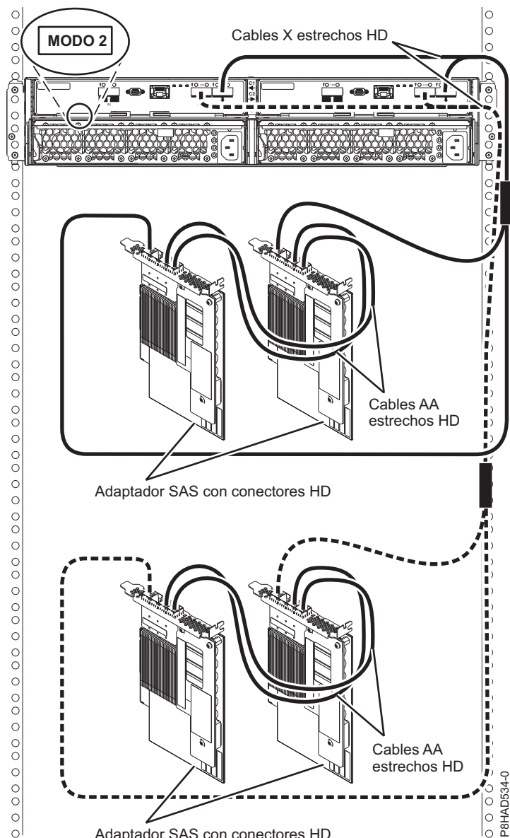
Figura 89. Conexión de modalidad 2 de un alojamiento 5887 a dos pares de adaptadores SAS PCIe3 con conectores estrechos HD.
