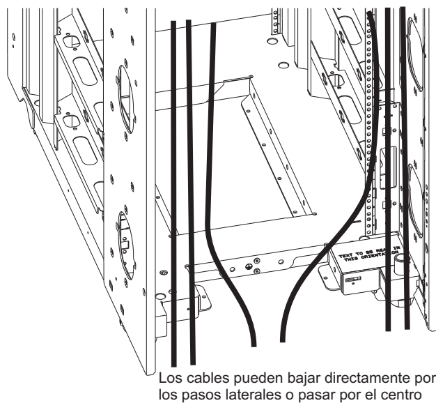
Figura 37. Cableado bajo el suelo
