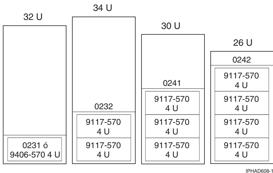
Figura 7. 570 en bastidor
