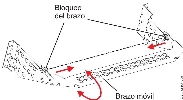
Figura 52. Abrazadera portacables
