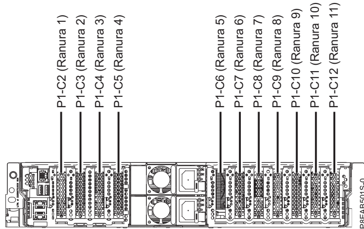
Figura 1. Vista posterior de un sistema 5148-21L, 5148-22L, 8247-21L, 8247-22L, 8284-21A o 8284-22A con códigos de ubicación de ranuras PCIe
