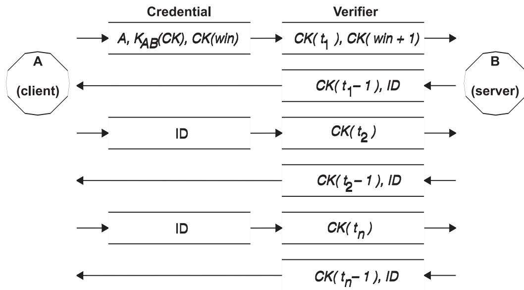
Rysunek 15. Proces uwierzytelniania. Ten rysunek przedstawia proces uwierzytelniania.
