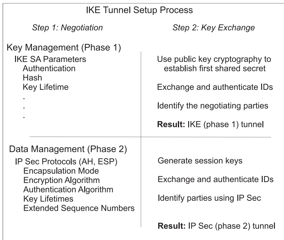
Rysunek 9. Proces konfigurowania tunelu IKE
