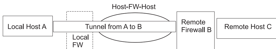
Rysunek 14. Host-Firewall-Host
