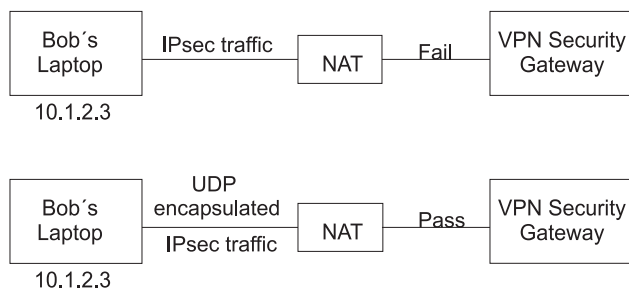
Rysunek 12. Bezpieczeństwo IP z włączoną translacją NAT
