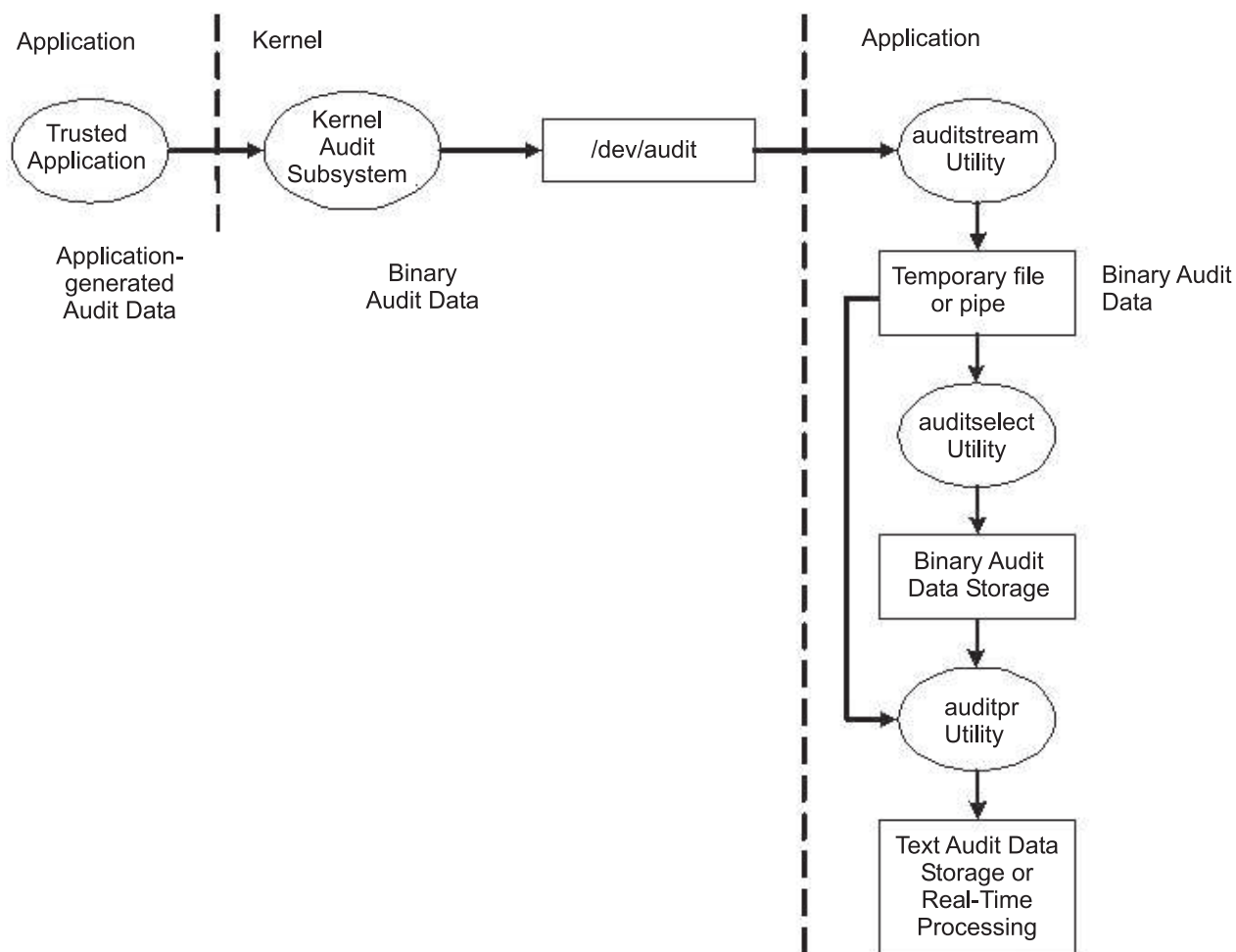
Rysunek 2. Proces trybu kontroli STREAM. Ta ilustracja przedstawia proces trybu kontroli STREAM.
