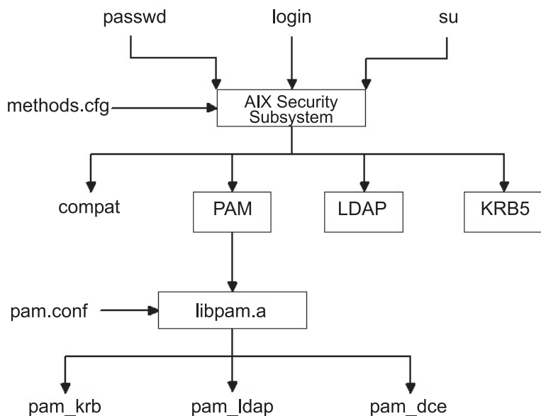
Rysunek 5. Ścieżka między usługami zabezpieczeń systemu AIX i modulem PAM
