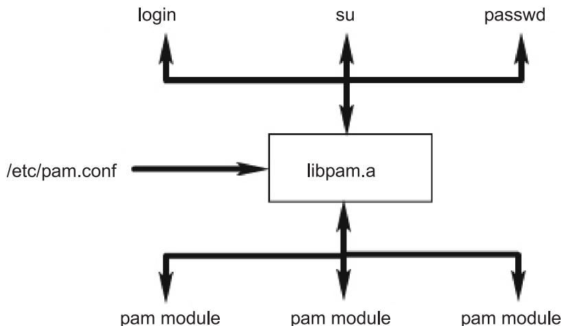
Rysunek 3. Struktura i elementy modułu PAM. Rysunek pokazuje, w jaki sposób komendy z włączoną obsługą PAM korzystają z biblioteki PAM, aby uzyskać dostęp do odpowiedniego modułu PAM.
