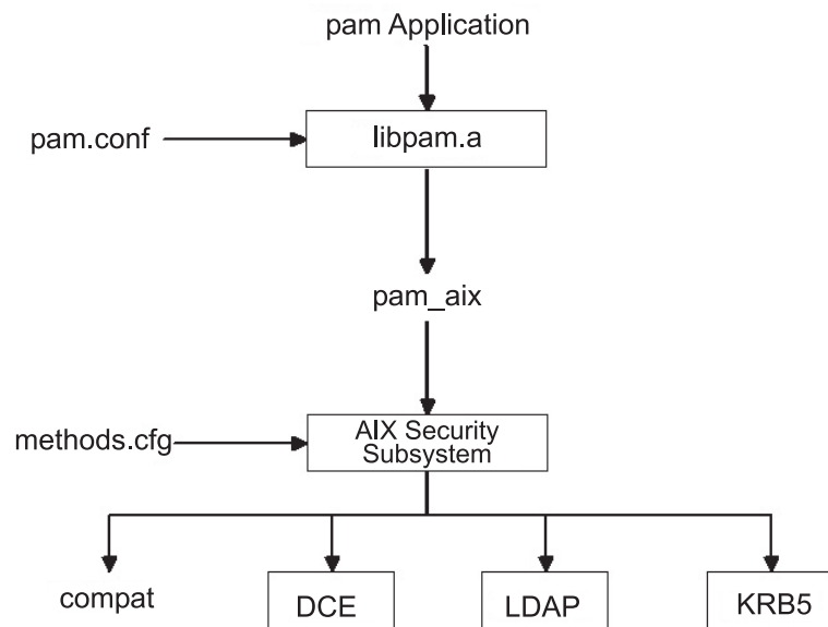
Rysunek 4. Ścieżka między aplikacją PAM a podsystemem bezpieczeństwa systemu AIX
