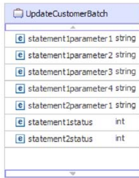
图 11. 具有两个 SQL 语句的批处理 SQL 业务对象
