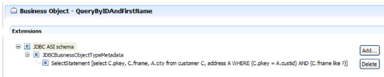
图 10. SELECT 语句保存在业务对象的特定于应用程序的信息中
