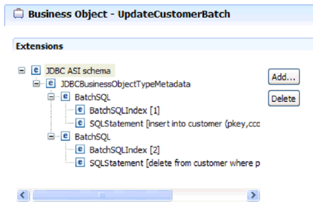
图 12. 批处理 SQL 业务对象的特定于应用程序的信息
