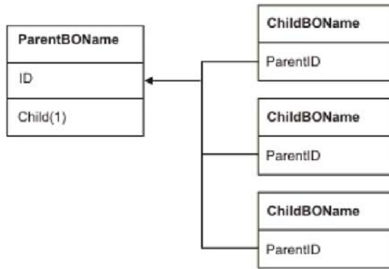
图 16. 多基数业务对象关系 ( N>1 )
