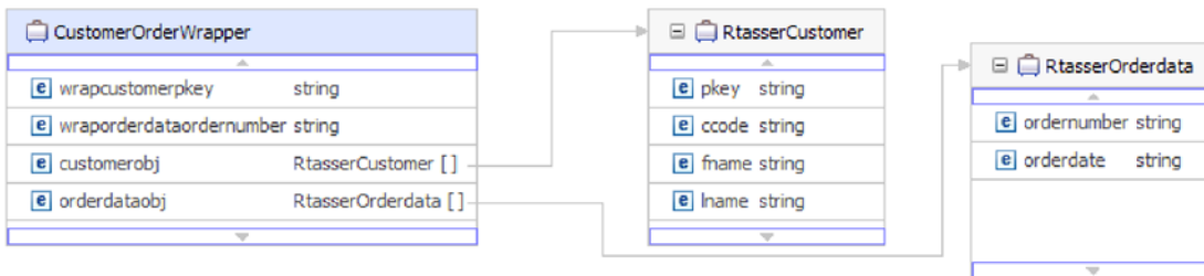
图 13. 包含两个表业务对象的包装器业务对象
