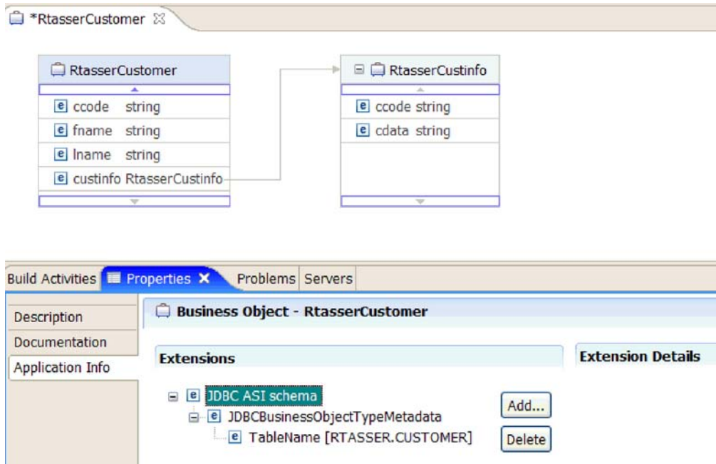
图 8. 具有一个子业务对象的表业务对象。
