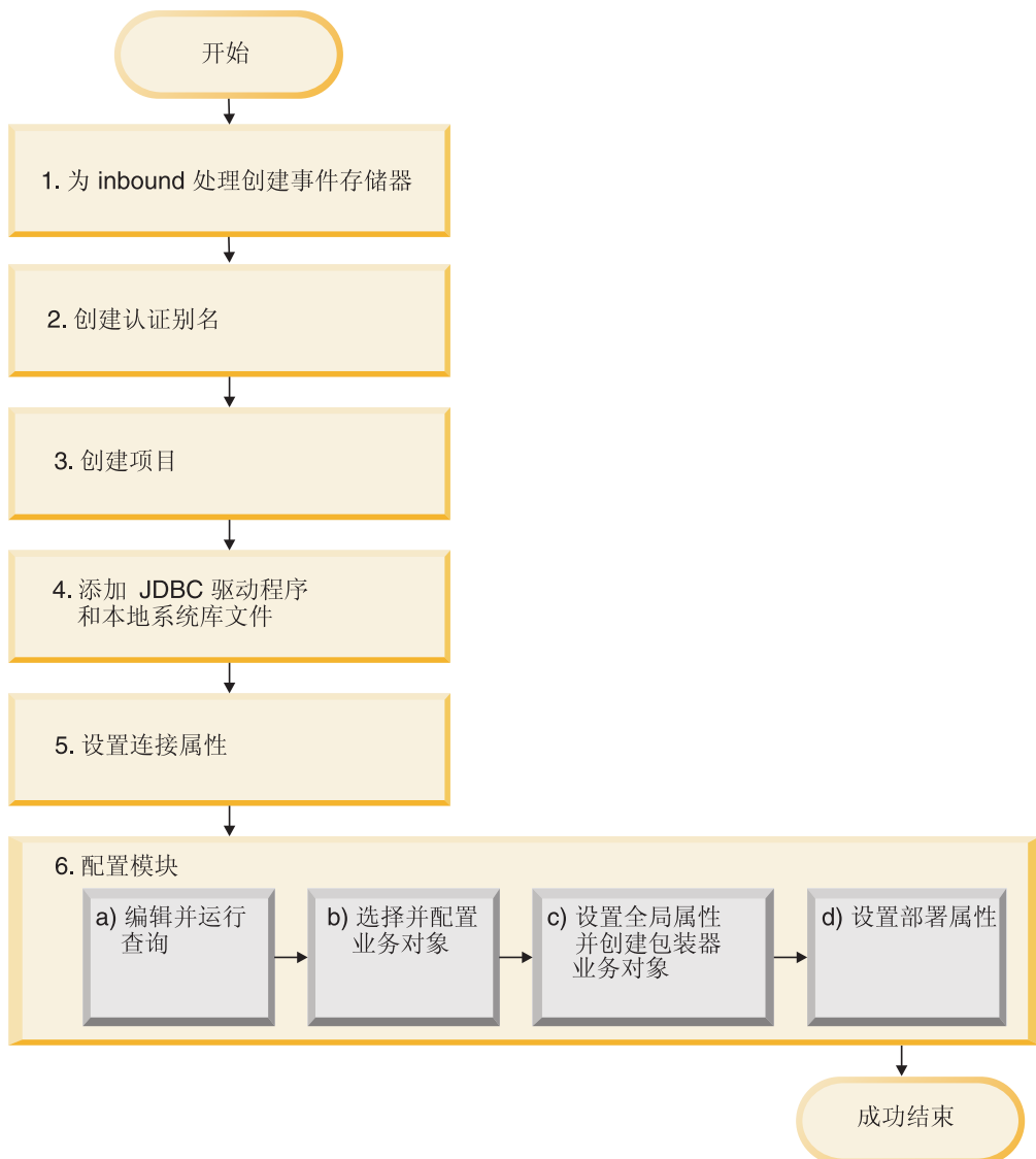
图 19. 配置模块的路线图
