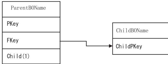
图 15. 典型单基数关系
