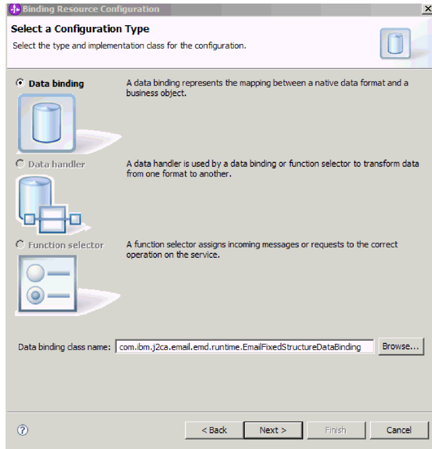
Рисунок 55. Класс связывания данных автоматически указывается в окне типа конфигурации
