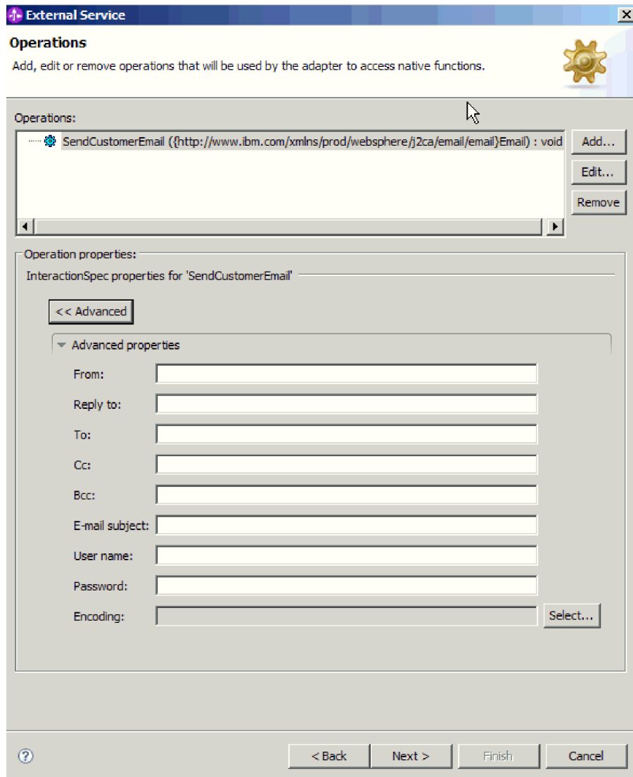
Рисунок 41. Настройка свойств спецификации взаимодействия
