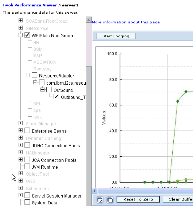
Рисунок 92. График статистики производительности адаптера
