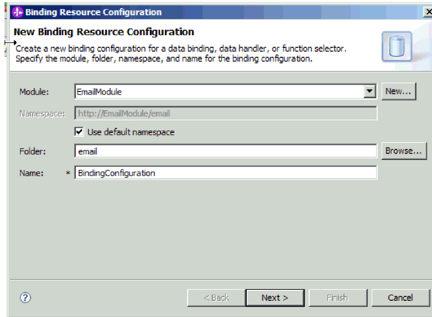
Рисунок 53. Указание имени для конфигурации связывания данных
