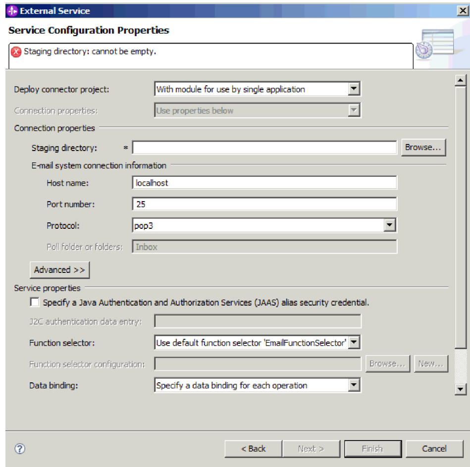
Рисунок 66. Настройка свойств входящего соединения
