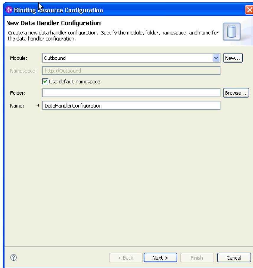
Рисунок 39. Создание обработчика данных
