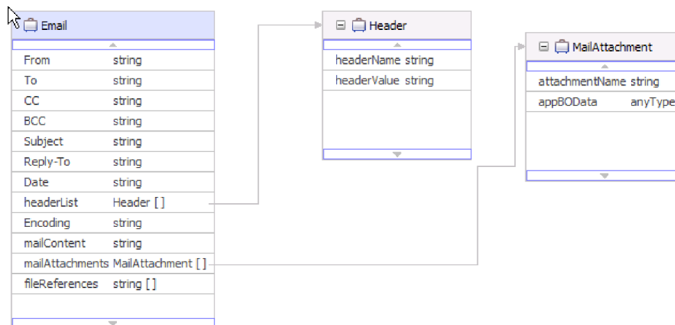
Рисунок 95. Бизнес-объект Email с дочерними объектами вложения и заголовка.
