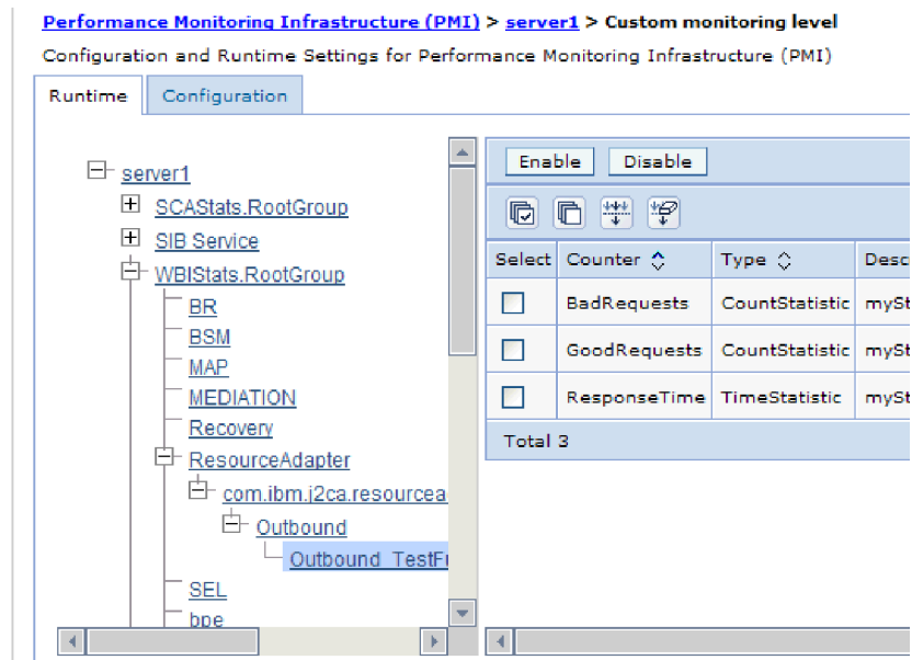
Рисунок 91. Вкладка Рабочая среда применяется для настройки PMI
