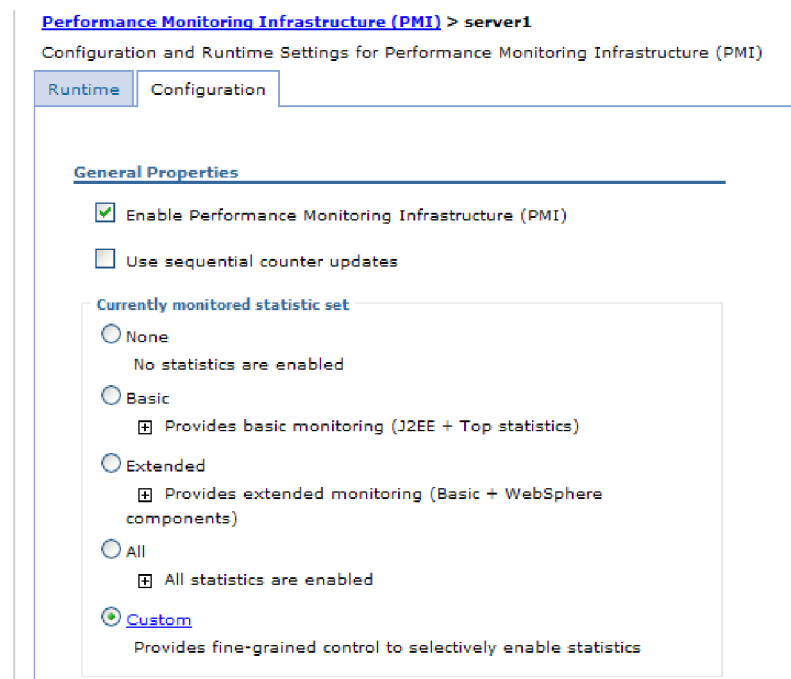
Рисунок 90. Включение системы сбора статистики
