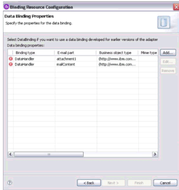
Рисунок 56. Указание свойств связывания данных
