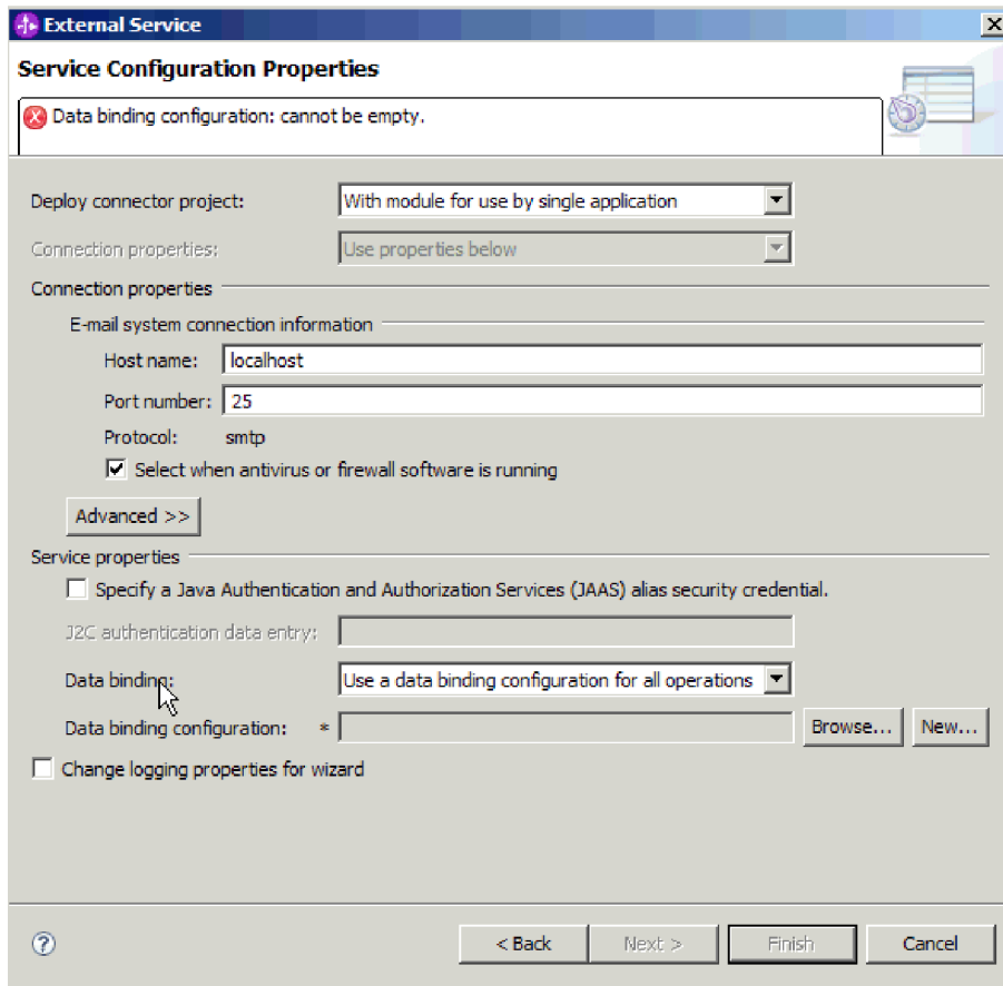
Рисунок 45. Окно Параметры конфигурации службы
