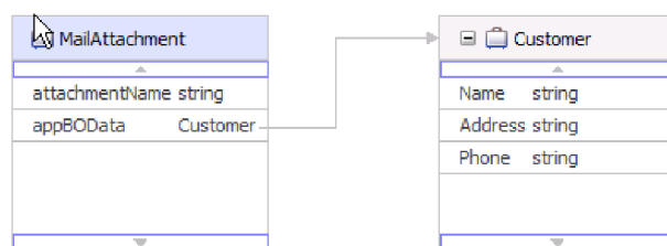
Рисунок 96. Бизнес-объект mailAttachment с дочерним объектом Customer .
