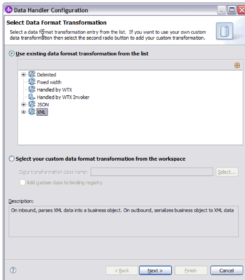
Рисунок 61. Выбор типа конфигурации обработчика данных
