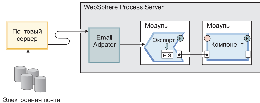
Рисунок 4. Точка экспорта в случае обработки входящих событий
