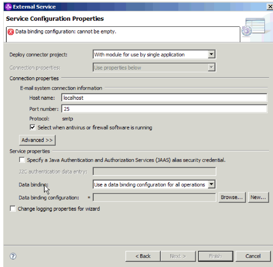
Рисунок 30. Окно Параметры конфигурации службы
