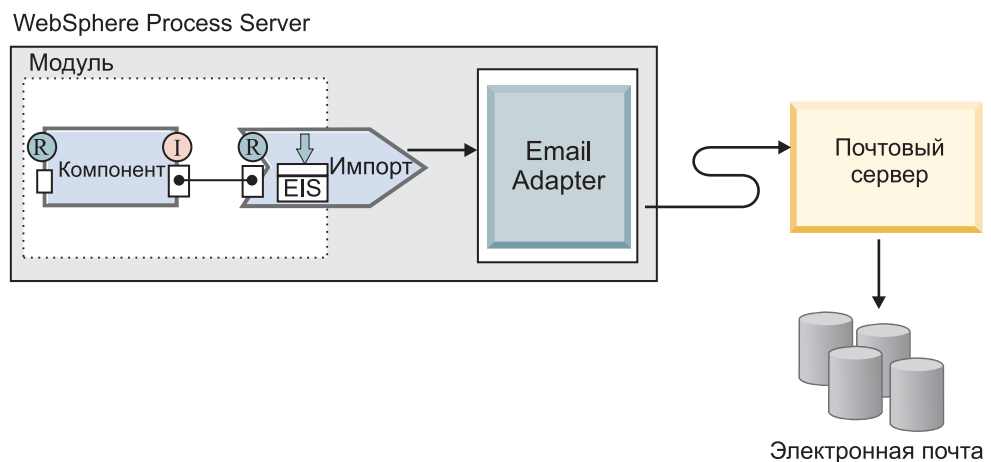
Рисунок 2. Исходящие соединение с указанием точки импорта
