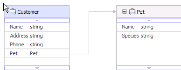
Рисунок 6. Бизнес-объект Customer с дочерним бизнес-объектом Pet
