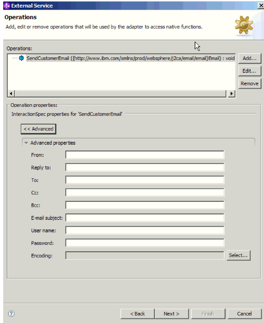
Рисунок 62. Настройка свойств спецификации взаимодействия
