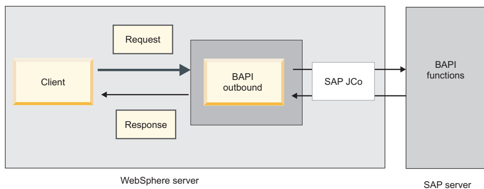
Rysunek 5. Sposób, w jaki adapter łączy aplikację wywołującą z aplikacją SAP
