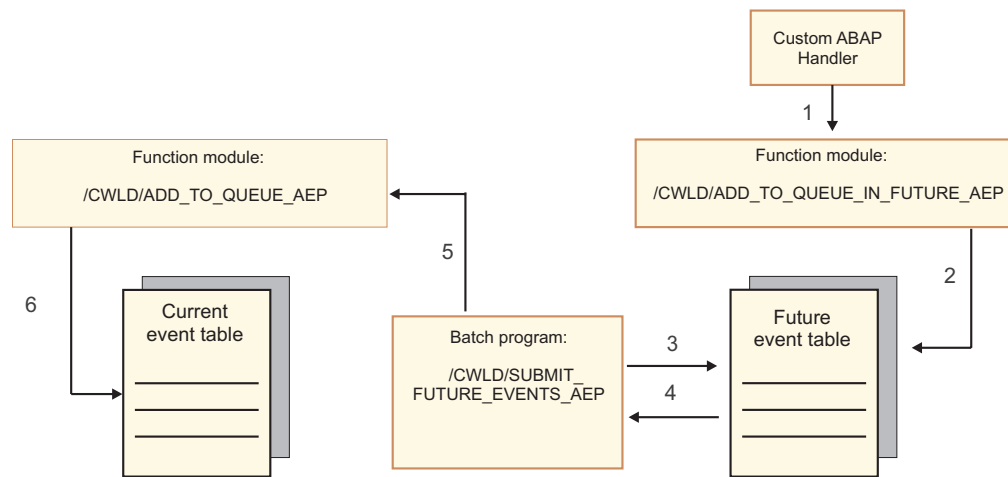
Rysunek 46. Sposób dodawania zdarzenia do tabeli przyszłych zdarzeń, pobierania go z tej tabeli i dodawania do tabeli bieżących zdarzeń
