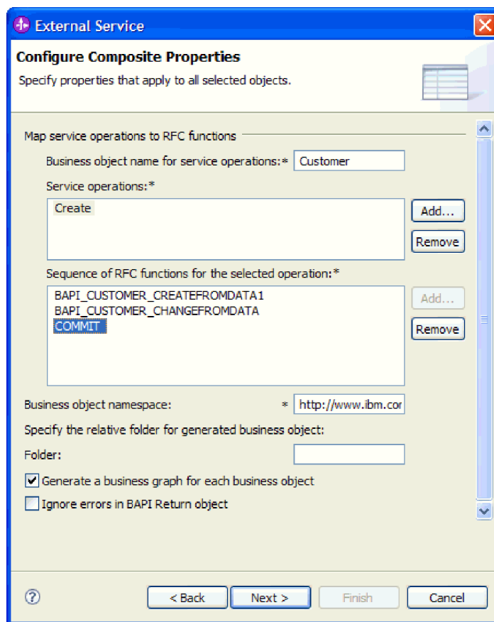
Rysunek 71. Okno Konfiguracja właściwości złożonych po wybraniu funkcji BAPI oraz operacji COMMIT
