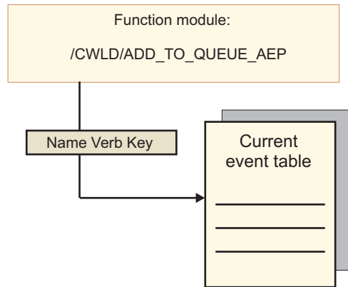
Rysunek 45. Dodawanie wiersza danych do tabeli bieżących zdarzeń przez moduł funkcji
