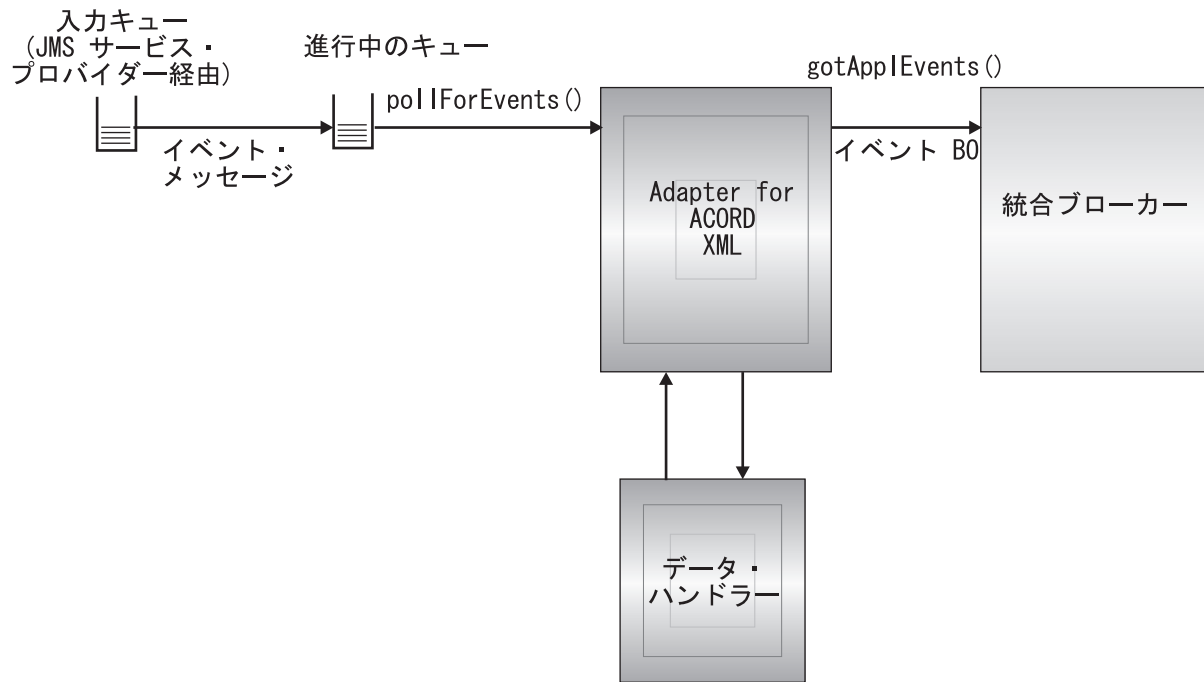
図2. アプリケーションとコネクタ間の通信方式: イベント・デリバリー
