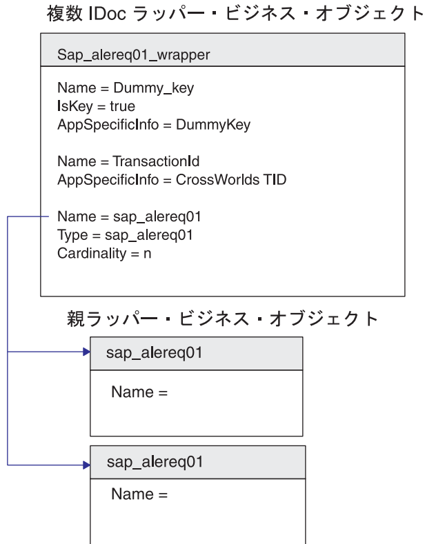
図 21. 子ビジネス・オブジェクトを含んでいるラッパー・ビジネス・オブジェクト
