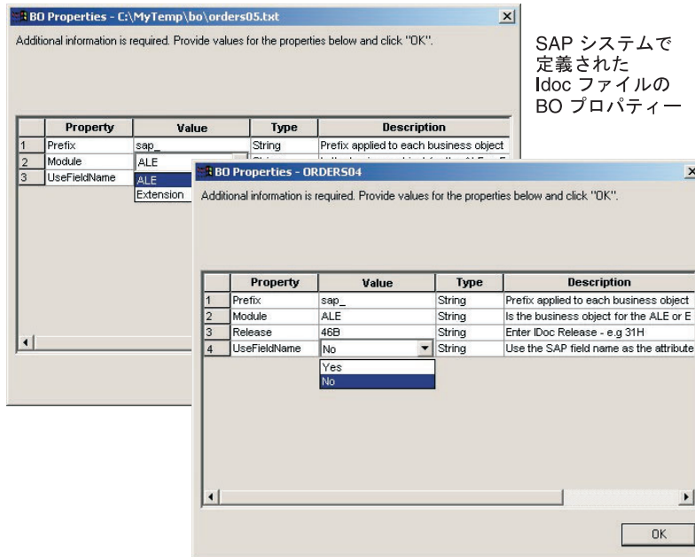
図 45. IDoc タイプ・ビジネス・オブジェクトの追加情報の指定
