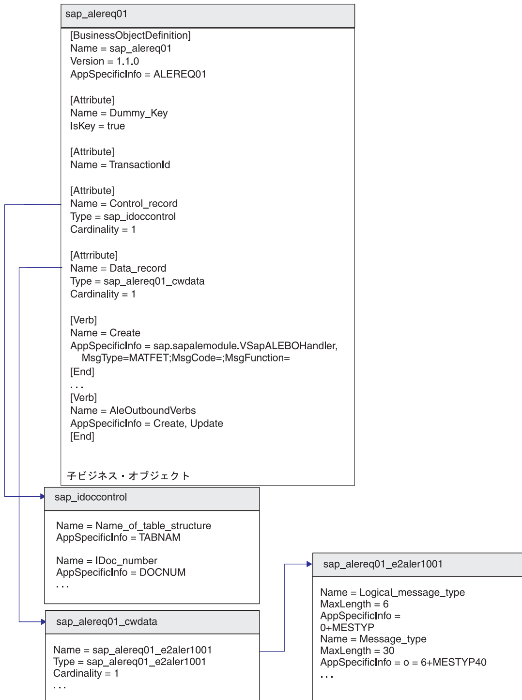
図 19. SAP の WebSphere ビジネス・オブジェクトと IDoc の関係
