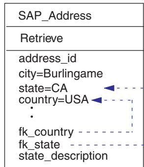
図 34. 例: 現在のビジネス・オブジェクトが外部キーを格納している場合
