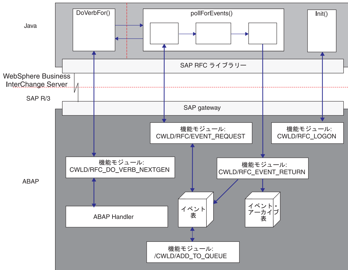
図 5. ABAP Extension Module のアーキテクチャー
