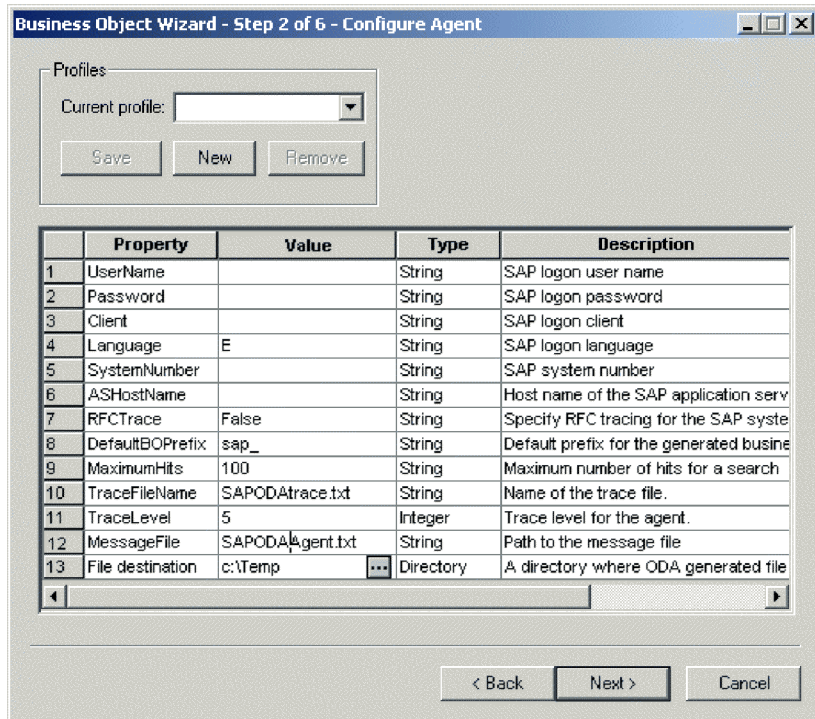
図 40. エージェント・プロパティの構成
