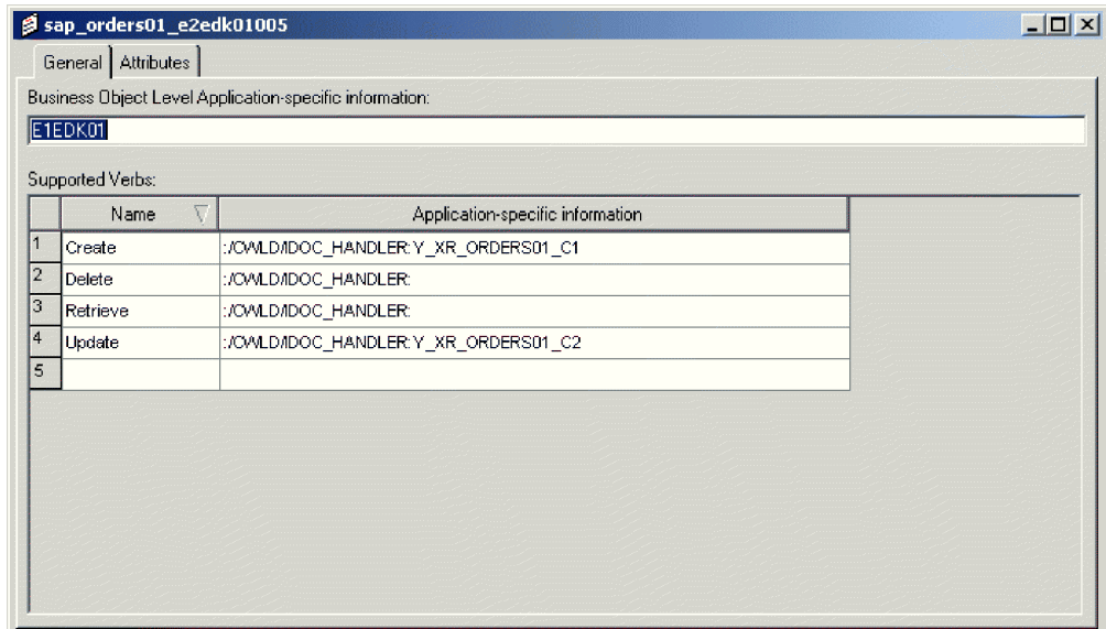
図 47. Business Object Designer での ABAP Handler の指定
