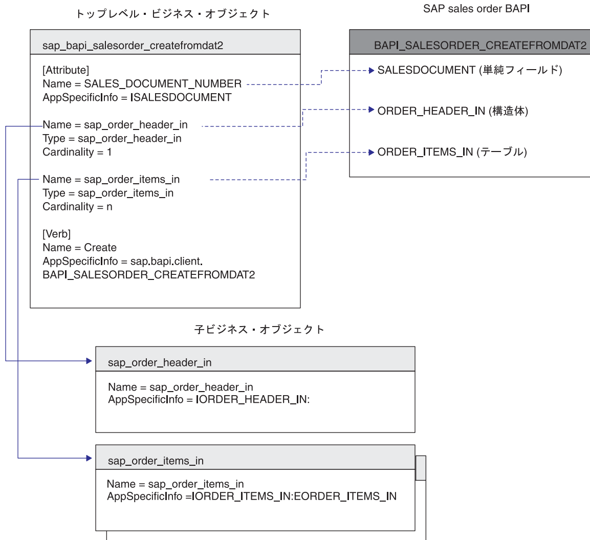
図 24. ビジネス・オブジェクトと BAPI とのマッピング
