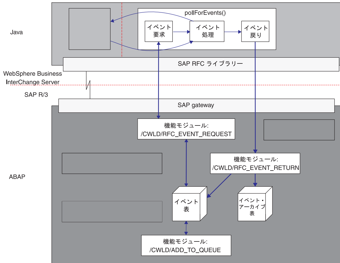
図 8. イベント通知プロセス
