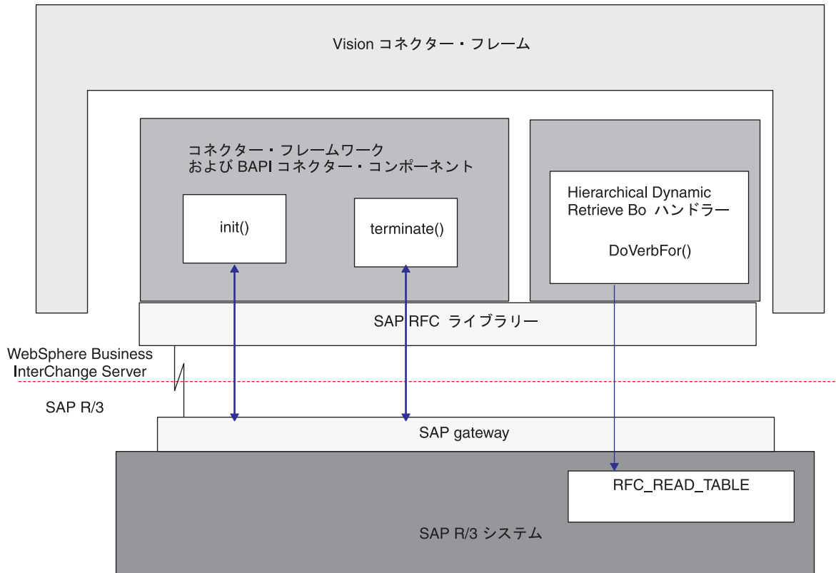
図 30. Hierarchical Dynamic Retrieve Module のアーキテクチャー
