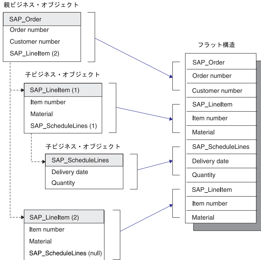
図 13. ビジネス・オブジェクトからフラットな構造への変換
