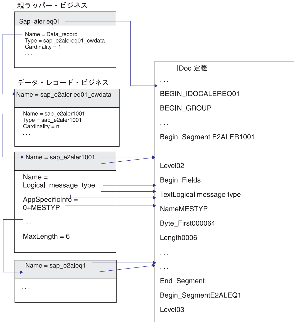
図 20. データ・レコード・ビジネス・オブジェクトと IDoc 定義フィールドとの関係
