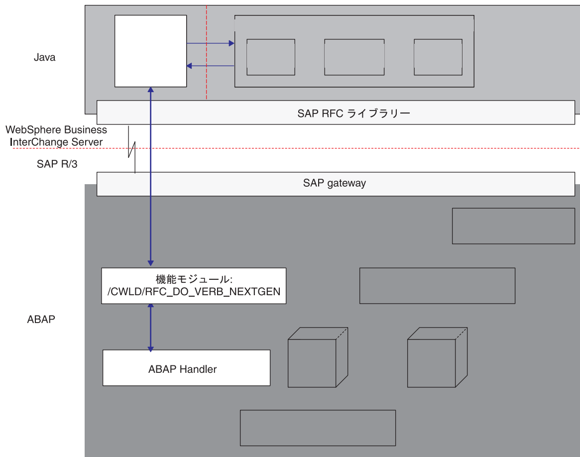
図 6. doVerbFor() のビジネス・オブジェクト処理
