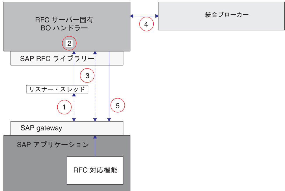
図 27. ビジネス・オブジェクトの処理
