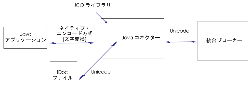
図 4. エージェント・プロパティの構成
