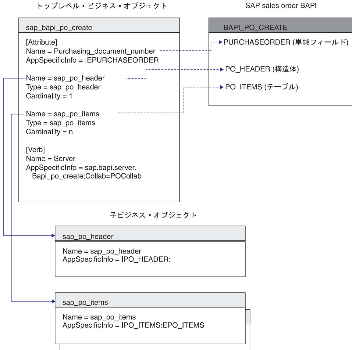
図 28. ビジネス・オブジェクトと BAPI とのマッピング
