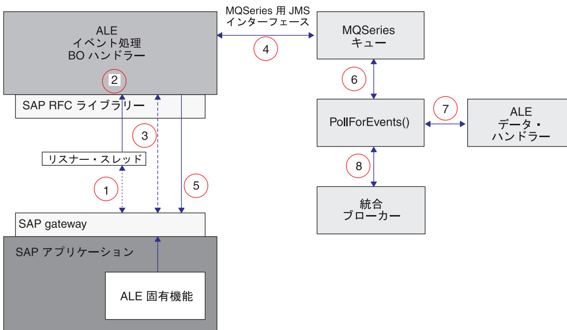
図 18. ビジネス・オブジェクト・イベント処理
