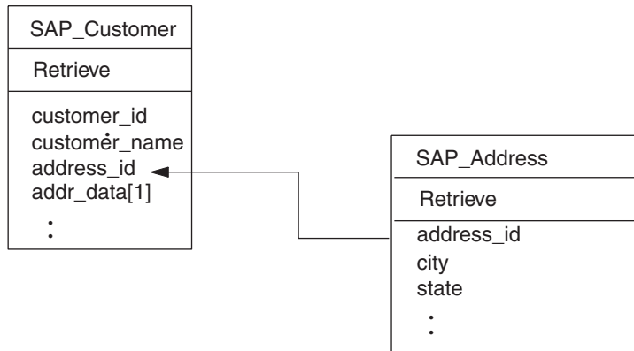
図 31. カスタマーとアドレスの関係の例
