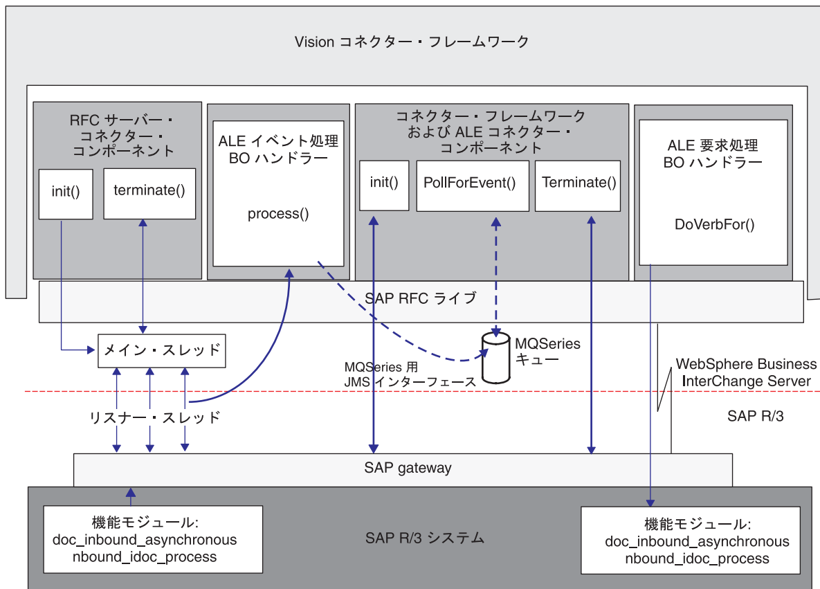
図 17. ALE Module のアーキテクチャー
