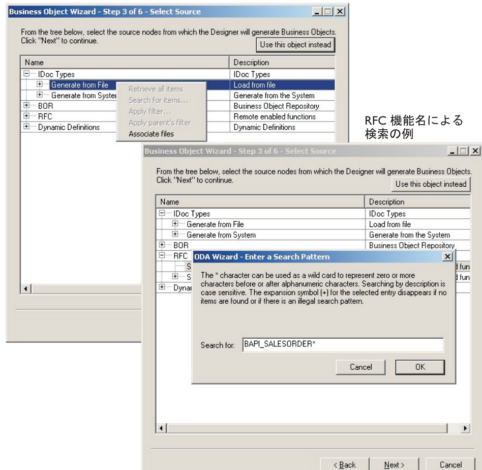
図 42. ファイルの関連付けと検索基準の入力
