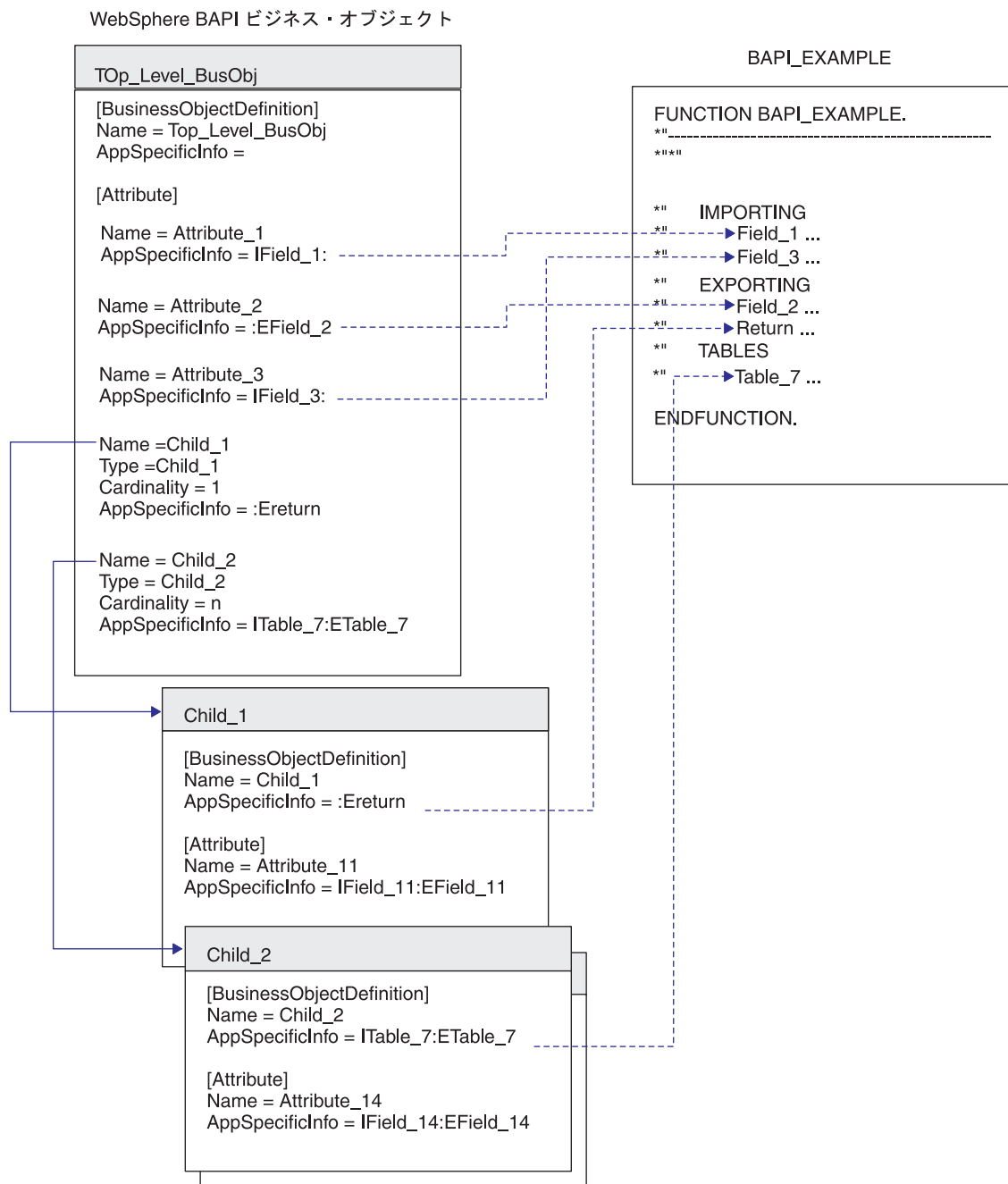
図 25. ビジネス・オブジェクトとサンプル BAPI との対応
