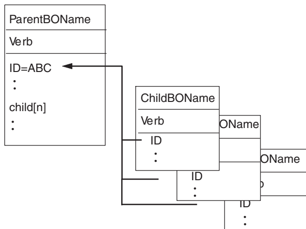
図 32. 複数カーディナリティーのビジネス・オブジェクト関係
