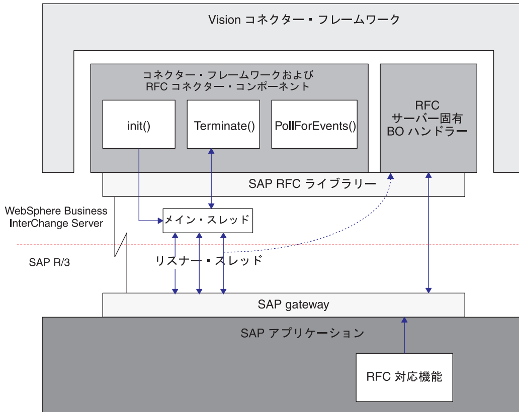
図 26. RFC Server Module のアーキテクチャ
