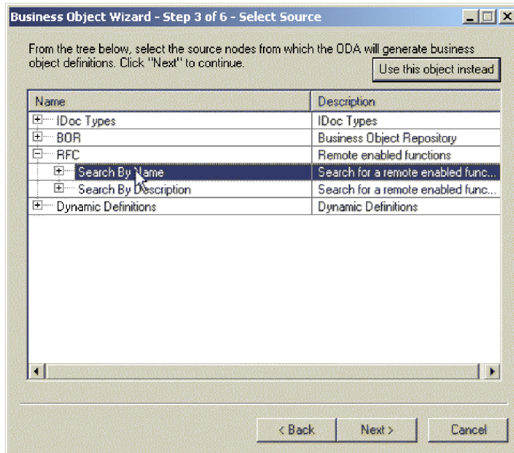
図 36. ビジネス・オブジェクト・ウィザード—ソースの選択
