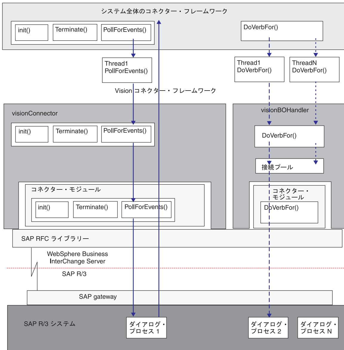
図3. Connector for SAP のマルチスレッド化アーキテクチャ
