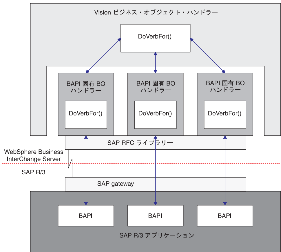
図 23. BAPI Module ビジネス・オブジェクト処理
