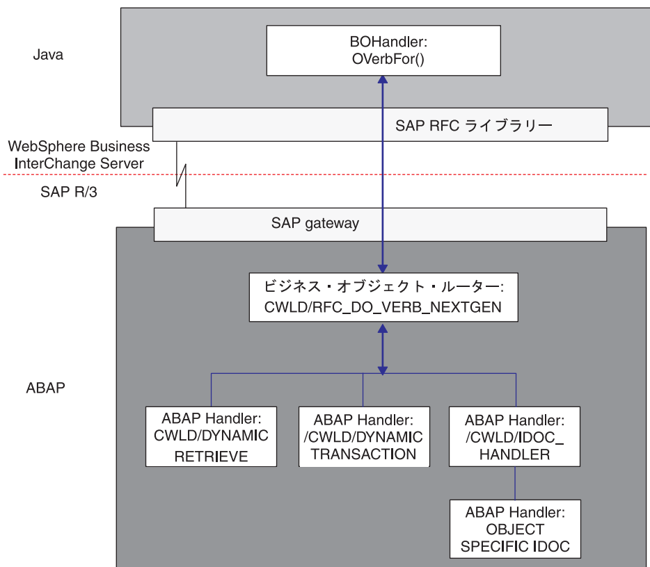
図7. Adapter 提供のビジネス・オブジェクト処理コンポーネント
