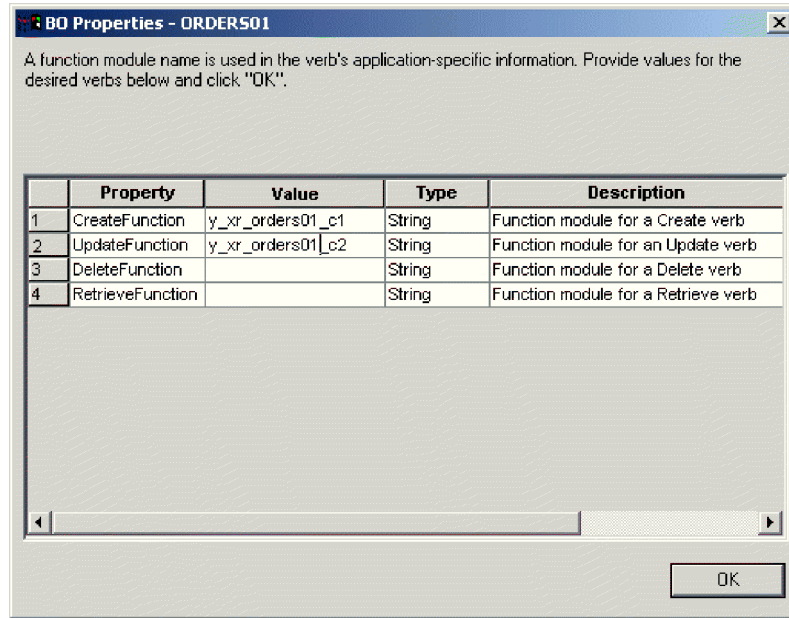
図 46. ABAP Handler に対する機能モジュールの指定
