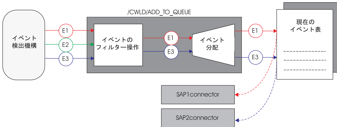
図 11. 機能モジュール /CWLD/ADD_TO_QUEUE によるイベント優先順位の設定
