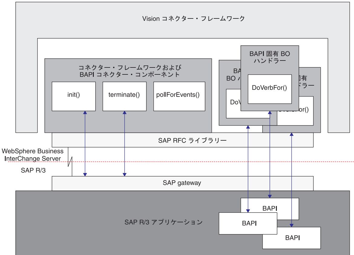
図 22. BAPI Module のアーキテクチャー
