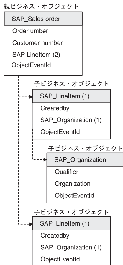
図 15. 階層型ビジネス・オブジェクト SAP sales order (IDoc)
