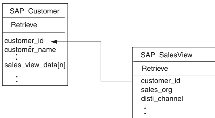
図 33. カスタマーと販売ビュー関係の例
