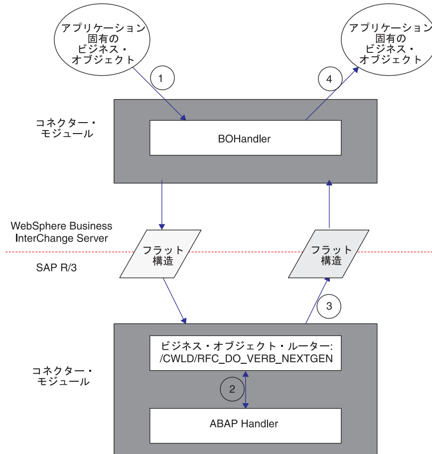
図 12. ビジネス・オブジェクトの処理
