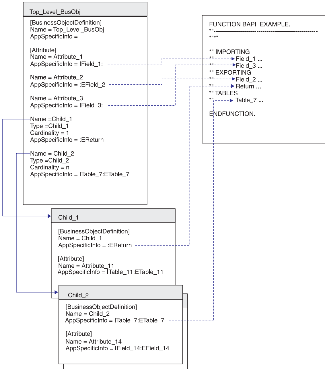
図 29. ビジネス・オブジェクトと BAPI 例とのマッピング
