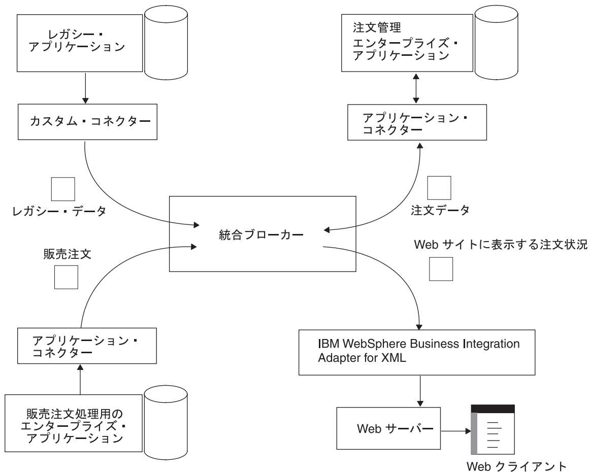
図 2. WebSphere Business Integration システム
