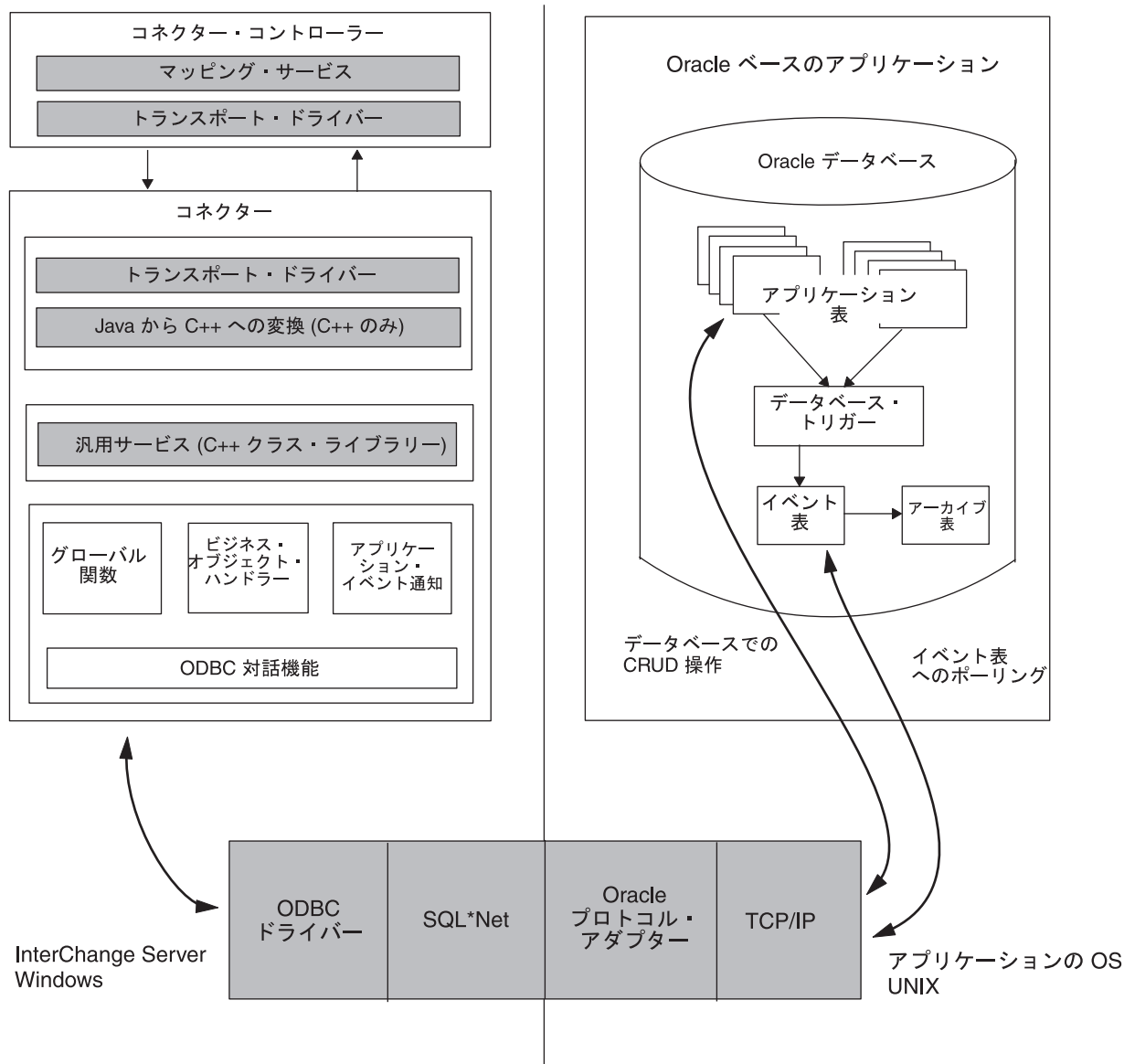
図 22. ODBC ベースのコネクタ・アーキテクチャのサンプル
