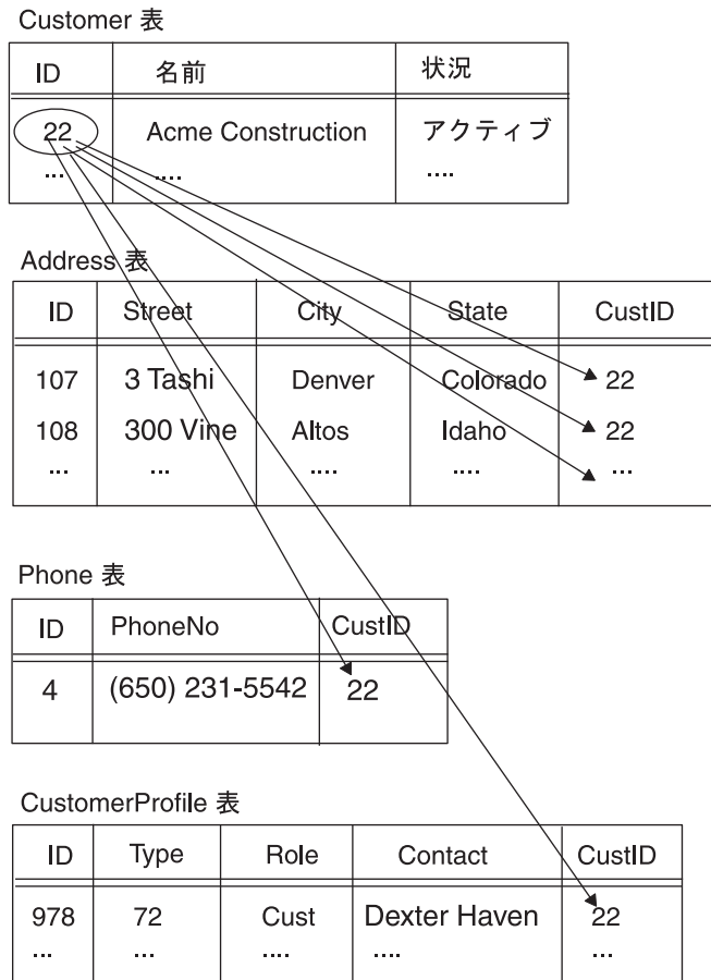
図 36. Update 要求後の Customer エンティティ
