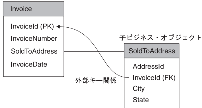
図 44. 単一カーディナリティーを持つビジネス・オブジェクト
