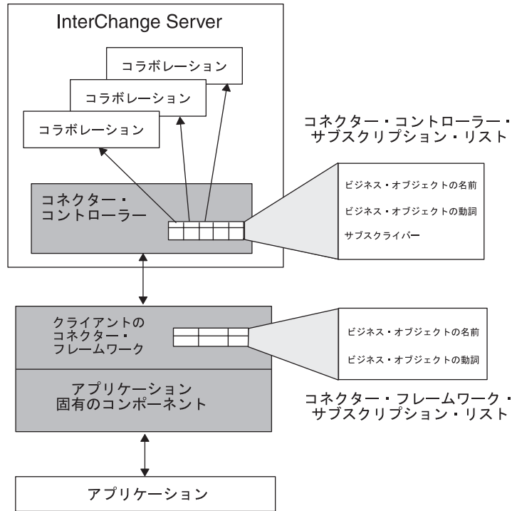
図7. サブスクリプション処理
