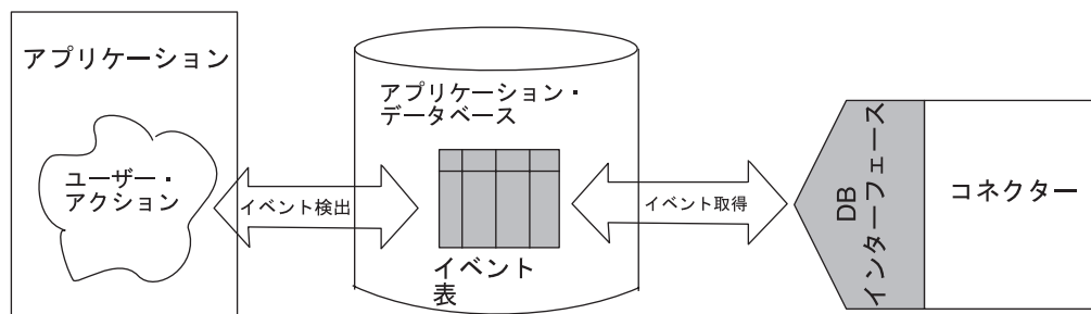
図48. イベント・ストアとしてのイベント表
