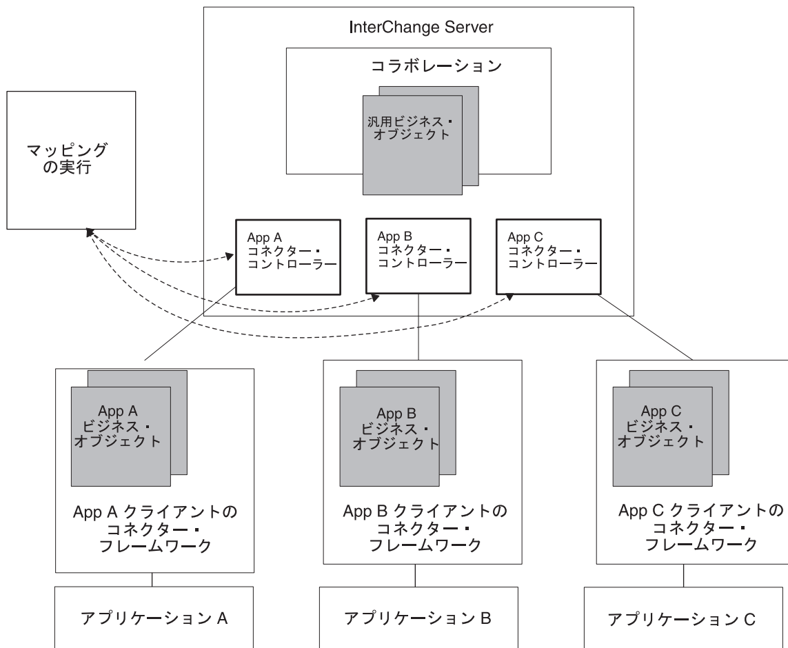
図 6. InterChange Server System でのマッピング
