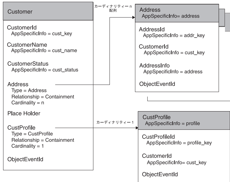
図 46. 階層型ビジネス・オブジェクト定義の例
