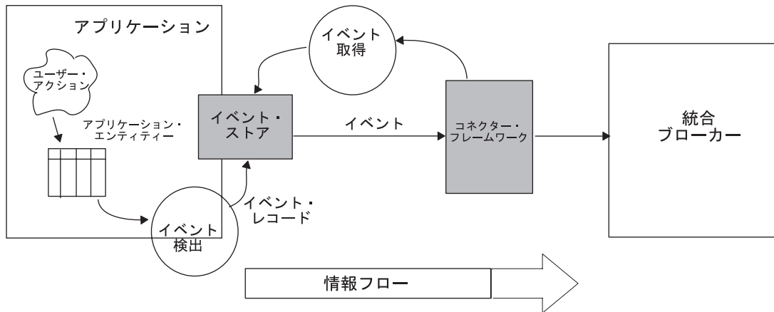
図 11. イベントの検出および取得
