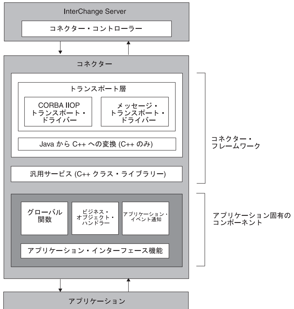
図 8. InterChange Server との通信に対応したコネクタ・アーキテクチャ
