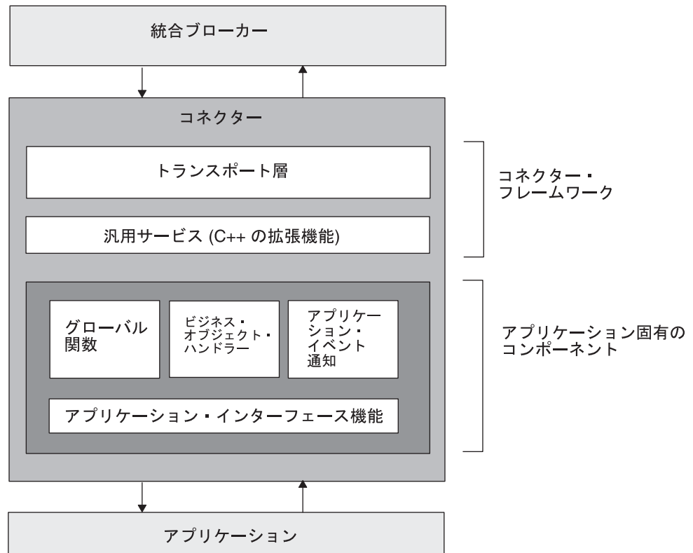
図3. Java コネクタのコンポーネント
