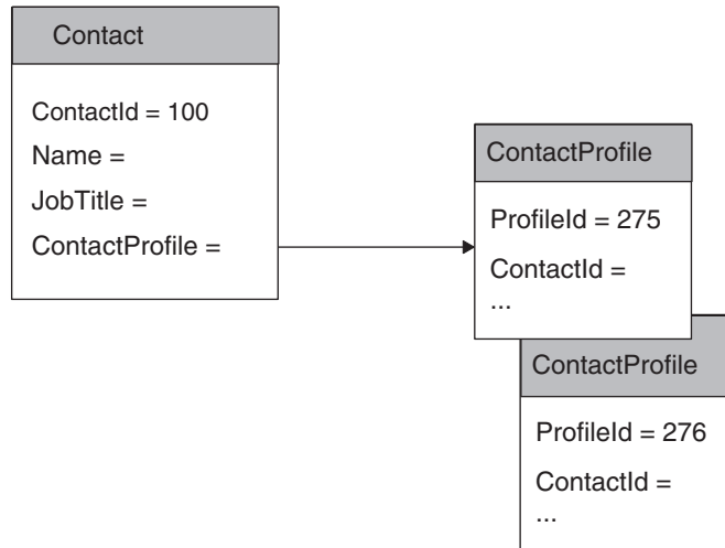
図 29. Retrieve 要求用のビジネス・オブジェクト例
