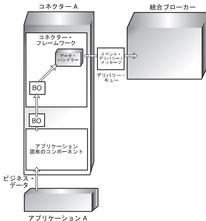
図 4. WebSphere Message Broker を使用した上位のコネクタ・アーキテクチャ
