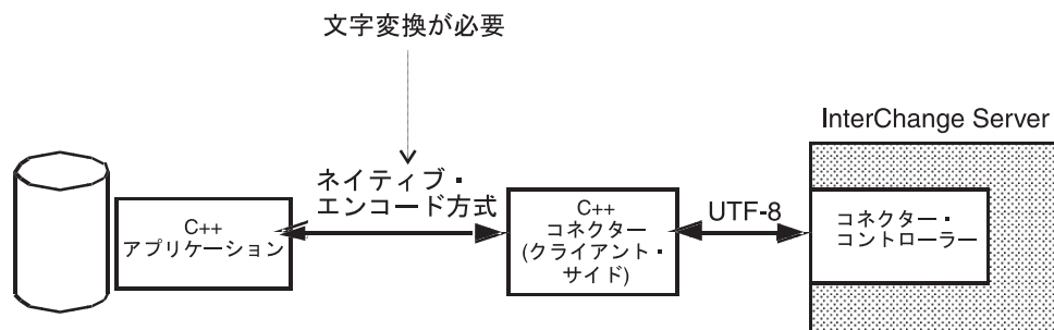
図 23. C++ コネクタでの文字エンコード
