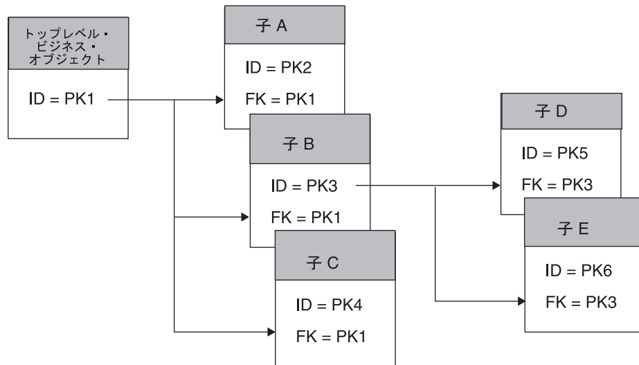
図 28. 親子関係の作成
