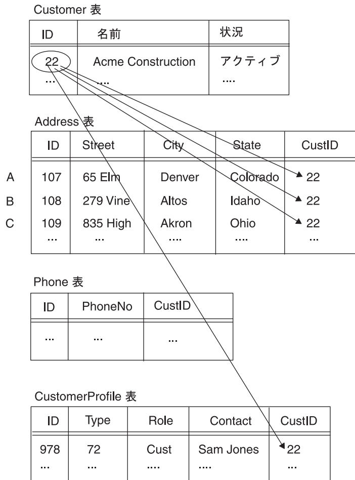
図 34. Update 要求前の Customer エンティティ
