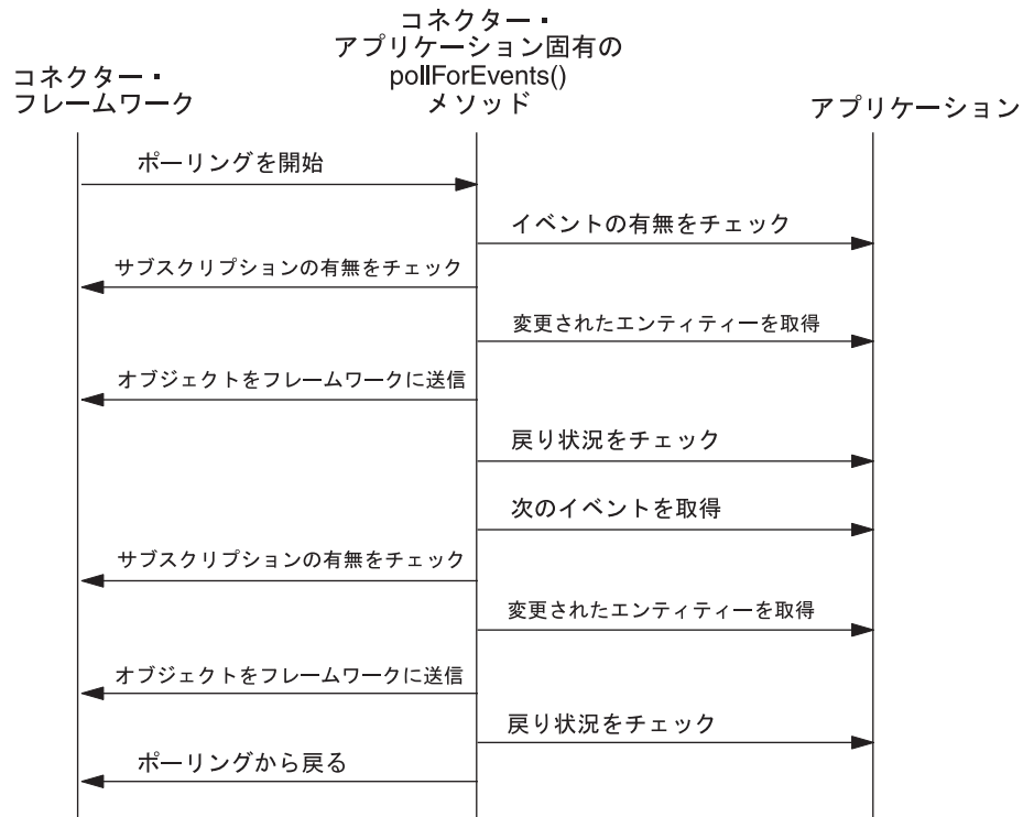
図 54. pollForEvents() メソッドの基本的な振る舞い
