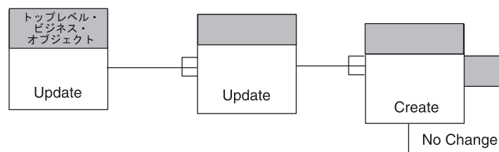
図 38. 物理削除コネクタの要求ビジネス・オブジェクトの更新
