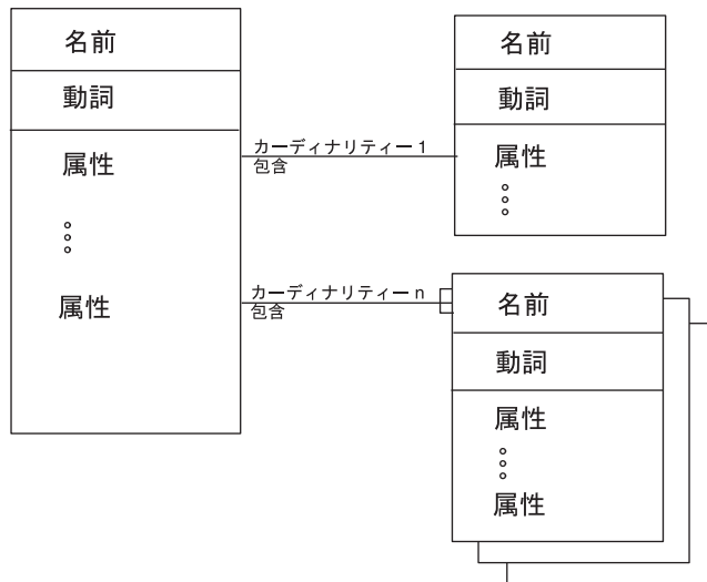
図 43. 階層型ビジネス・オブジェクト
