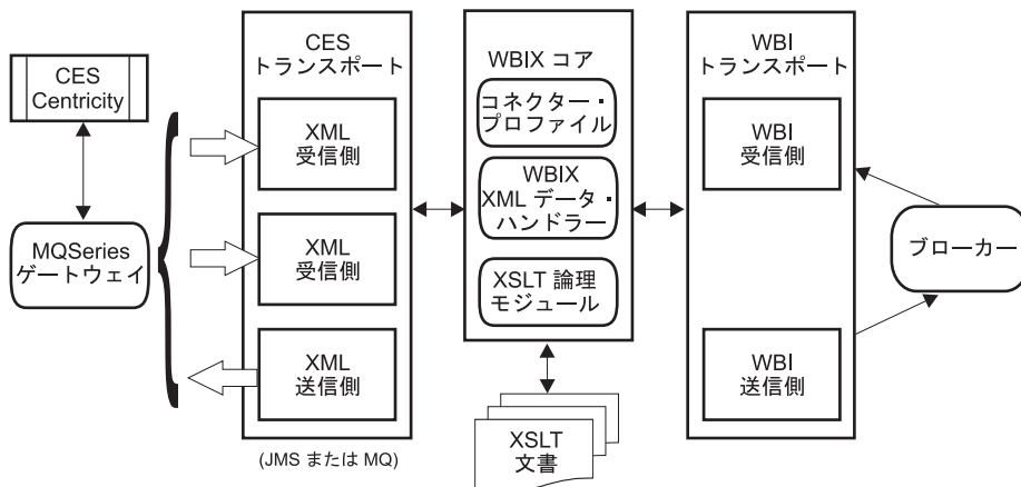
図 1. Adapter for CES Centricity Gateway のアーキテクチャーの詳細
