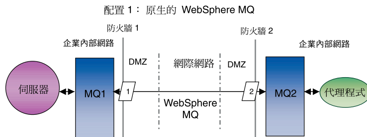
圖 2. 原生的 WebSphere MQ 配置
