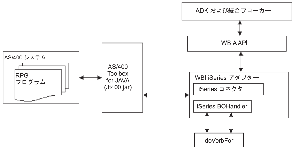
図2. Adapter for iSeries を使用した場合の接続図
