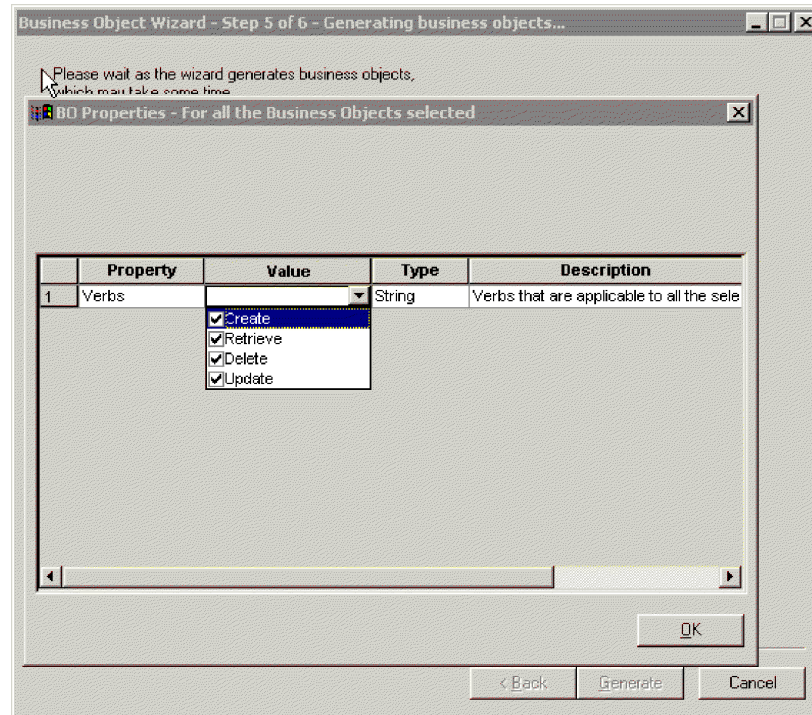
図 49. 追加情報の入力 - 動詞
