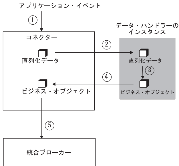
図3. コネクタのコンテキストでのストリングからビジネス・オブジェクトへの変換
