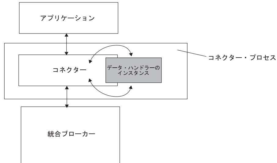
図 1. コネクターのコンテキストでのデータ・ハンドラー
