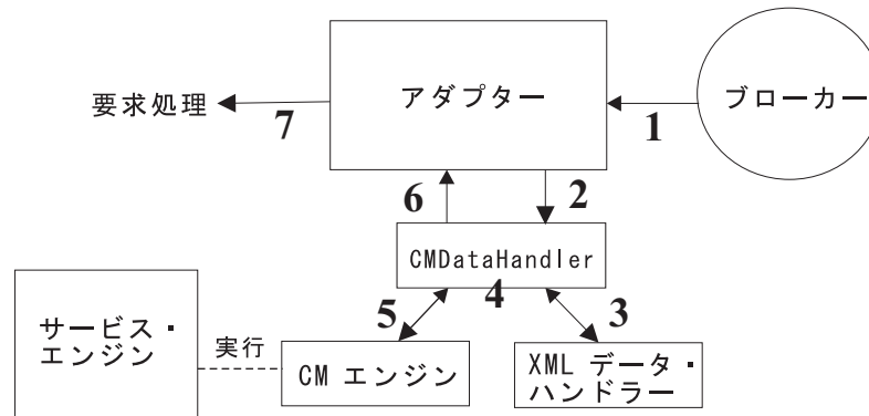
図 37. Complex Data データ・ハンドラーによる要求処理
