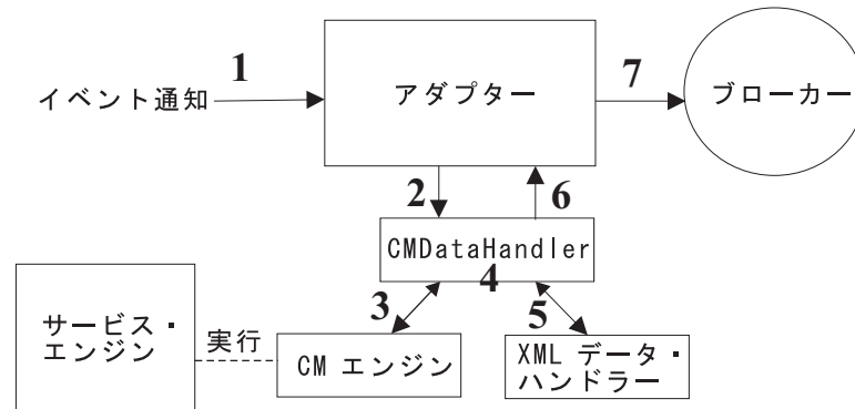
図 38. Complex Data データ・ハンドラーによるイベント通知
