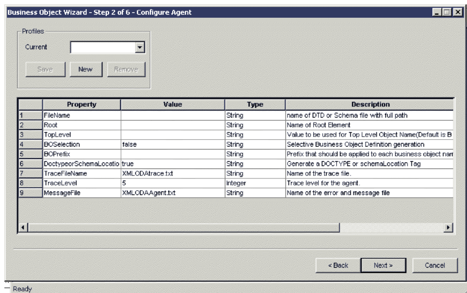
図 45. ODA 構成プロパティの指定
