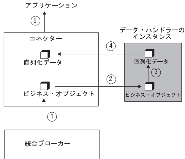
図2. コネクターのコンテキストでのビジネス・オブジェクトからストリングへの変換
