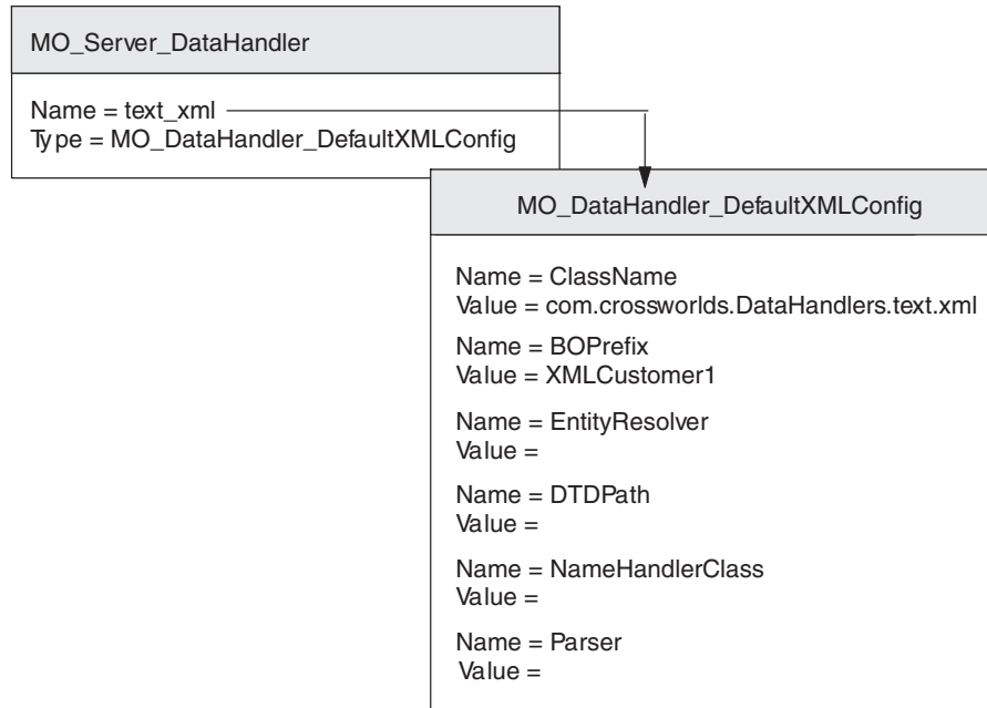
図9. MO_Server_DataHandler メタオブジェクト
