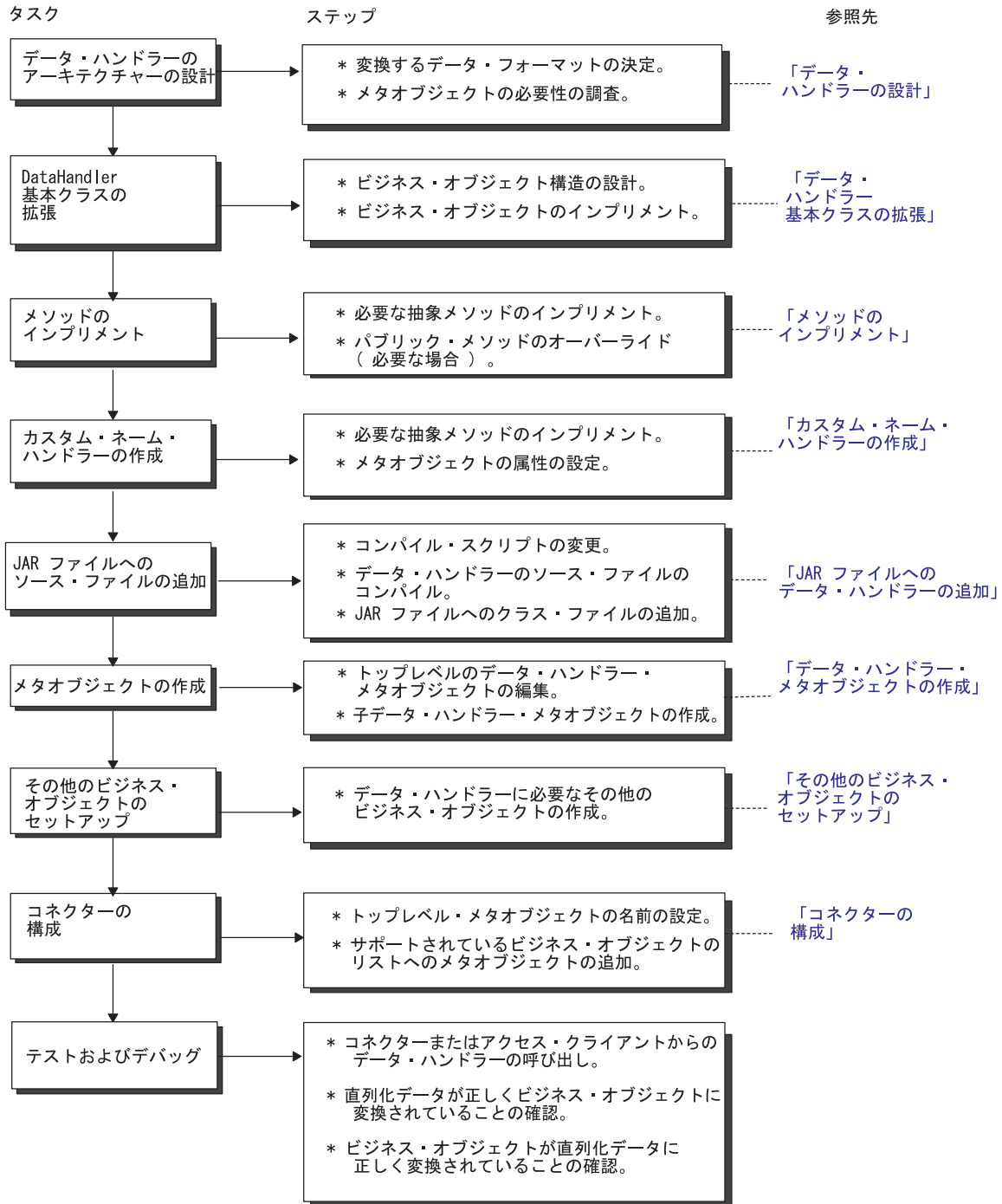
図 39. データ・ハンドラー開発過程の概要
