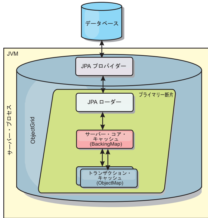
図 29. JPA ロードアーキテクチャー
