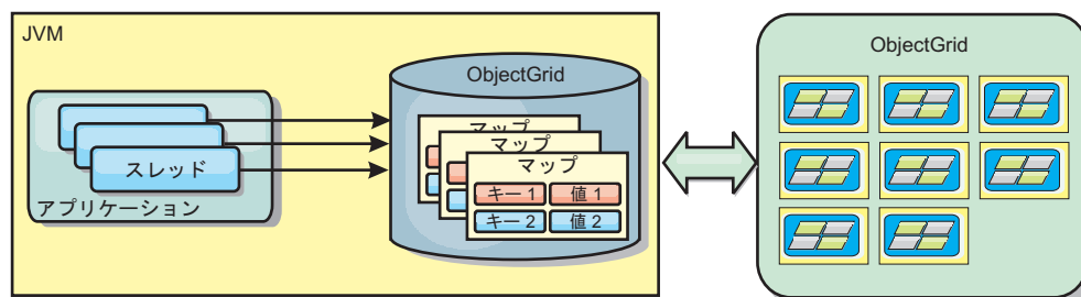
図10. ニア・キャッシュ
