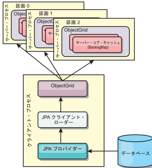
図 30. ObjectGrid へのロードに JPA 実装を使用するクライアント・ローダー
