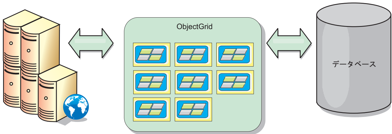
図 11. データベース・バッファーとしての ObjectGrid
