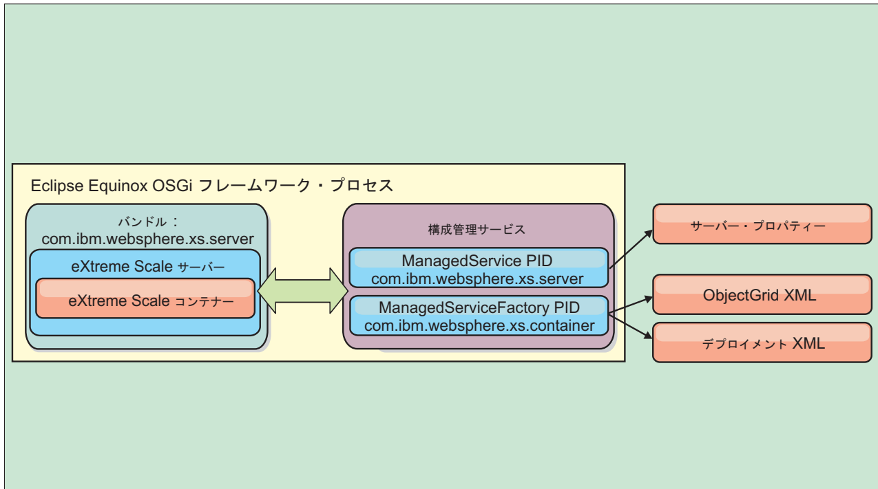
図 4. OSGi バンドルの外部で構成およびメタデータを指定するための Eclipse Equinox プロセス
