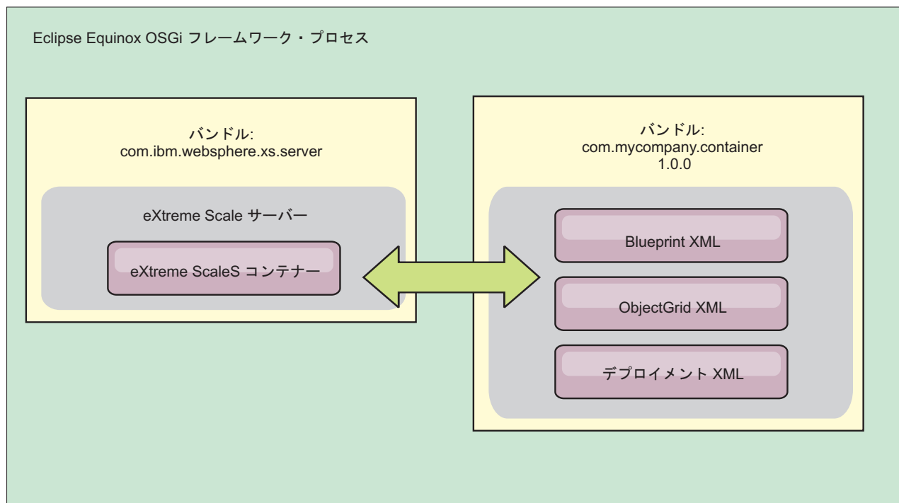
図 3. OSGi バンドルにすべての構成およびメタデータを含めるための Eclipse Equinox プロセス
