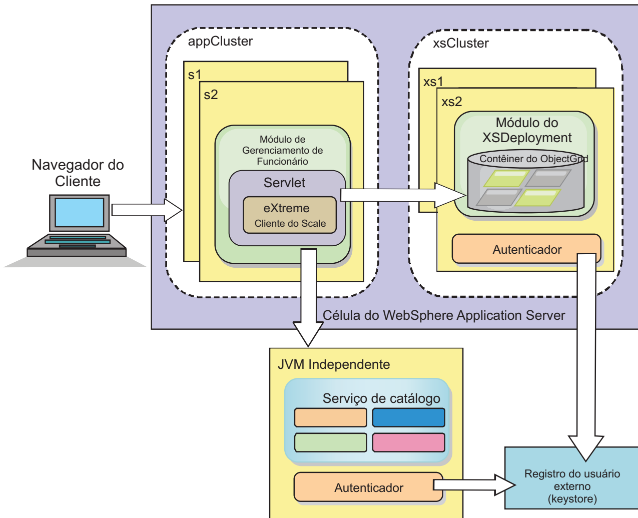
Figura 20. Topologia do Tutorial
