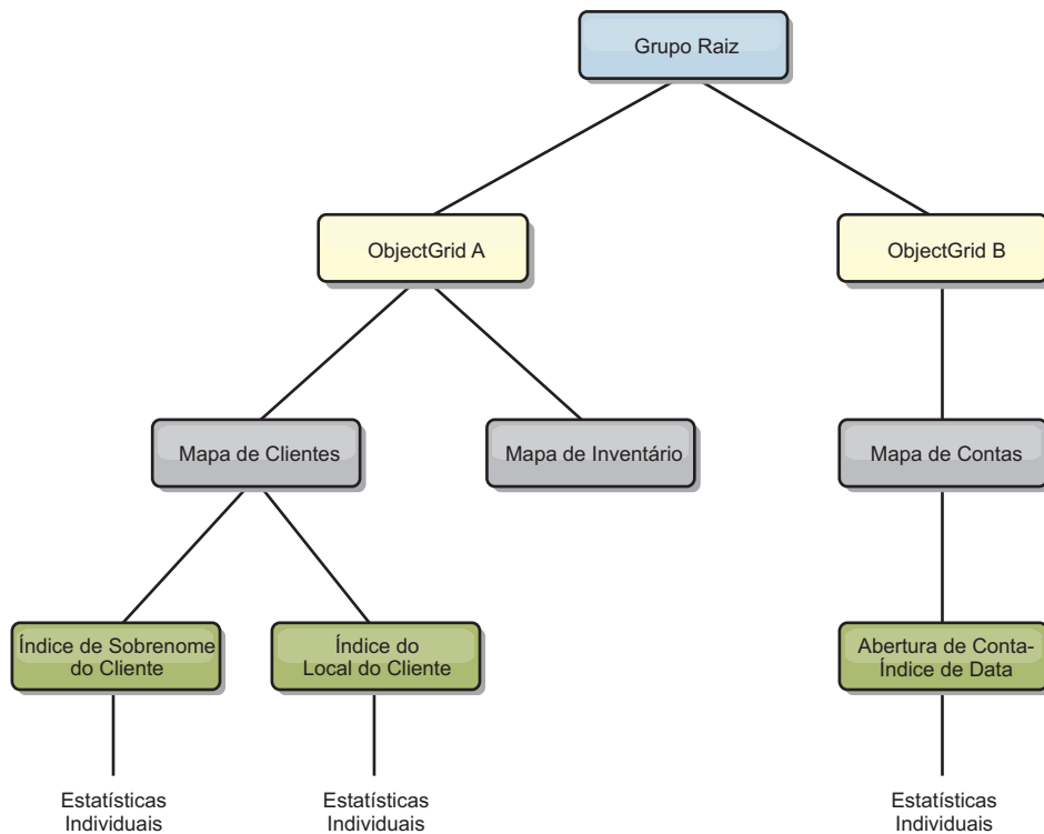
Figura 63. Exemplo da Estrutura do Módulo hashIndexModule
