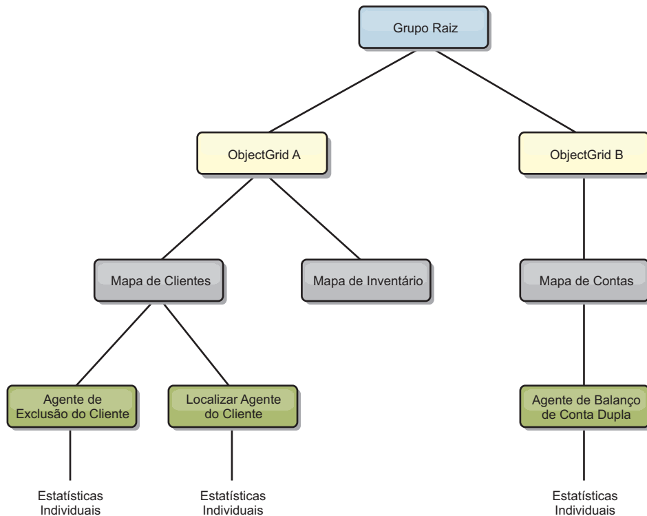
Figura 65. Exemplo da Estrutura agentManagerModule
