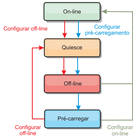
Figura 50. Estados de Disponibilidade de uma Instância do ObjectGrid
