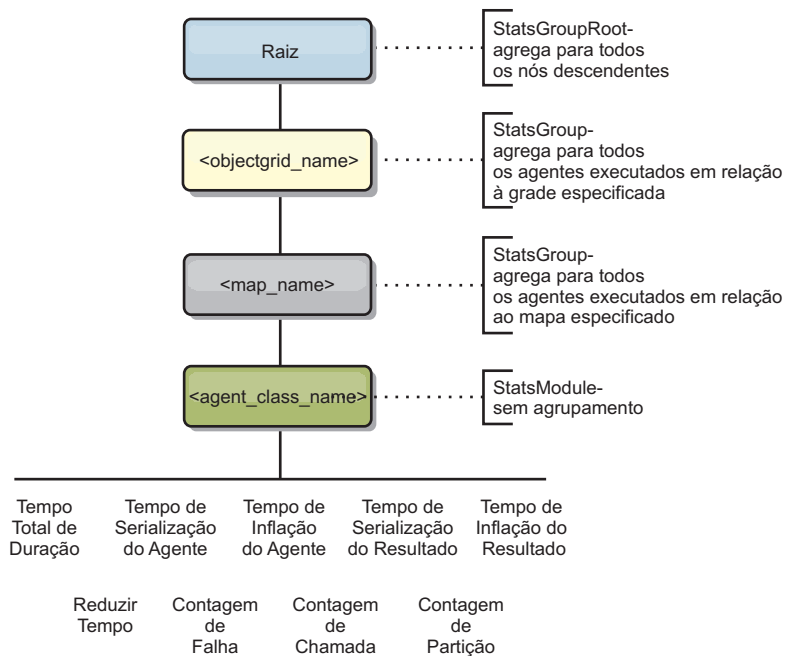
Figura 64. Estrutura agentManagerModule
