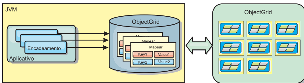
Figura 6. Cache Local
