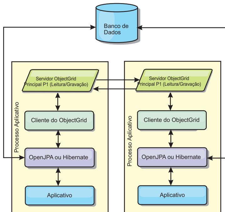
Figura 40. Topologia de Intradomínio do JPA
