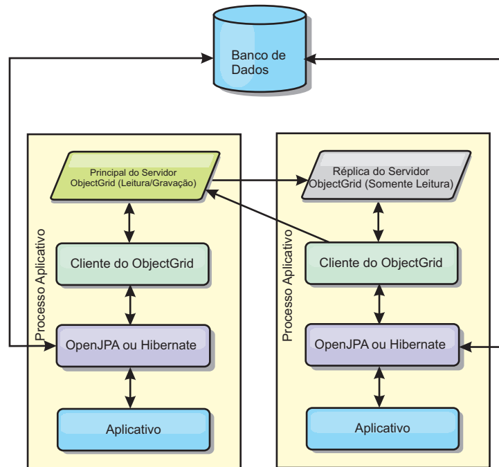
Figura 41. Topologia Integrado do JPA
