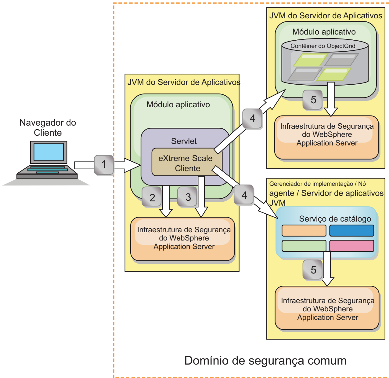
Figura 68. Fluxo de Autenticação para Servidores Dentro do Mesmo Domínio de Segurança
