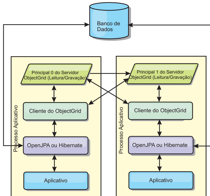
Figura 42. Topologia Particionada Integrada do JPA
