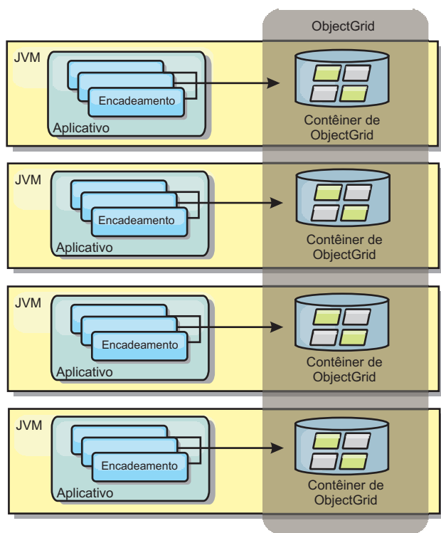
Figura 4. Cache Integrado
