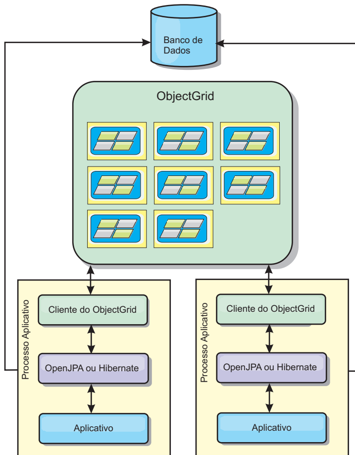
Figura 43. Topologia Remota do JPA
