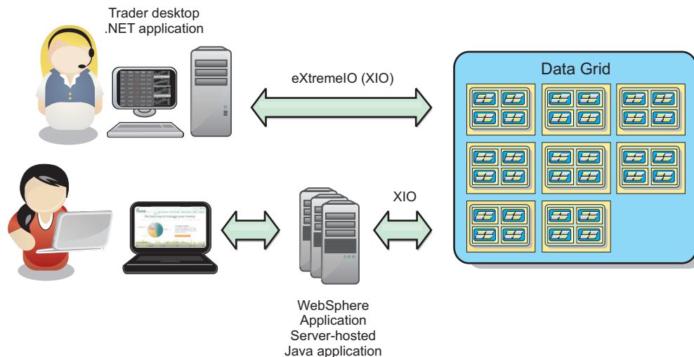
Figura 10. Visão Geral Resumida da Grade de Dados Corporativos
