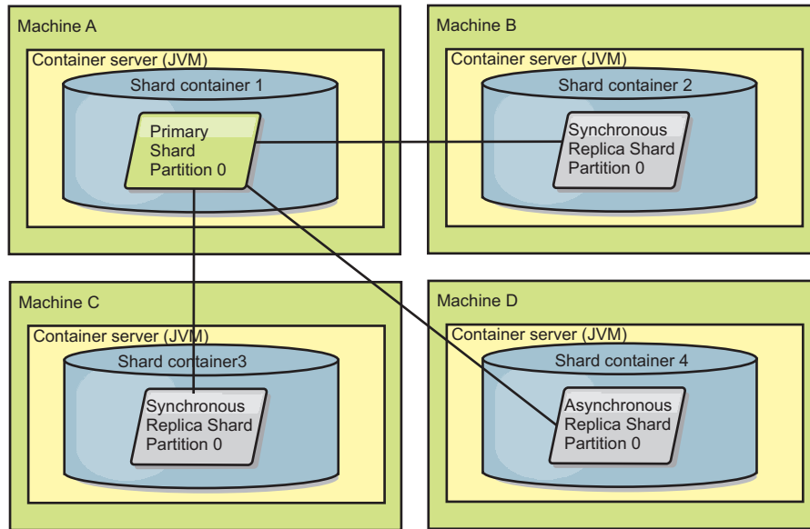
Figura 35. Posicionamento de exemplo de um conjunto de mapas do ObjectGrid para a partição partition0. A política de implementação tem um valor de minSyncReplicas de 1, um valor de maxSyncReplicas de 2, e um valor de maxAsyncReplicas de 1.
