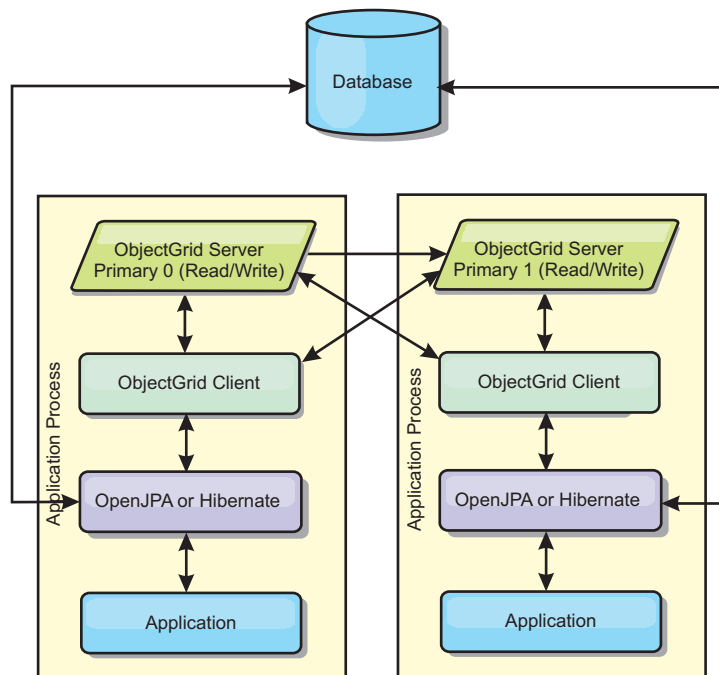
Figura 16. Topologia Particionada Integrada do JPA
