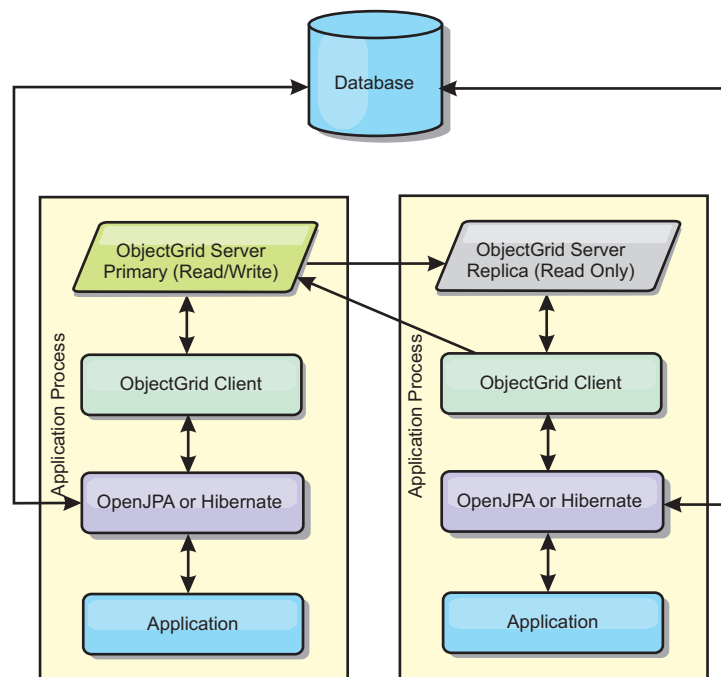
Figura 15. Topologia Integrado do JPA
