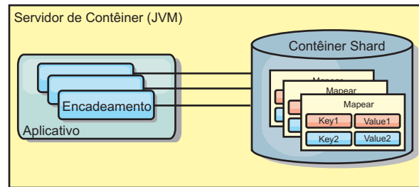
Figura 41. Cenário de Cache em Memória Local
