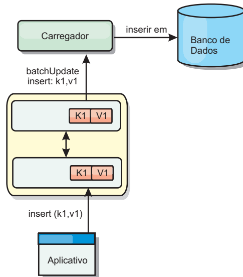
Figura 24. Armazenamento em Cache Write-through
