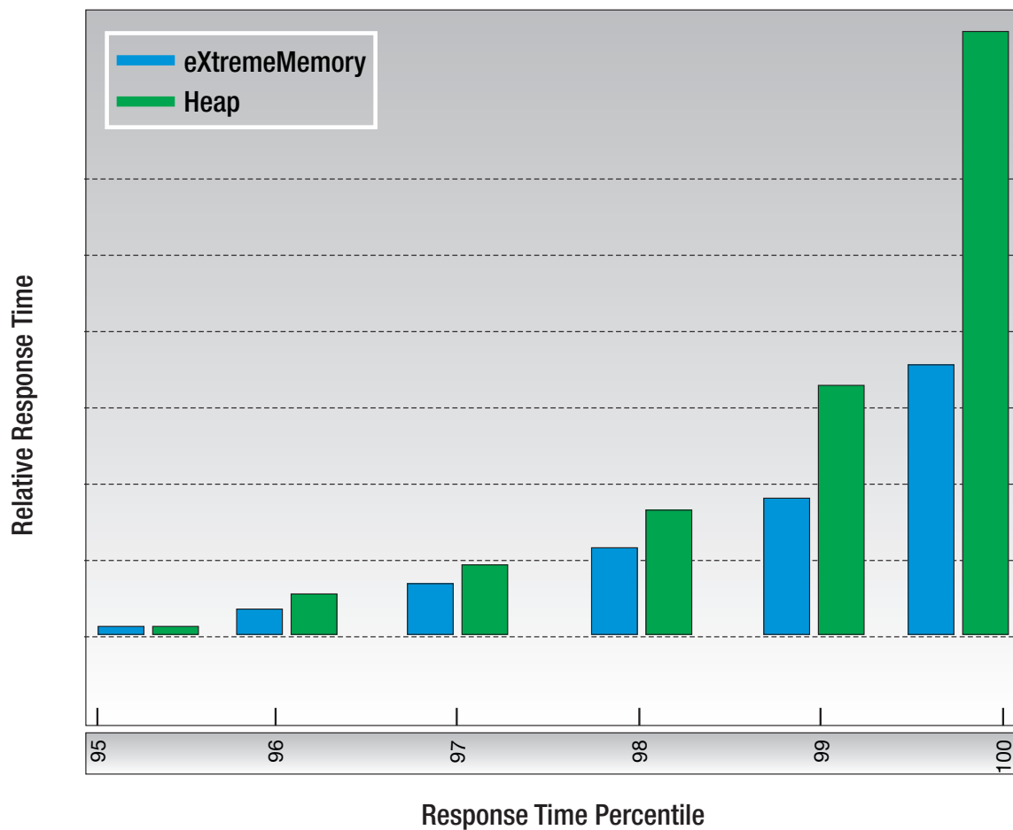
Figura 12. Comparação de eXtremeMemory e Tempos de Resposta de Armazenamento Heap
