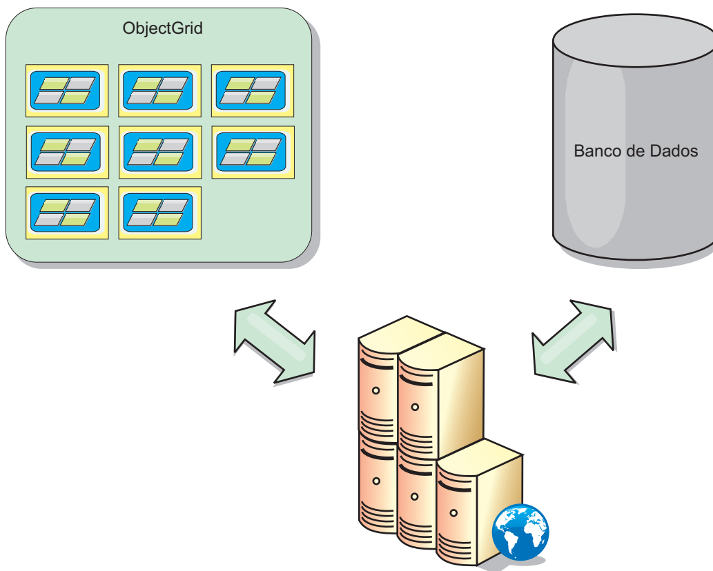
Figura 48. ObjectGrid como um Cache Secundário
