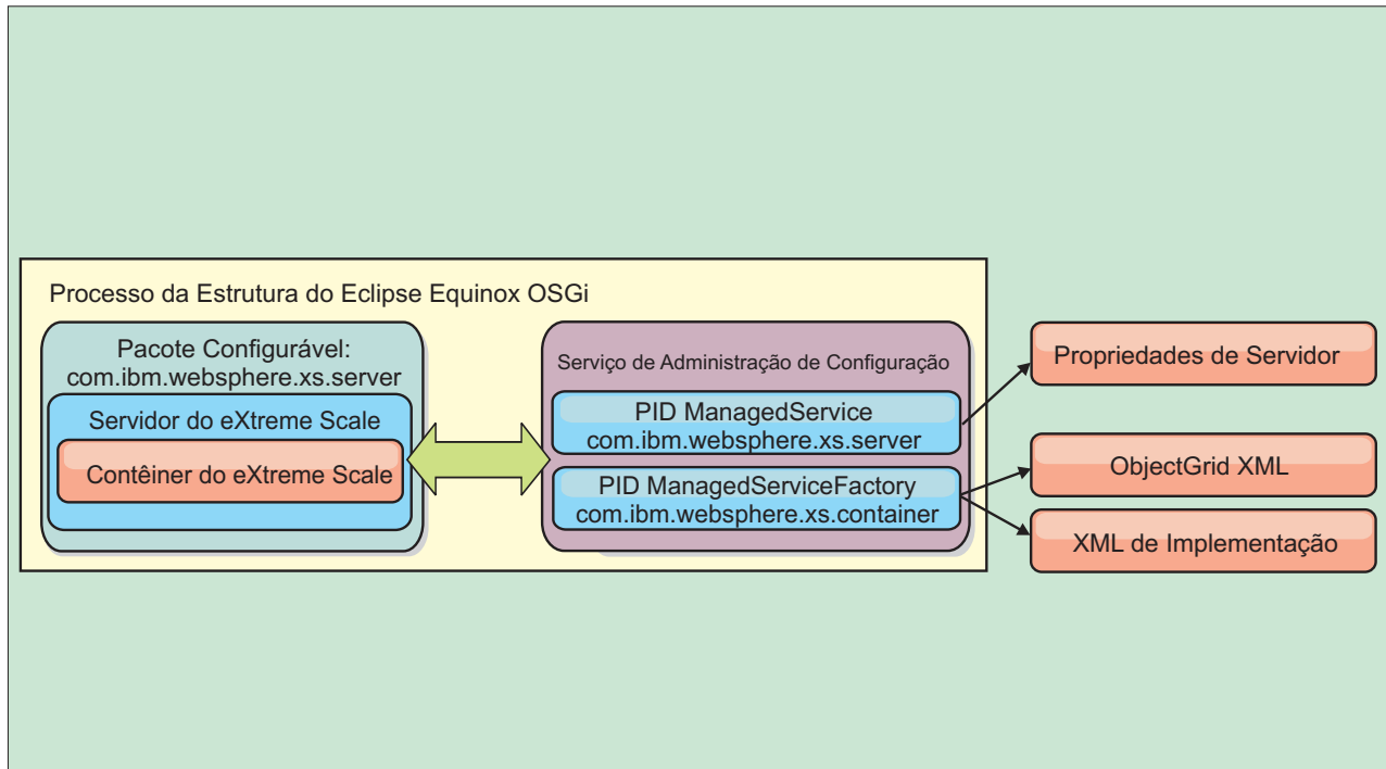
Figura 64. Processo do Eclipse Equinox para Especificar a Configuração e os Metadados Fora de um Pacote Configurável OSGi
