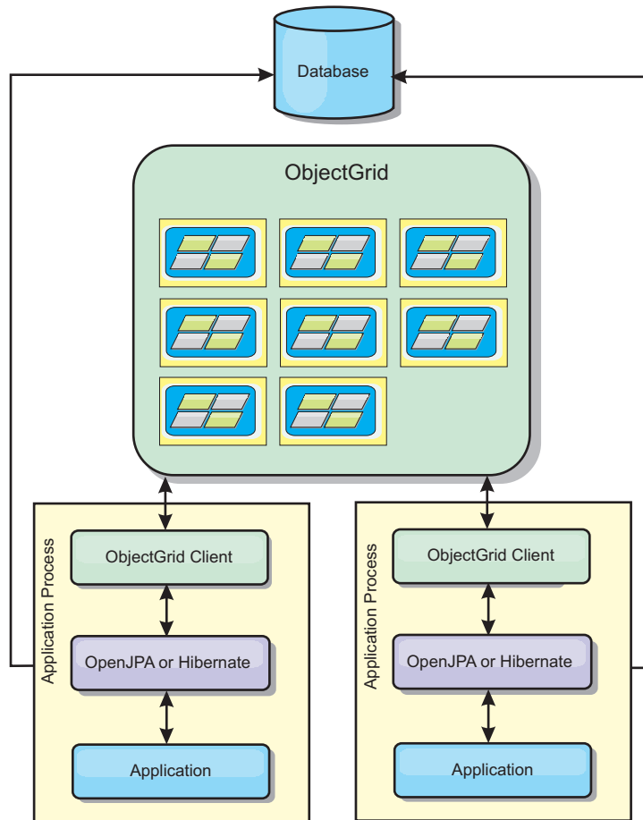
Figura 17. Topologia Remota do JPA
