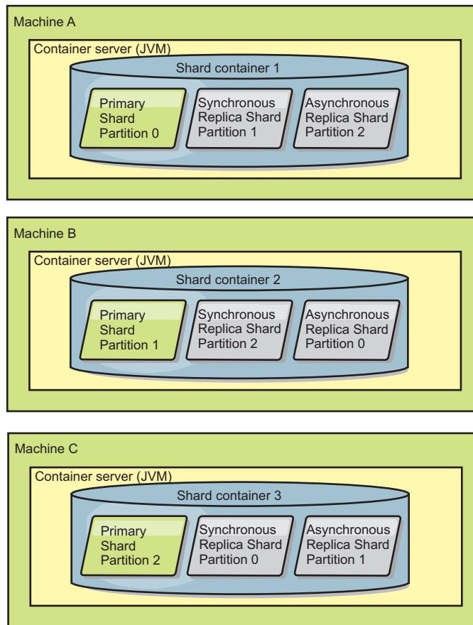
Figura 34. Posicionamento de um Conjunto de Mapas do ObjectGrid com uma Política de Implementação de 3 Partições com um Valor minSyncReplicas de 1, um Valor maxSyncReplicas de 1 e um Valor maxAsyncReplicas de 1
