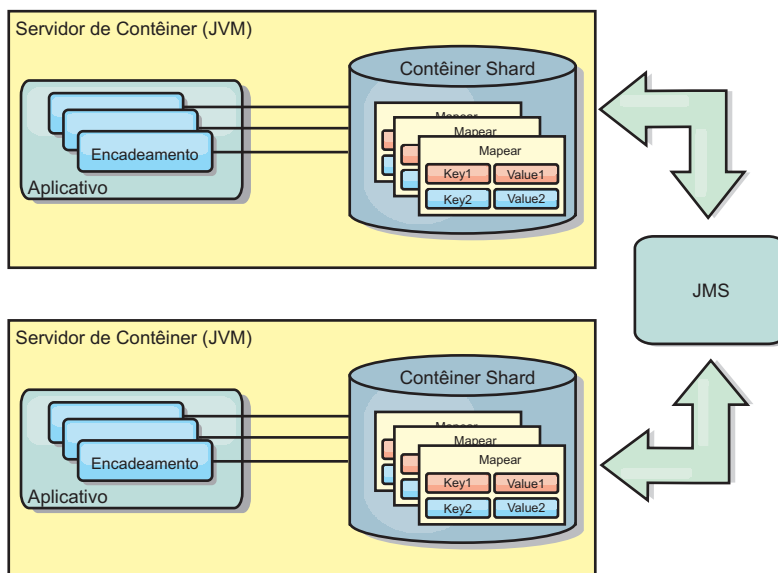
Figura 42. Cache Replicado pelo Peer com Alterações que são Propagadas com JMS
