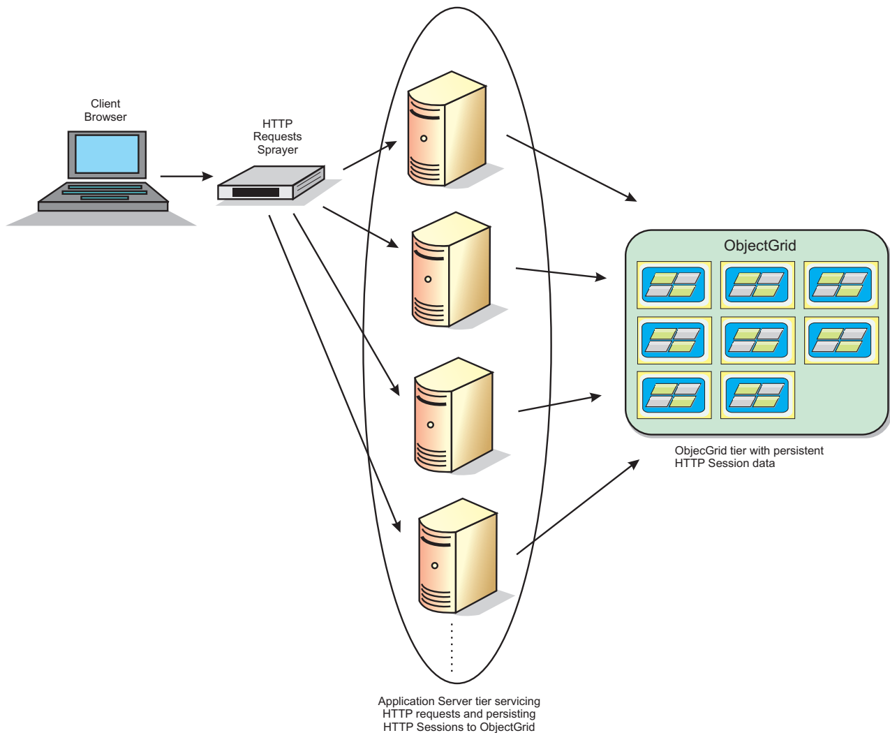
Figura 18. Topologia do Gerenciamento de Sessões HTTP com uma Configuração de Contêiner Remoto
