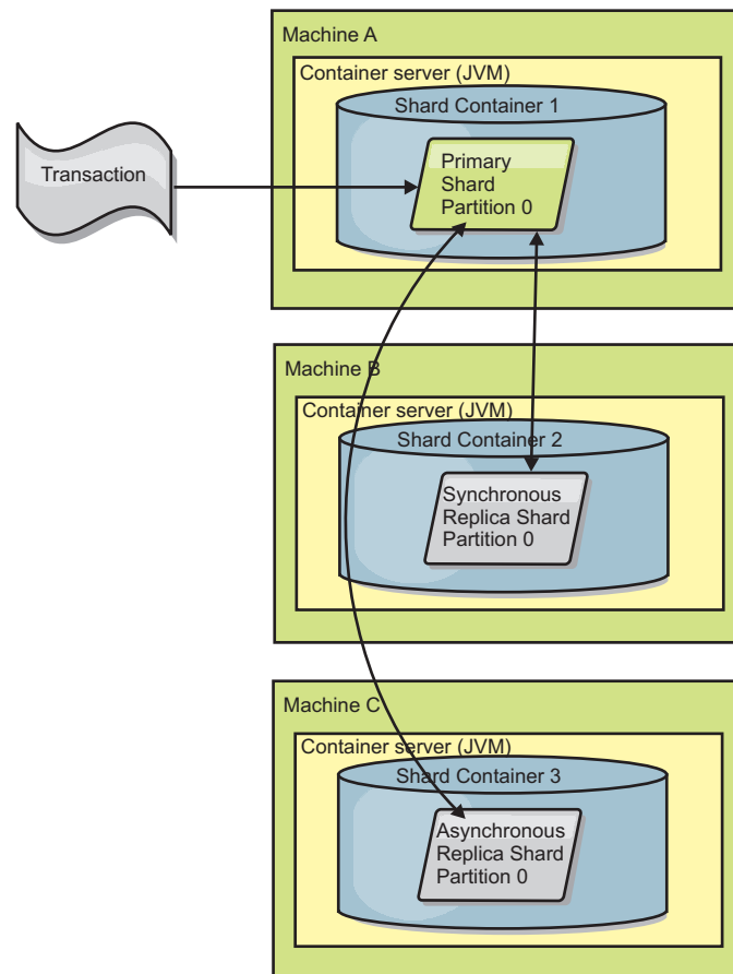
Figura 33. Caminho de Comunicação Entre um Shard Primário e Shards de Réplica
