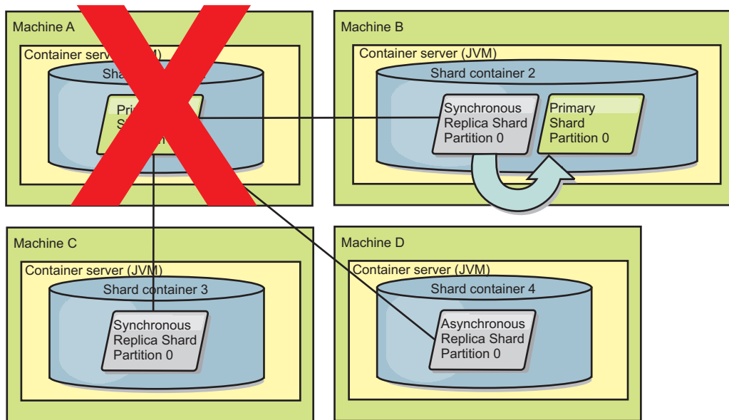
Figura 37. O Shard de Réplica Síncrona no Contêiner 2 do ObjectGrid se Torna o Shard Primário
