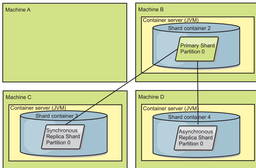
Figura 38. A máquina B contém o shard primário. Dependendo de como o modo de reparo automático é configurado e da disponibilidade dos contêineres, um novo shard de réplica síncrona pode ou não ser posicionado em uma máquina.
