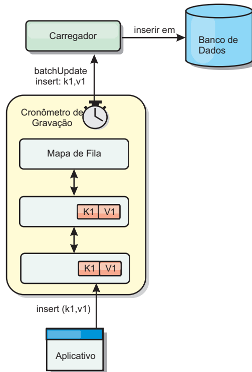
Figura 53. Armazenamento em Cache Write-behind
