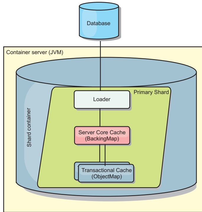
Figura 28. Plug-in do Utilitário de Carga
