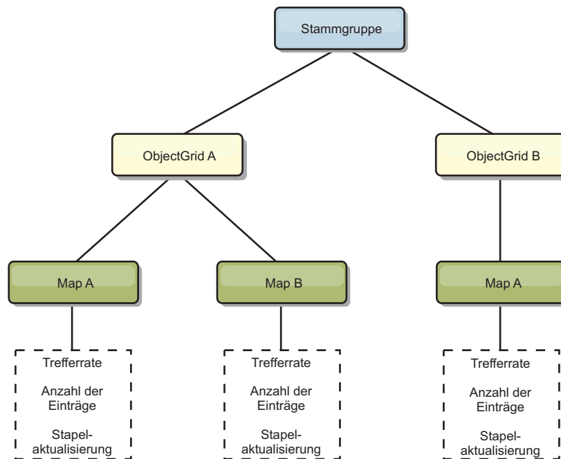
Abbildung 64. Beispielstruktur für das Modul "mapModule"
