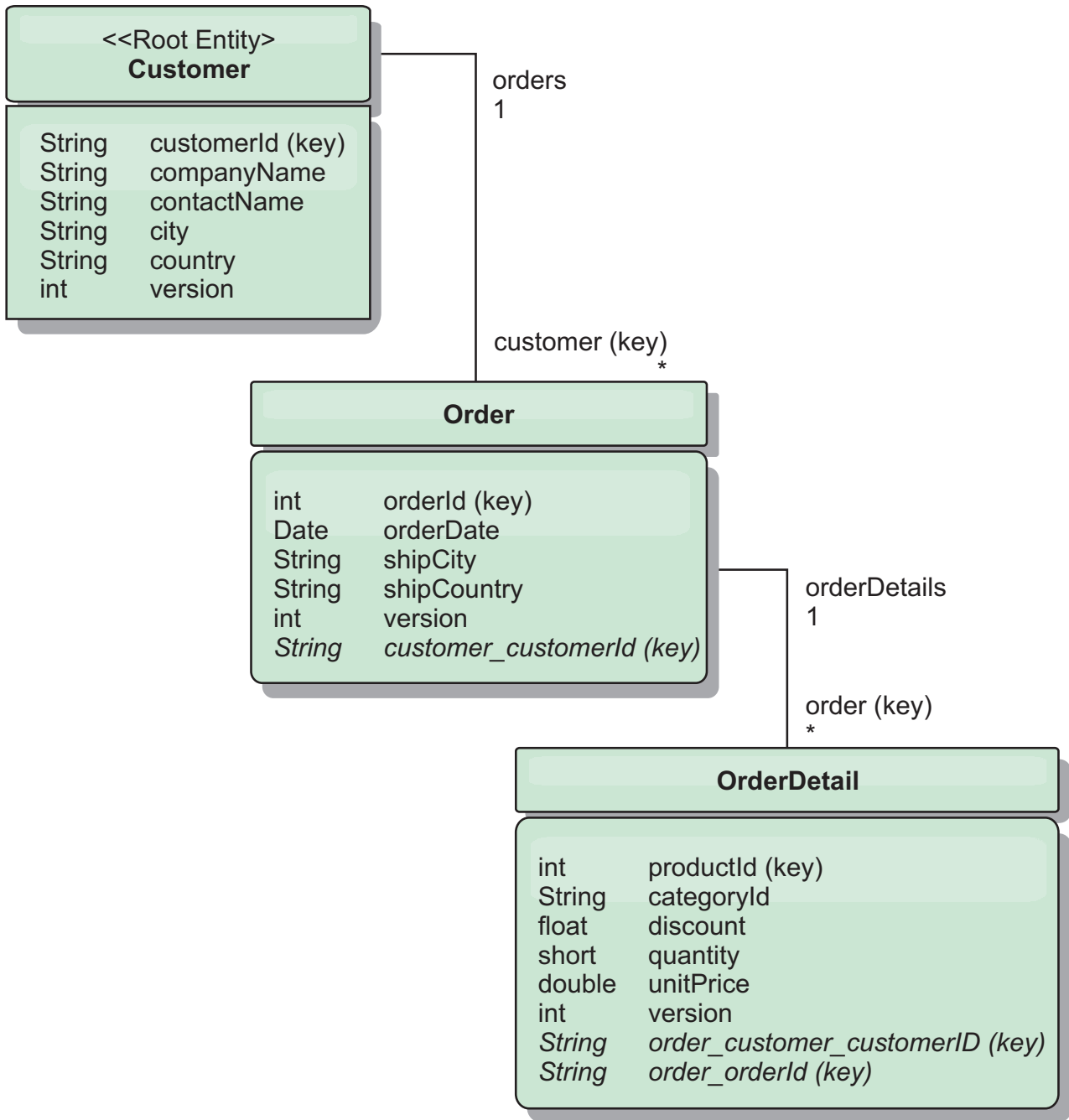
Abbildung 49. Entitätsschemadiagramm "Customer und Order"
