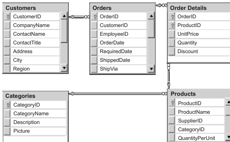
Abbildung 48. Schemadiagramm zum Beispiel "Microsoft SQL Server Northwind"
