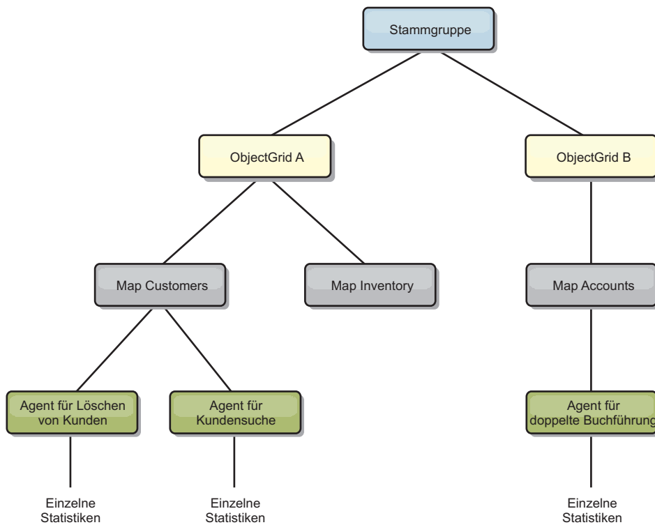
Abbildung 68. Beispielstruktur für das Modul "agentManagerModule"
