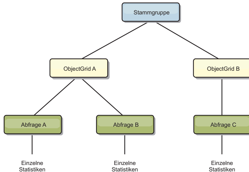
Abbildung 70. Beispielstruktur für das Modul "queryModule"
