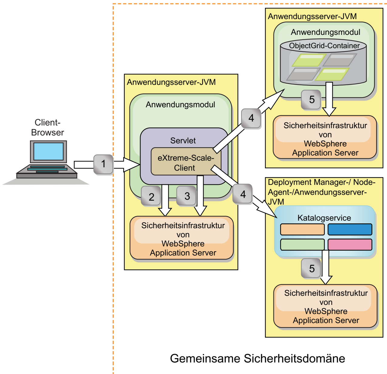
Abbildung 71. Authentifizierungsablauf für Server in derselben Sicherheitsdomäne
