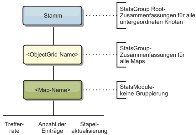
Abbildung 63. Struktur des Moduls "mapModule"
