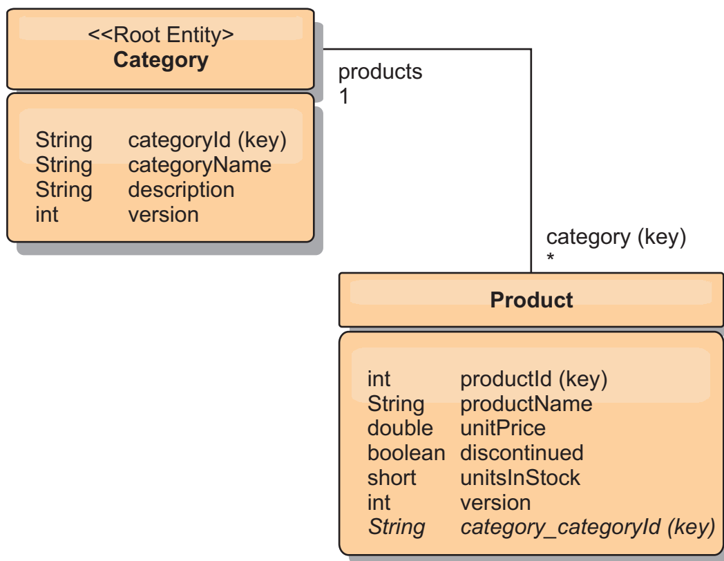
Abbildung 50. Entitätsschemadiagramm "Category und Product"
