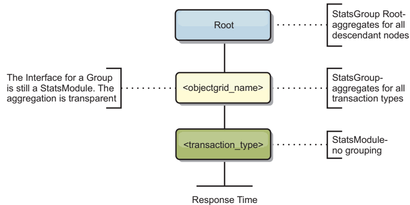
Abbildung 61. Struktur des Moduls "ObjectGridModule"
