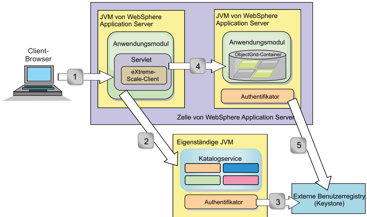
Abbildung 25. Authentifizierungsablauf
