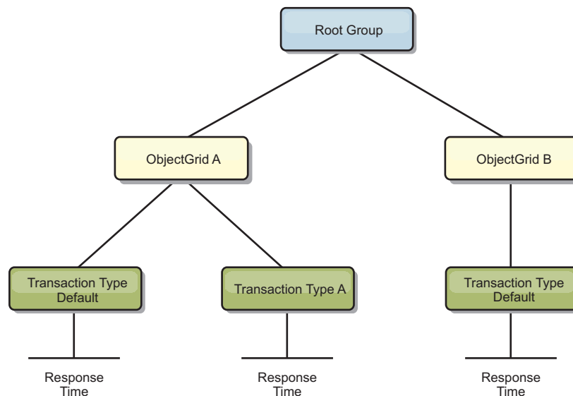
Abbildung 62. Beispielstruktur für das Modul "ObjectGridModule"
