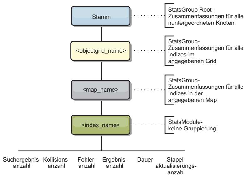
Abbildung 65. Struktur des Moduls "hashIndexModule"
