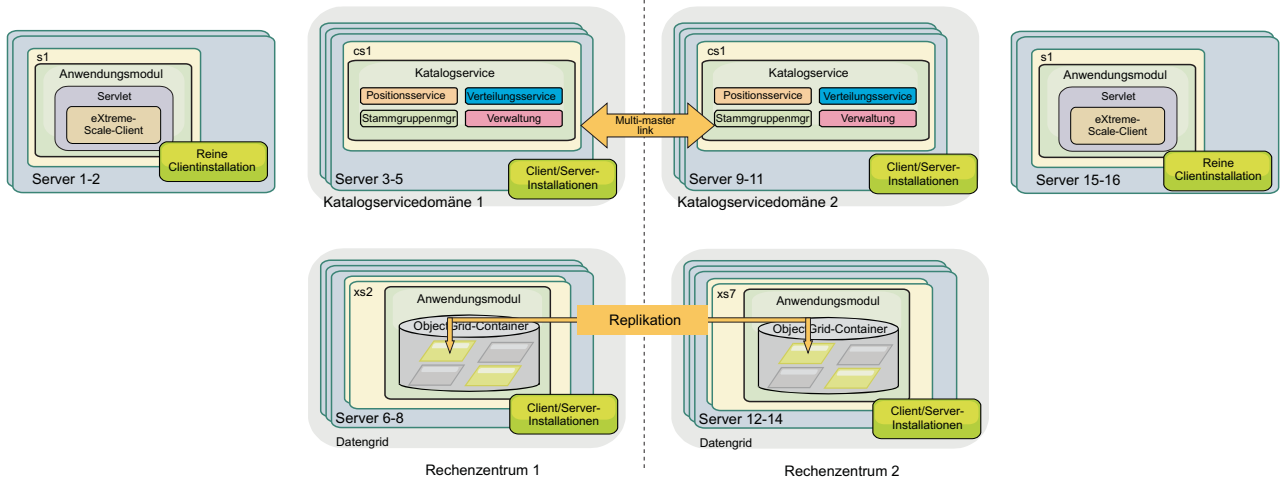
Abbildung 27. Eigenständige Topologie mit zwei Rechenzentren
