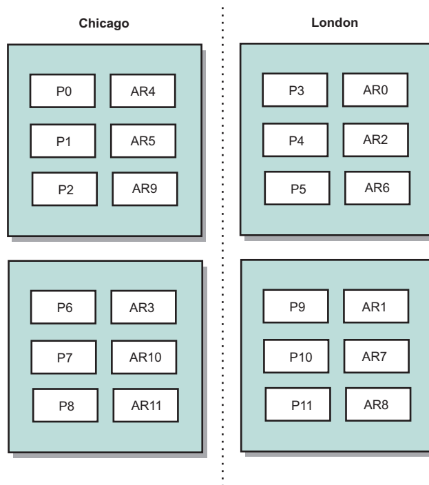
Abbildung 33. Primäre Shards und Replikate in Zonen
