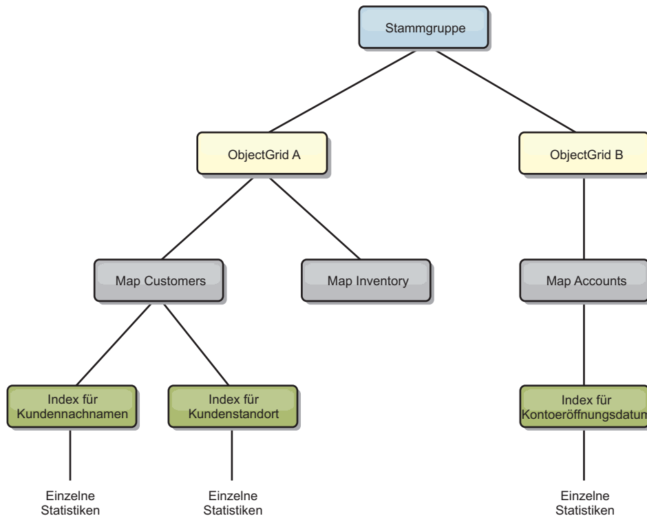
Abbildung 66. Beispielstruktur für das Modul "hashIndexModule"
