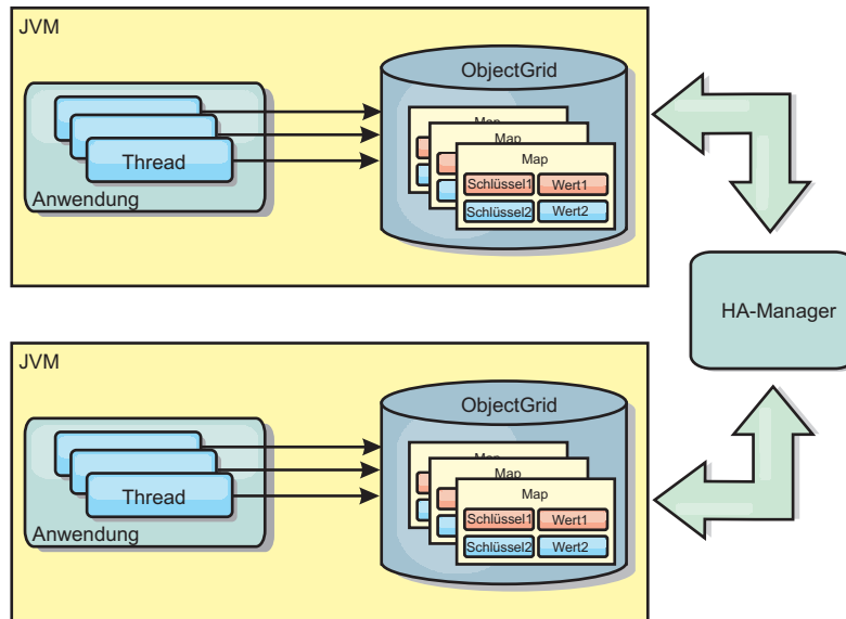
Abbildung 5. Auf Peers replizierter Cache mit Änderungen, die über den High Availability Manager weitergegeben werden
