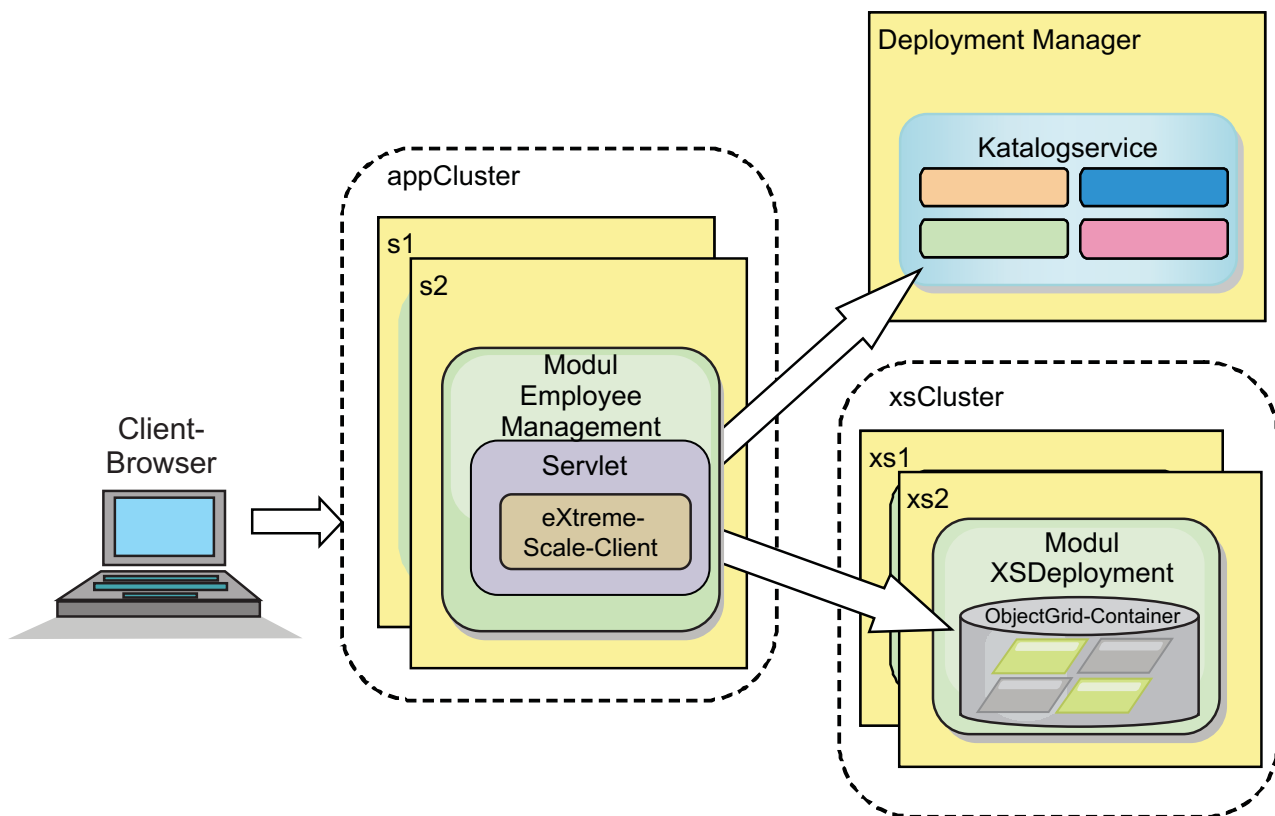
Abbildung 23. Lernprogrammtopologie
