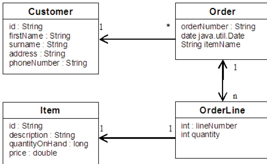
Abbildung 21. Bestellungsschema . Ein Bestellungsschema (Order) hat eine Eins-zu-eins-Beziehung mit einem Kunden (Customer) und eine Eins-zu-viele-Beziehung mit Bestellpositionen (OrderLine). Die Map "OrderLine" hat eine Eins-zu-eins-Beziehung mit einem Artikel (Item) und enthält die bestellte Menge.
