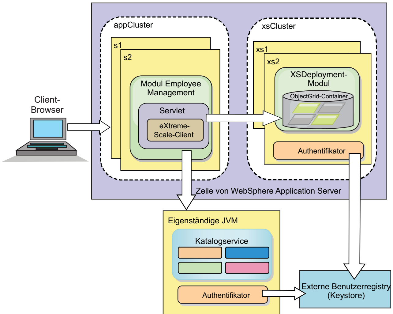
Abbildung 24. Lernprogrammtopologie
