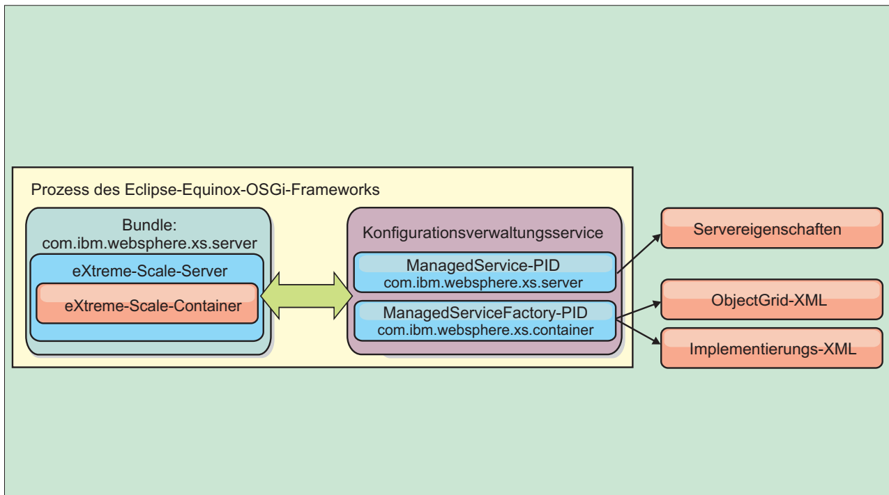
Abbildung 55. Eclipse-Equinox-Prozess für die Angabe von Konfigurations- und Metadaten außerhalb eines OSGi-Bundles
