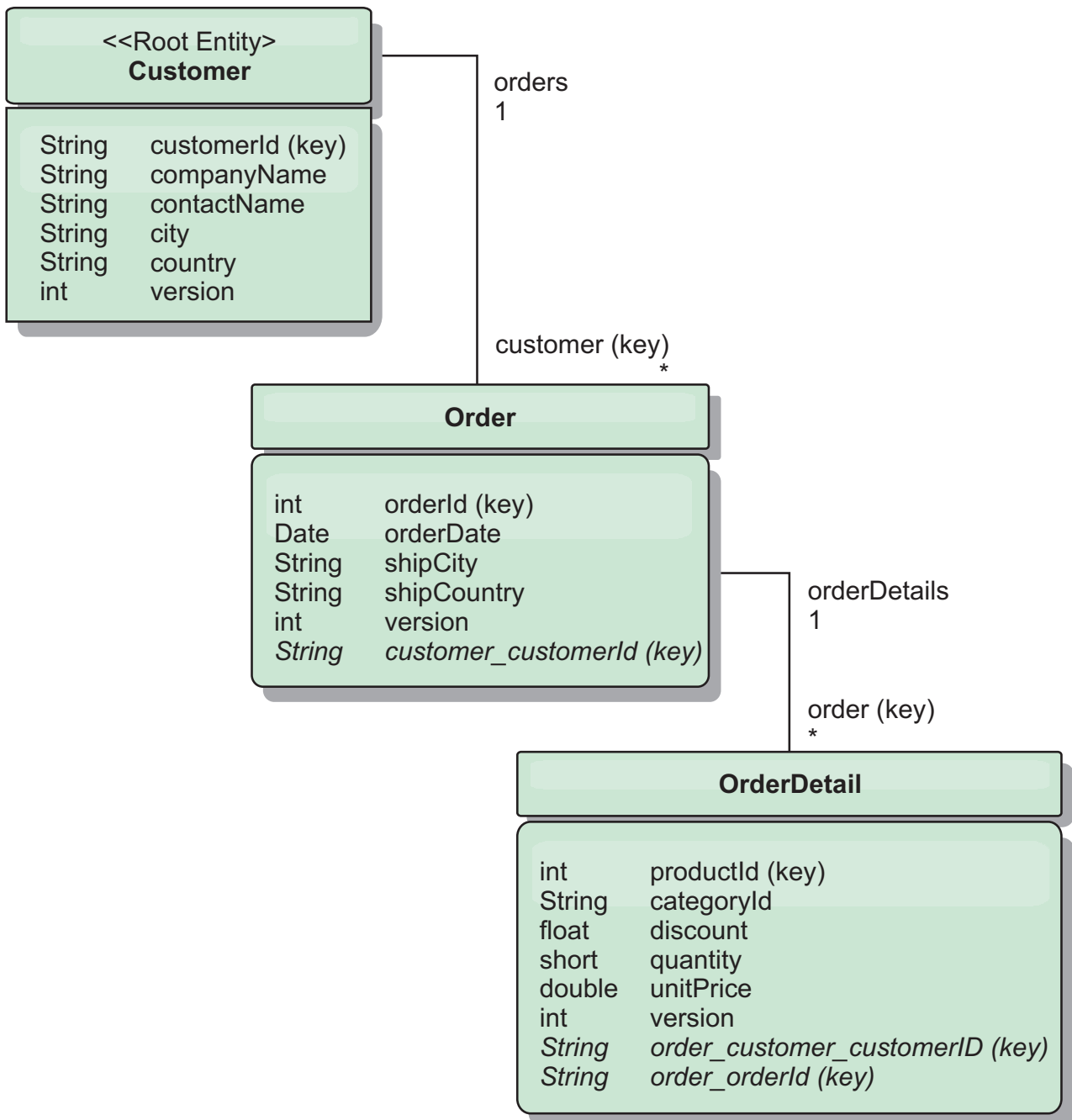
Abbildung 51. Entitätsschemadiagramm "Customer und Order"
