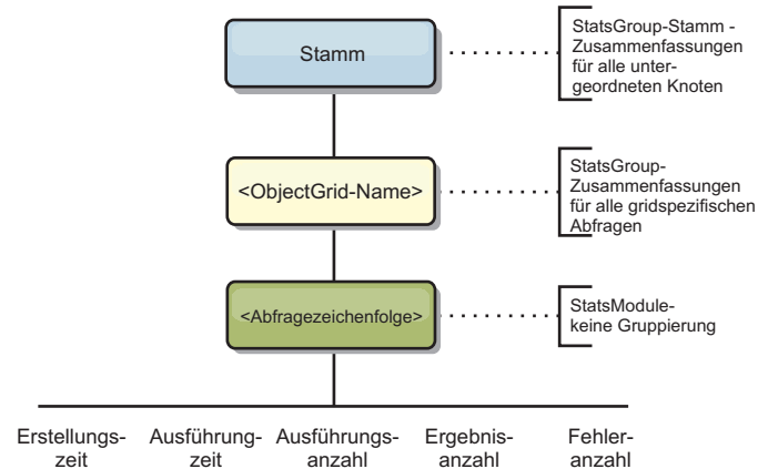
Abbildung 69. Struktur des Moduls "queryModule"
