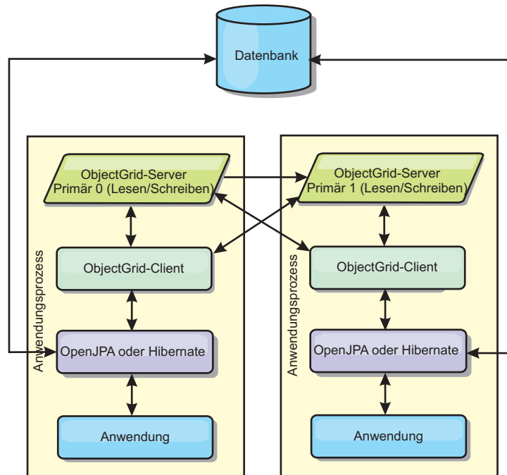
Abbildung 45. Integrierte, partitionierte JPA-Topologie
