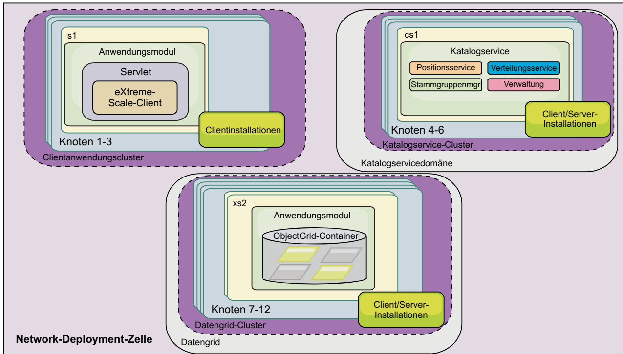
Abbildung 28. Beispiel für die Topologie mit WebSphere Application Server
