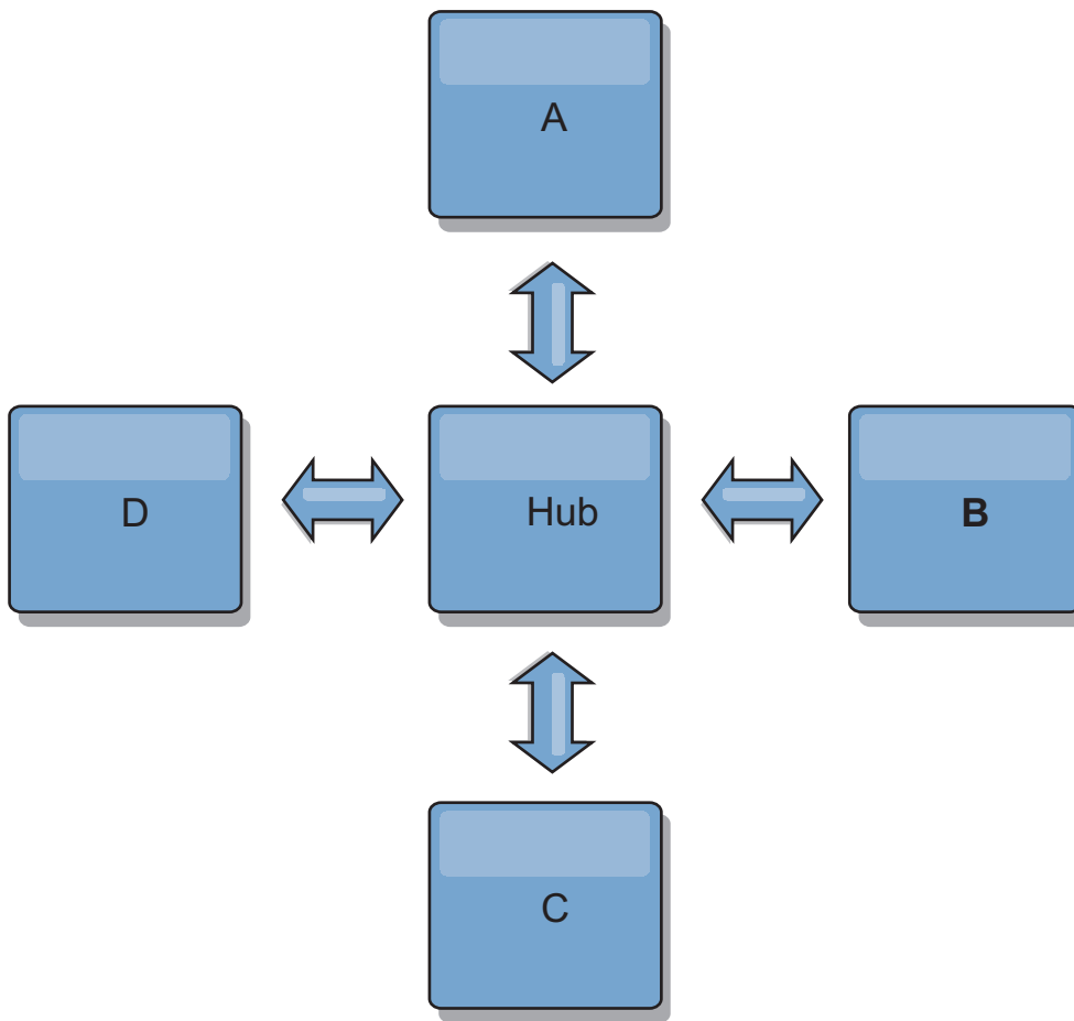
Abbildung 36. Beispiel: Hub- und Peripherietopologie
