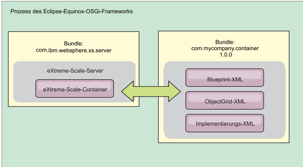
Abbildung 54. Eclipse-Equinox-Prozess für den Einschluss aller Konfigurations- und Metadaten in ein OSGi-Bundle
