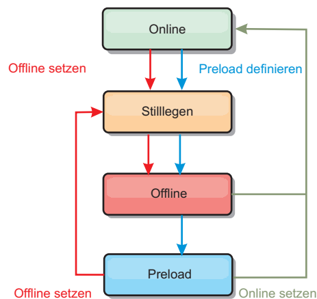
Abbildung 53. Verfügbarkeitsstatus einer ObjectGrid-Instanz
