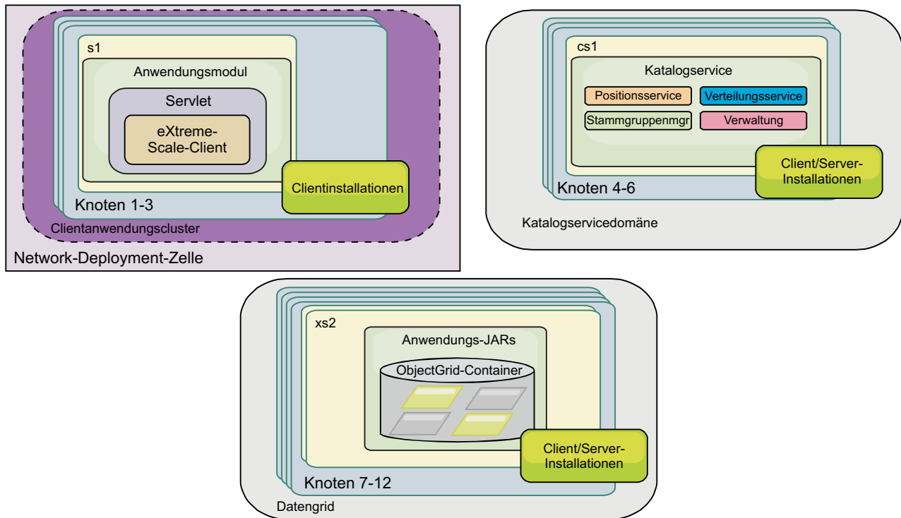
Abbildung 29. Beispiel für eine heterogene Topologie
