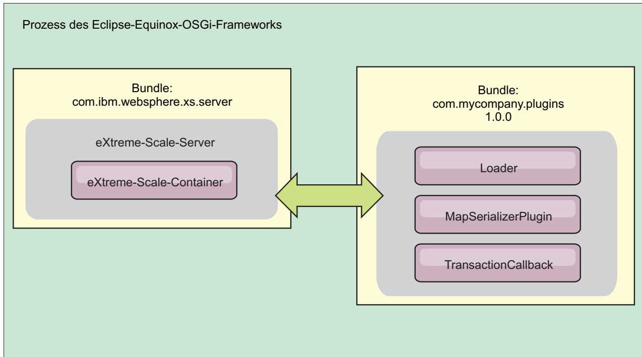
Abbildung 52. Eclipse-Equinox-Prozess für die Installation und das Starten von OSGi-Bundles mit Plug-ins von eXtreme Scale
