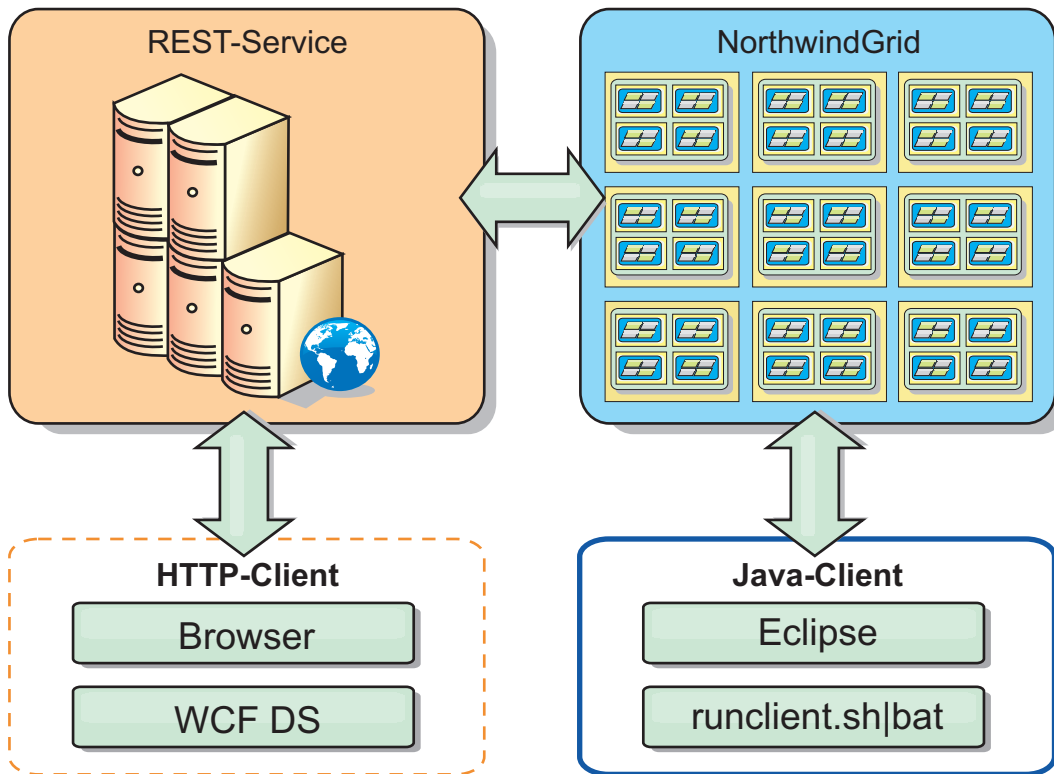
Abbildung 47. Beispieltopologie zur Einführung. HTTP-Clients, die den REST-Datenservice verwenden, und Java-Clients können auf dasselbe Datengrid zugreifen.
