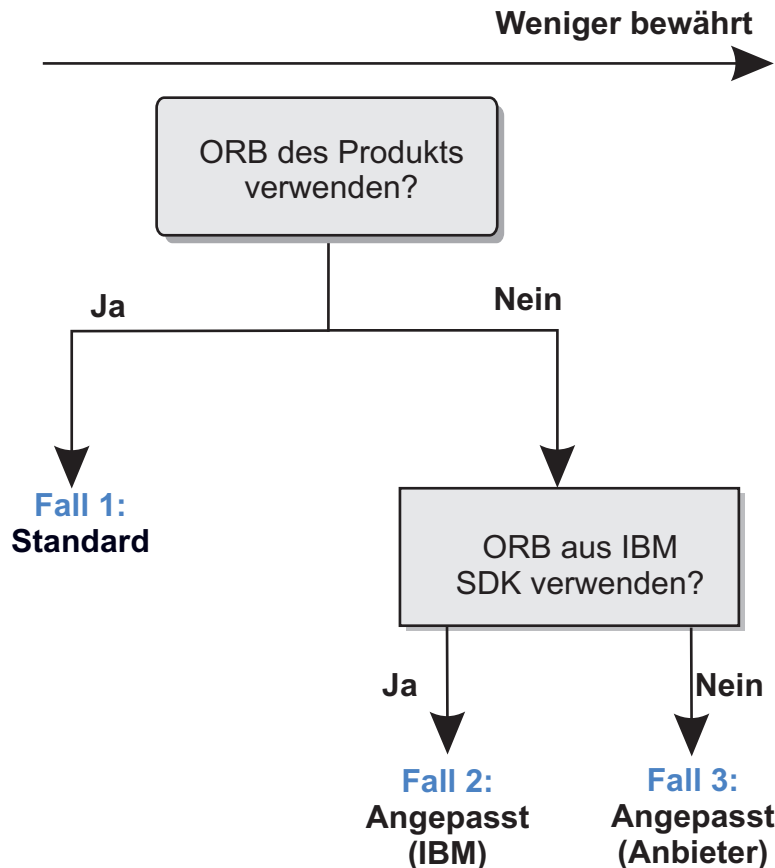
Abbildung 38. ORB auswählen
