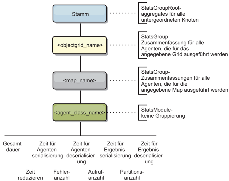
Abbildung 67. Struktur des Moduls "agentManagerModule"
