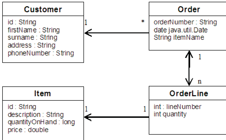
Abbildung 22. Schema für die Entität "Order". Eine Entität "Order" (Auftrag) hat eine Referenz auf einen Kunden (Customer) und keiner oder mehreren Auftragspositionen (OrderLine). Jede Entität "OrderLine" hat eine Referenz auf einen einzelnen Artikel (Item) und enthält die bestellte Menge.
