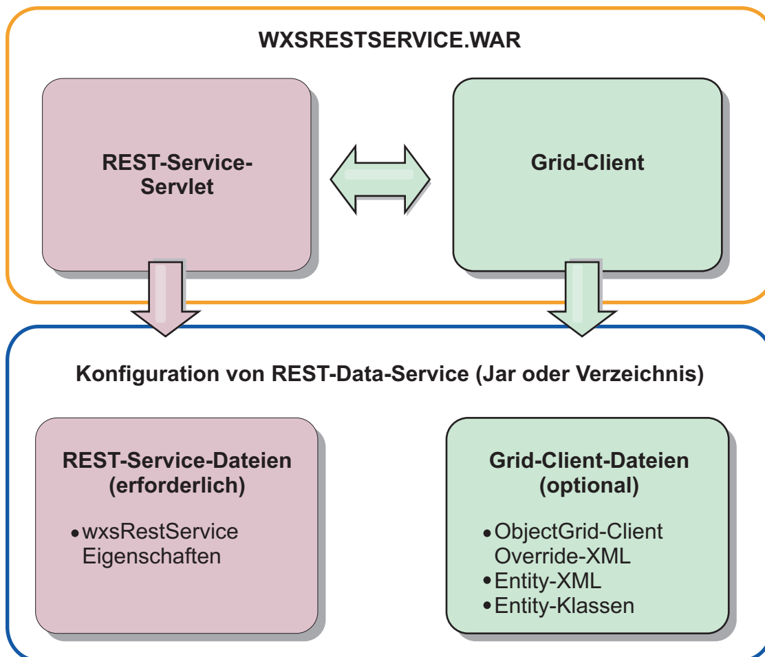
Abbildung 30. Dateien des REST-Datenservice von WebSphere eXtreme Scale
