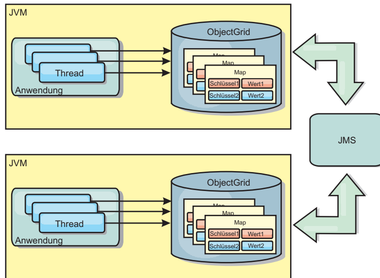
Abbildung 4. Auf Peers replizierter Cache mit Änderungen, die über JMS weitergegeben werden
